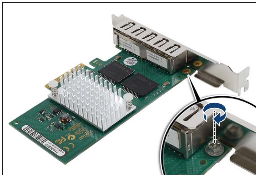
図 104: ネットワークアダプタ D2745 - スロットブラケットの取り付け (B)
