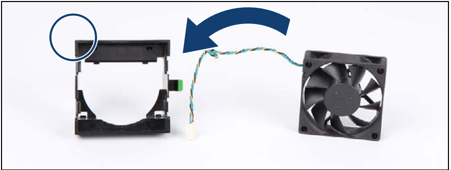
図 64: 3.5 インチファンホルダーへのファンの取り付け
