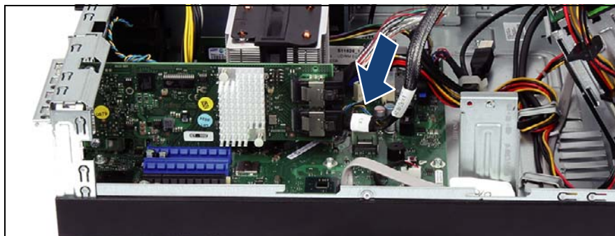
図 161: RAID コントローラへの SATA ケーブルの接続
