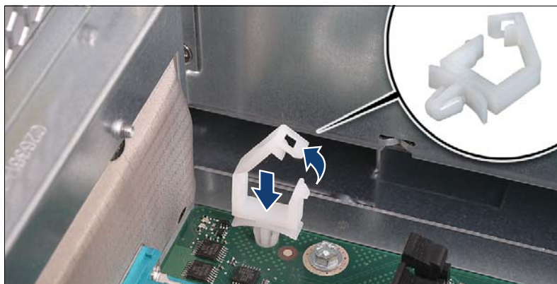
図 197: 電源ケーブルクランプの取り付け
