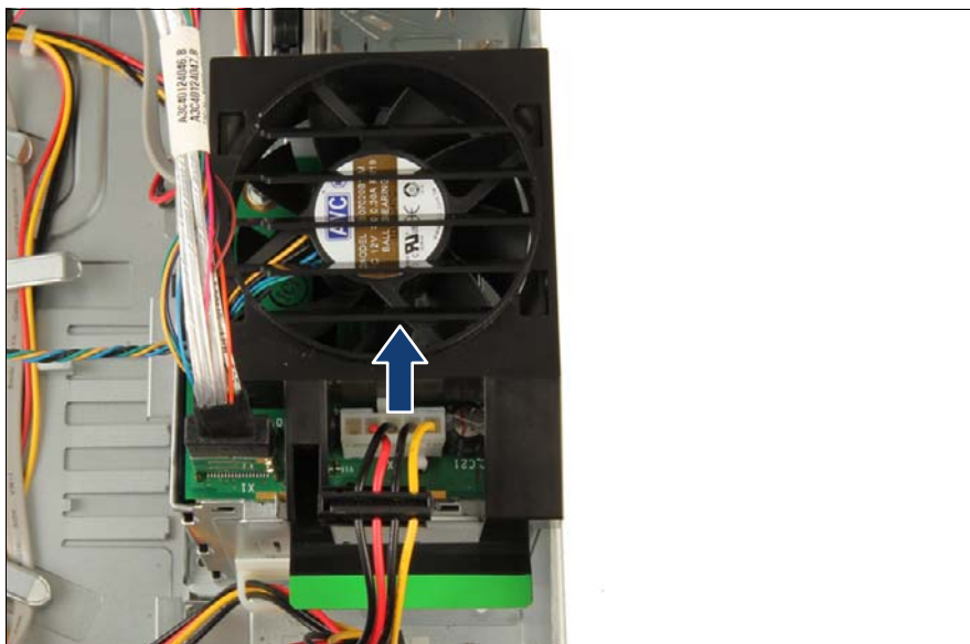
図 75: 電源ケーブルの HDD ファンモジュールからの取り外し
