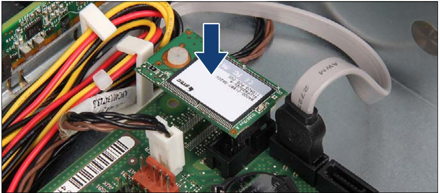
図 177: UFM の取り付け
