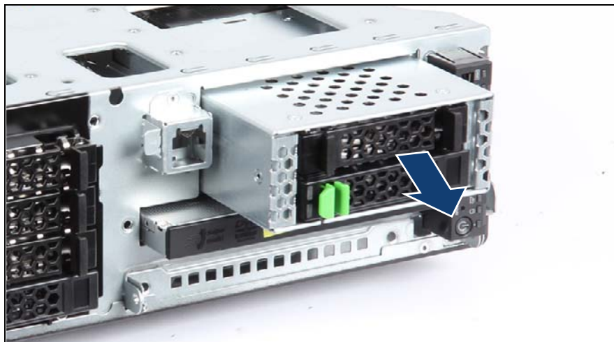
図 166: ベイ追加オプションの取り外し
