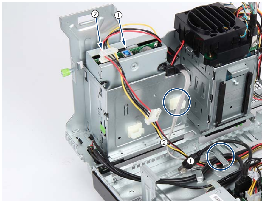
図 152: バックアップドライブからのケーブルの取り外し
