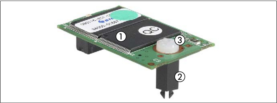
図 175: UFM キット
