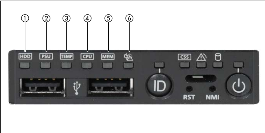
図 6: フロントパネルのローカル診断表示ランプ
