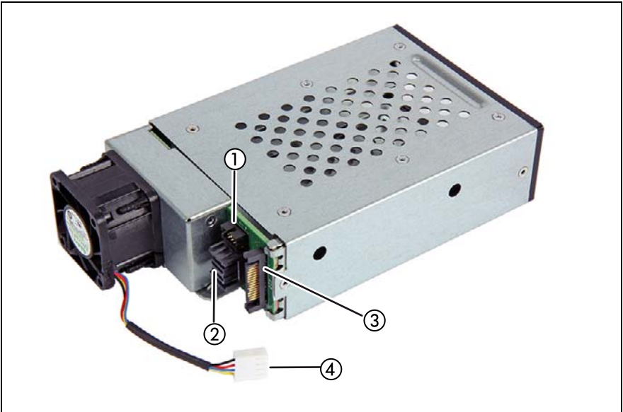
図 159: ベイ追加オプションの背面コネクタ
