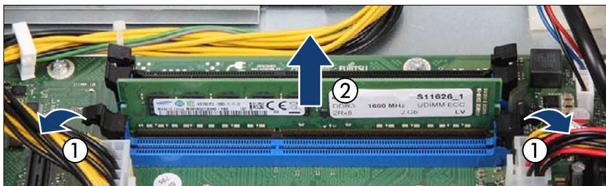
図 119: メモリモジュールの取り外し
