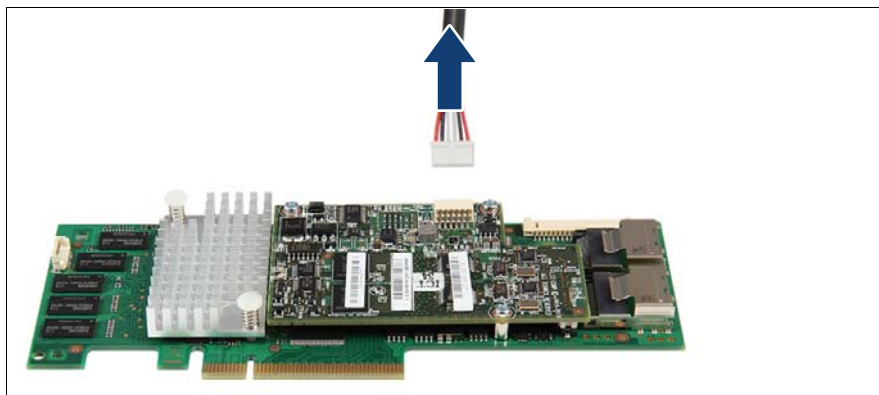
図 94: TFM からの FBU アダプタケーブルの取り外し
