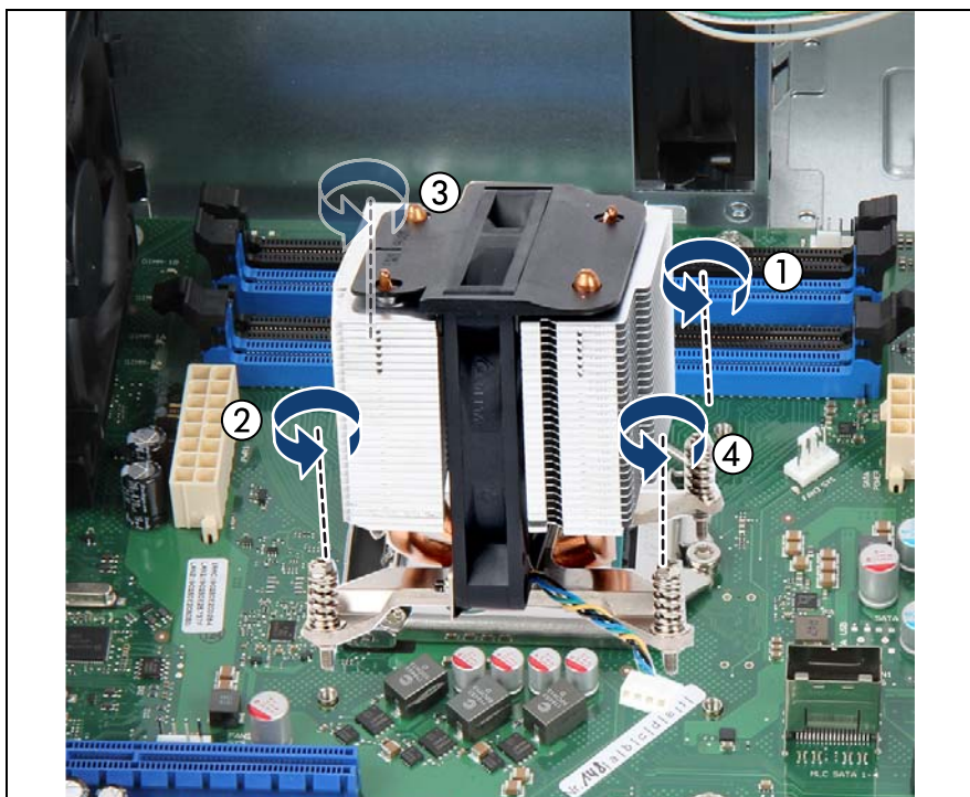
図 121: プロセッサヒートシンクの取り外し
