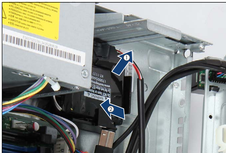
図 96: FBU ホルダーの取り付け
