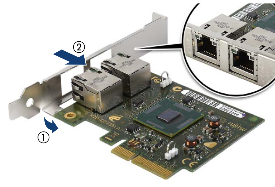
図 100: ネットワークアダプタ D2735 - スロットブラケットの取り付け (A)
