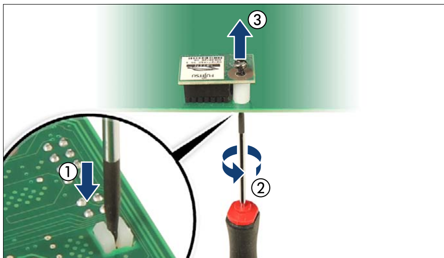
図 189: TPM 用ネジの取り外し
