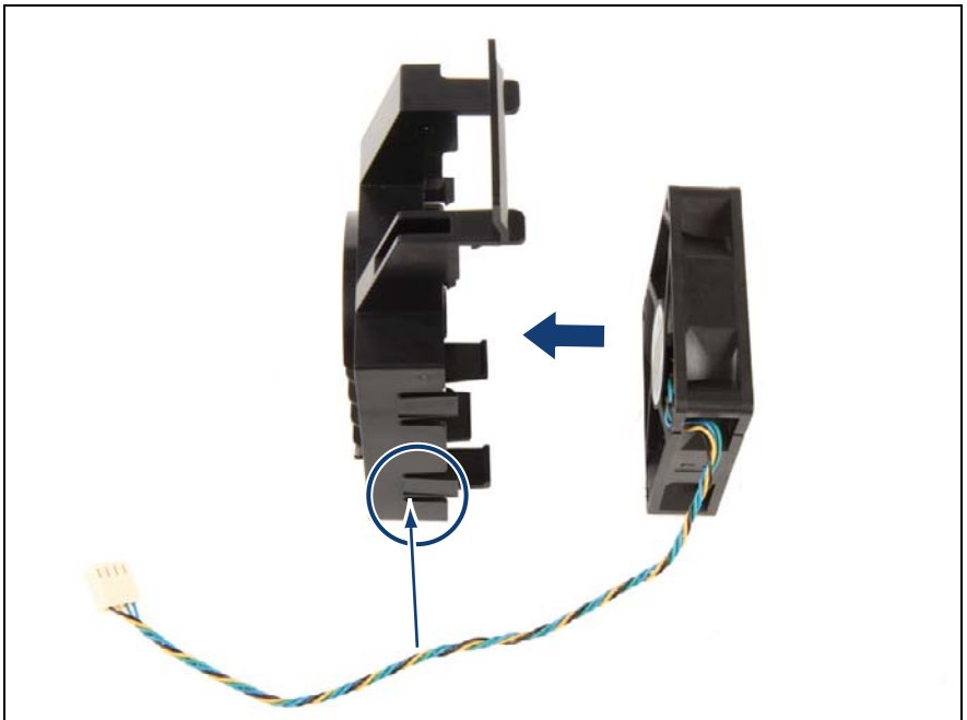
図 77: 3.5 インチファンホルダーへのファンの取り付け
