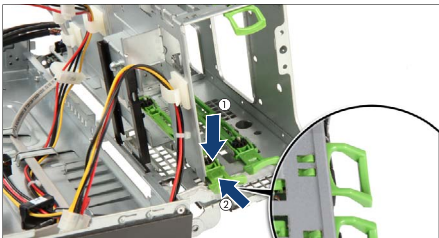
図 50: イージークリックレールの挿入
