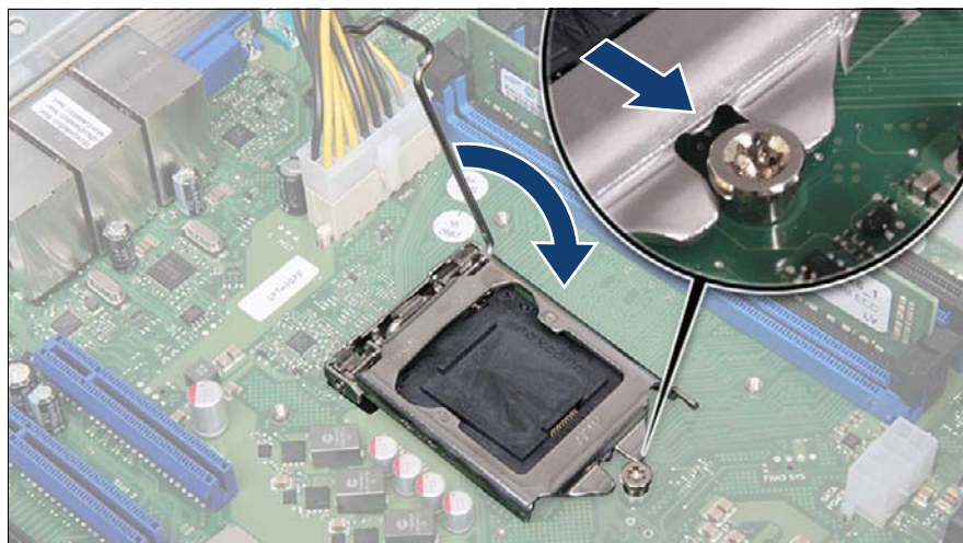
図 201: ソケット保護カバーの取り付け（故障しているシステムボード）（B）
