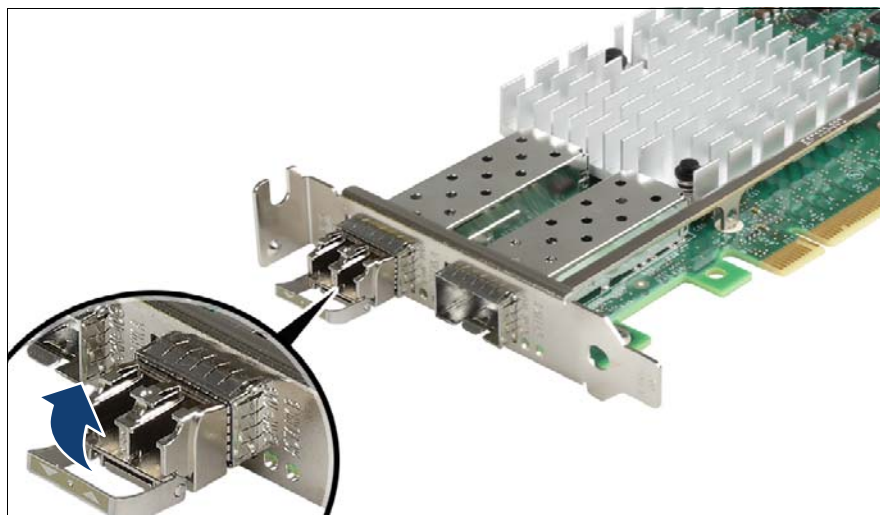
図 112: ロッキングハンドルのラッチ留め
