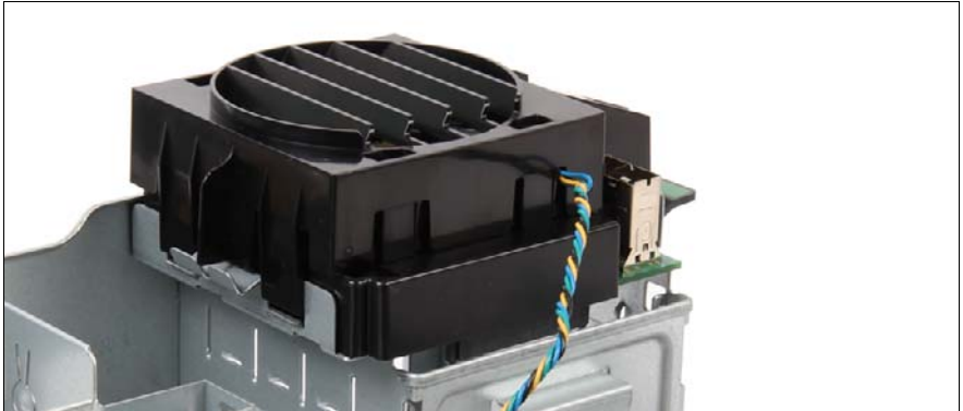
図 73: 追加の送風ダクトの位置
