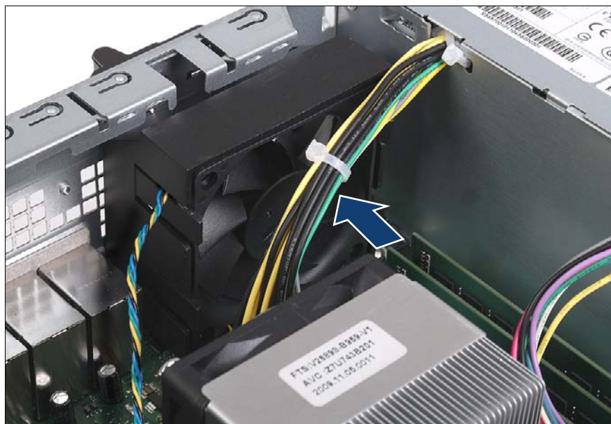
図 65: システムファンモジュールの取り付け (A)
