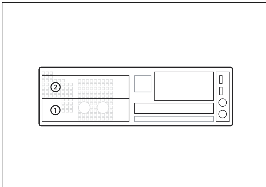
図 43: 3.5 インチ HDD の取り付け順序
