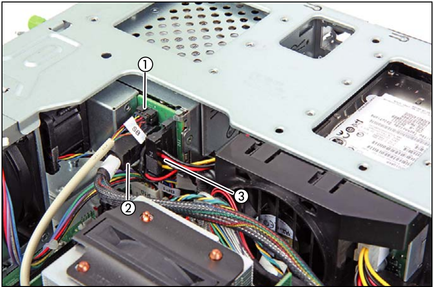
図 164: すべてのケーブルを ベイ追加オプションからの取り外し
