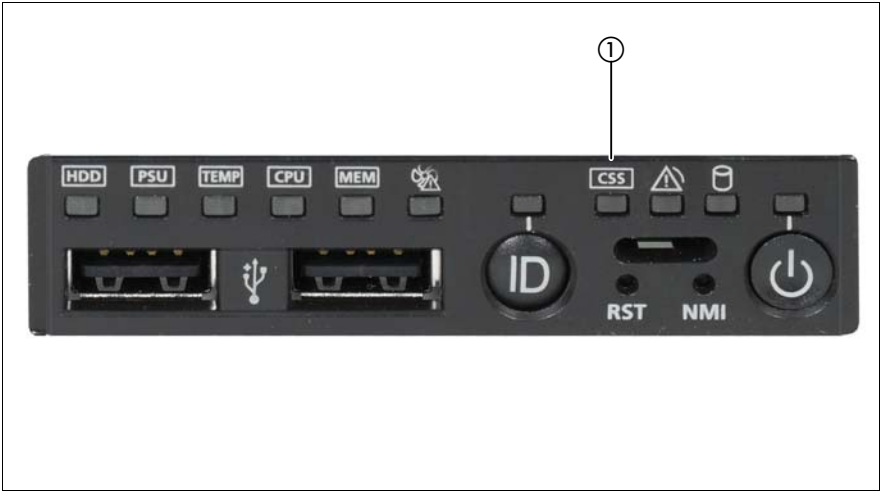
図 5: フロントパネルの CSS 表示ランプ
