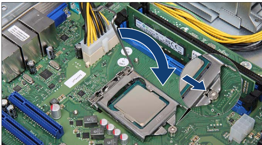
図 126: ロードプレートを閉じる (B)
