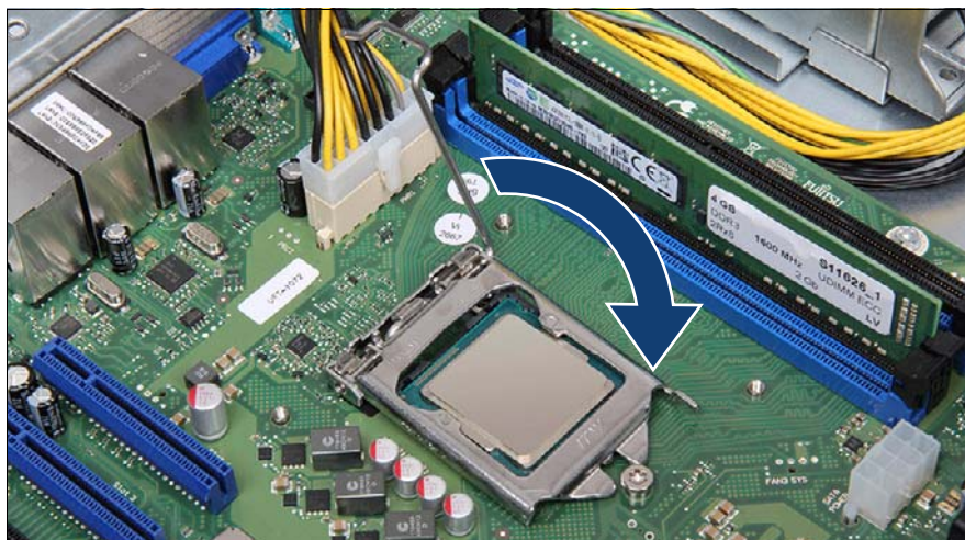
図 125: ロードプレートを閉じる (A)
