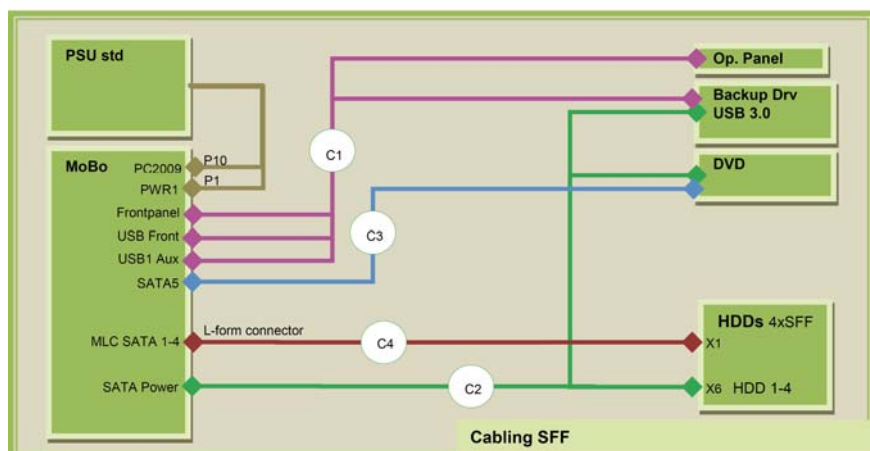
図 204: ケーブル配線 - 4x 2.5 インチ HDD モデル (SFF)
