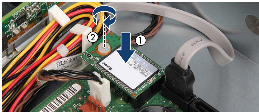
図 181: UFM の取り付け
