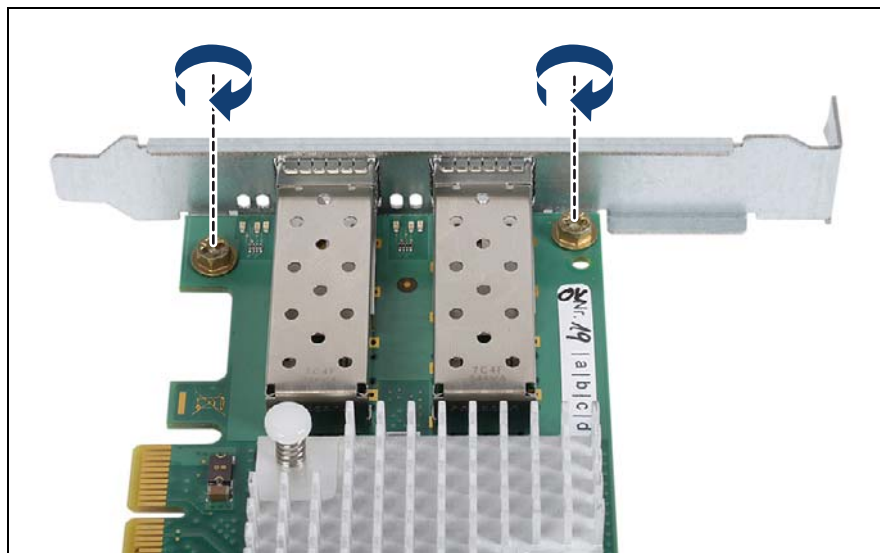
図 107: ネットワークアダプタ D2755 - スロットブラケットの取り付け (B)
