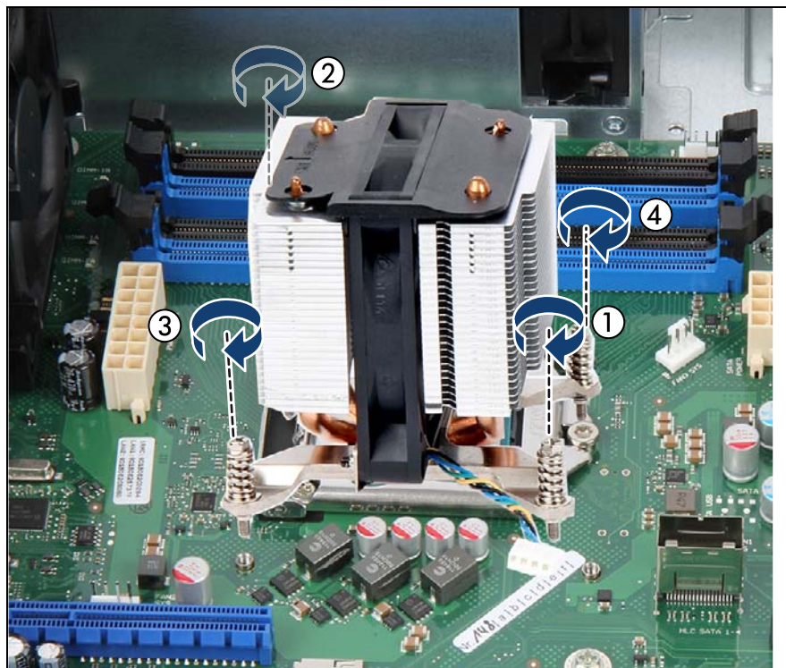
図 131: ヒートシンクを取り付ける (B)
