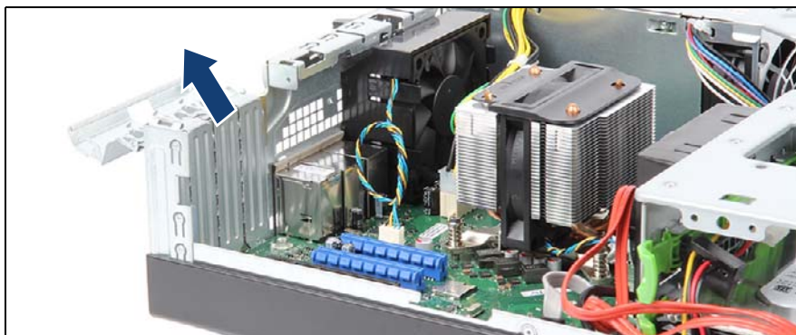
図 81: PCI スロットブラケットの取り外し
