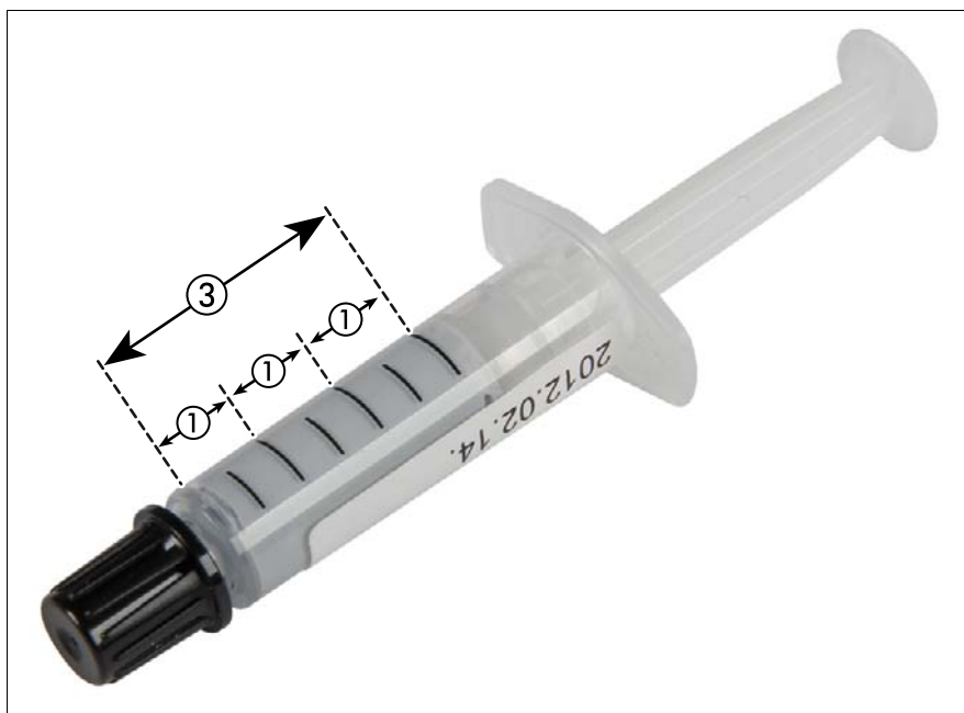
図 128: サーマルペーストの注射器
