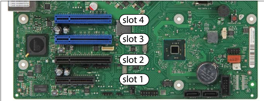
図 79: PCI スロットの概観
