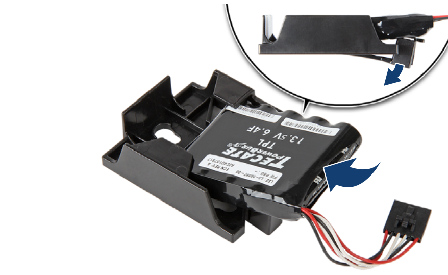
図 88: FBU ホルダーへの FBU の取り付け (A)
