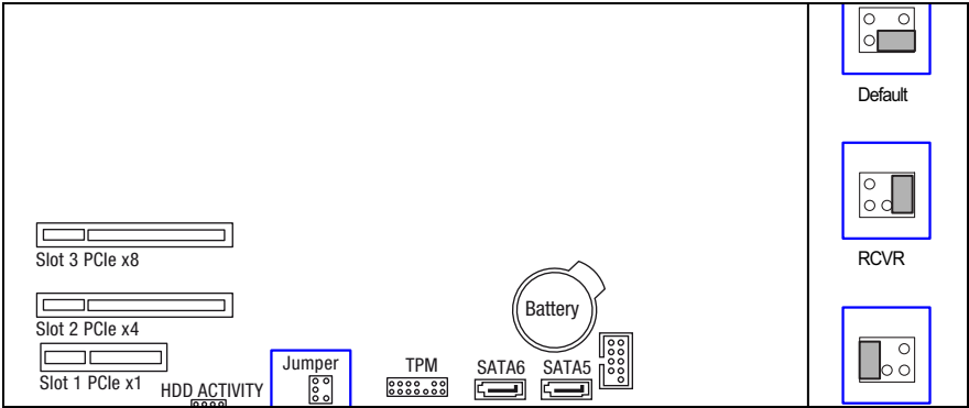
図 210: ジャンパ
