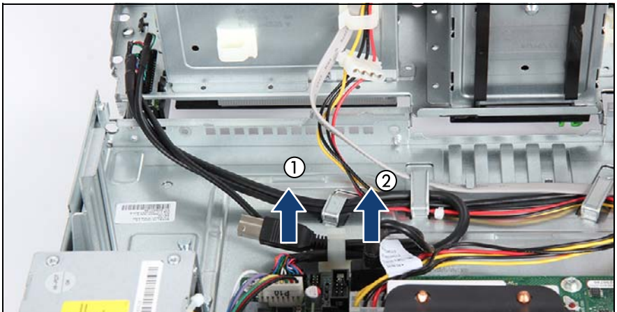
図 168: フロントパネルケーブルの取り外し
