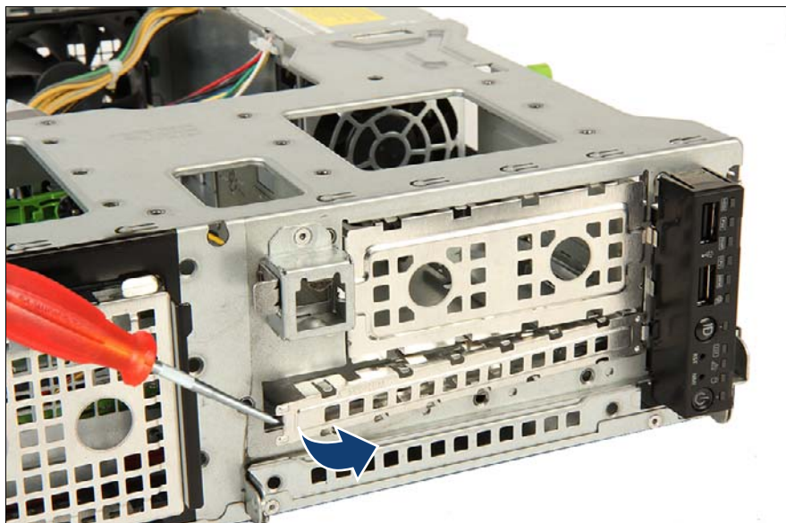
図 134: ODD フィラーカバーの取り外し
