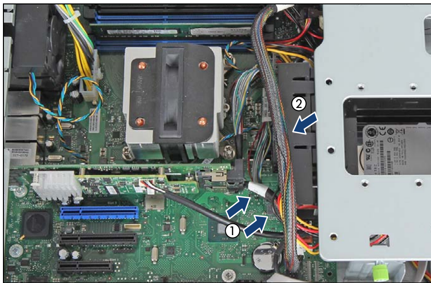
図 162: RAID コントローラからの SATA ケーブルの配線
