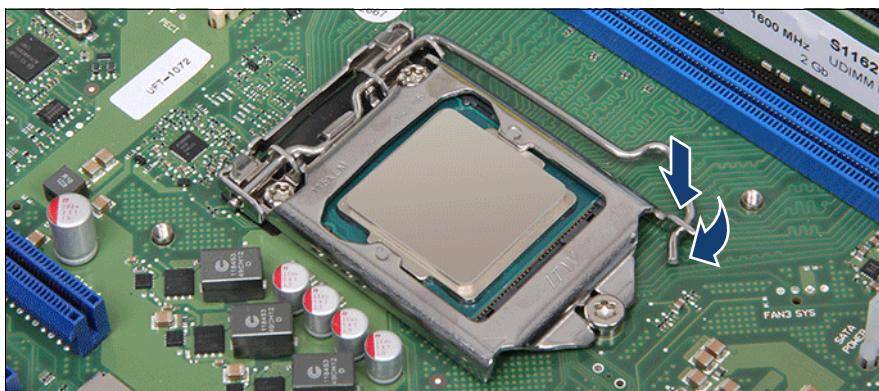
図 127: ソケットレバーのラッチ留め
