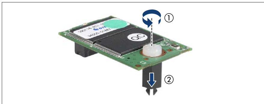
図 180: 新しい UFM の準備
