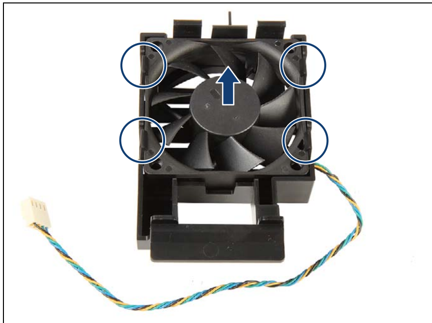
図 76: 2.5 インチファンホルダーからのファンの取り外し
