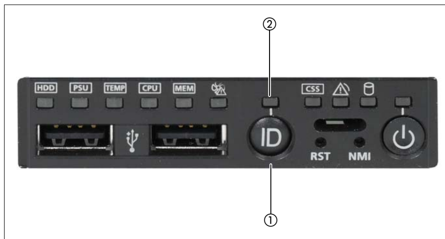
図 2: フロントパネルの ID ボタンとランプ
