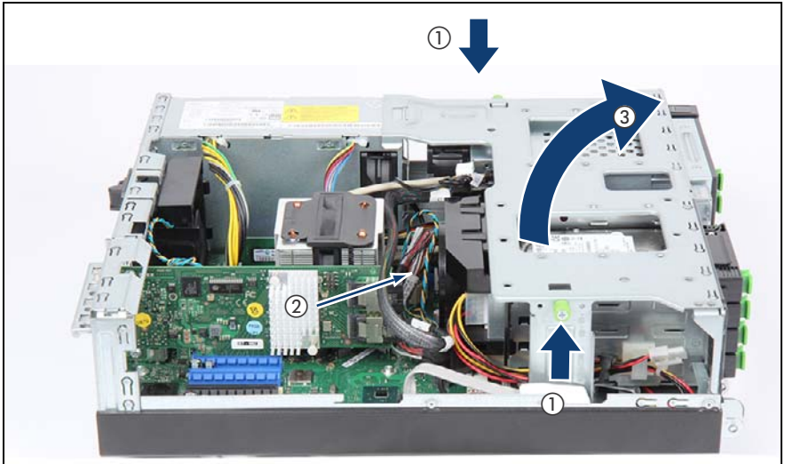
図 17: フロントケースを開く
