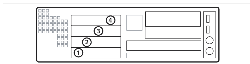
図 35: 2.5 インチ HDD/SSD の取り付け順序
