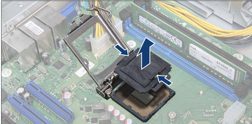
図 199: ソケット保護カバー（新しいシステムボード）の取り外し
