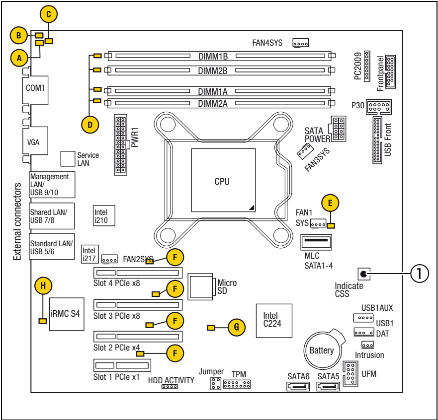
図 211: オンボード表示ランプと CSS ボタン
