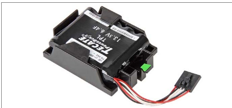
図 89: FBU を FBU ホルダーへの取り付け (B)
