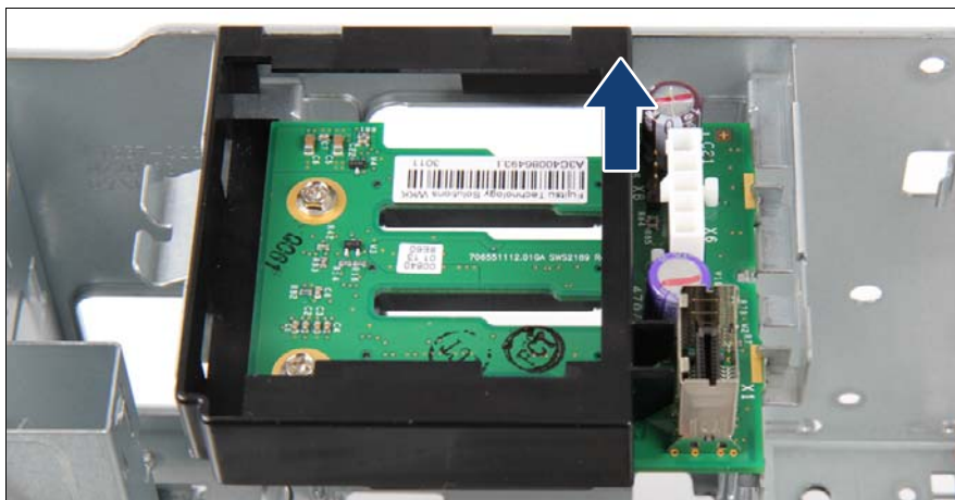
図 52: 送風ダクトを持ち上げる
