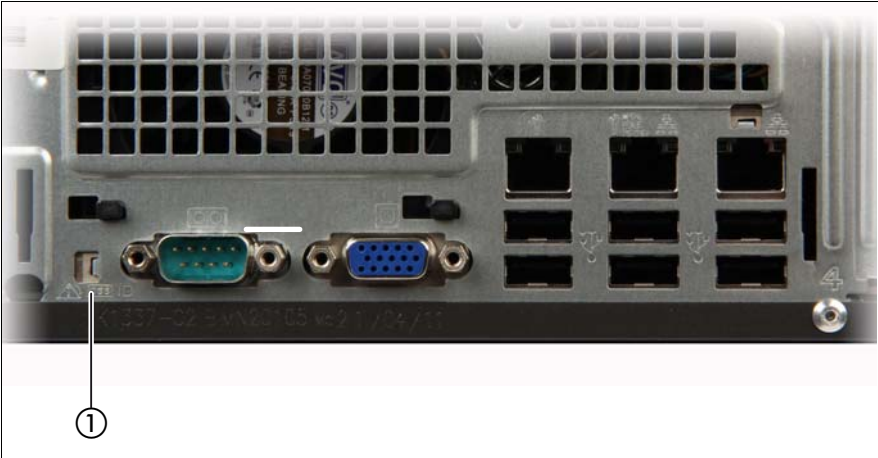
図 213: コネクタパネルの表示ランプ : CSS ランプ、保守ランプ、およびシステム ID ランプ
