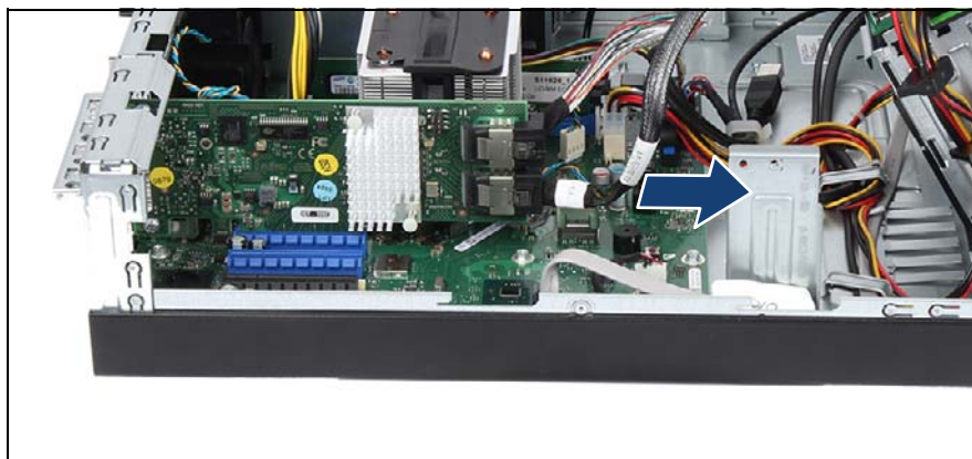
図 163: RAID コントローラからの SATA ケーブルの取り外し
