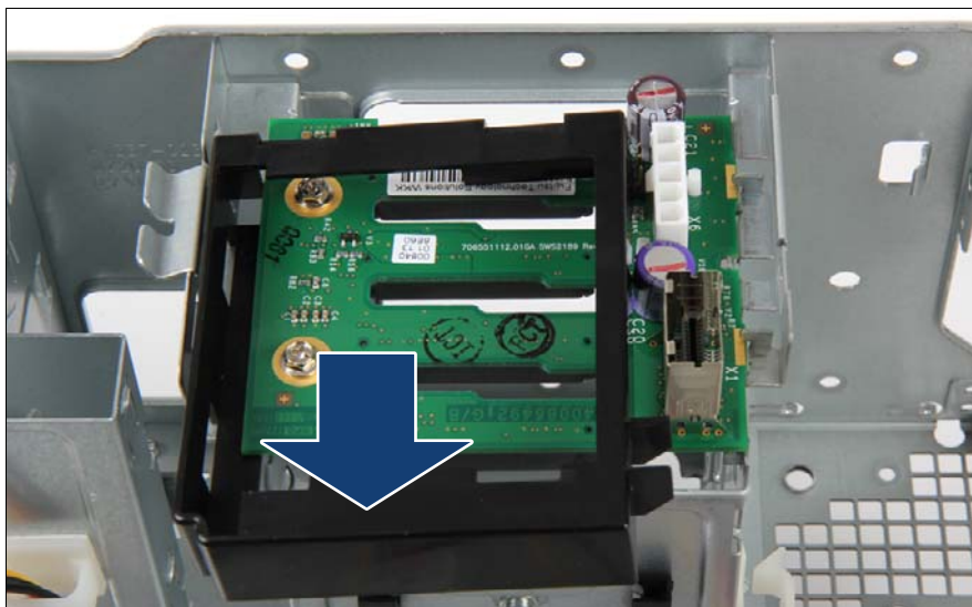
図 53: 送風ダクトの取り外し
