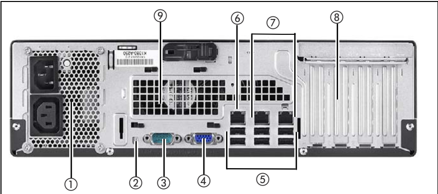
図 207: PRIMERGY TX1320 M1 背面
