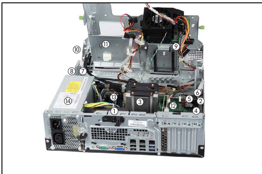
図 208: PRIMERGY TX1320 M1 内部 (2.5 インチ HDD / 標準 PSU モデル)
