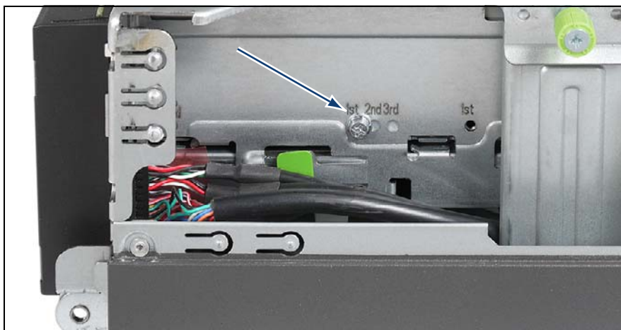
図 153: バックアップドライブからネジを取り外す
