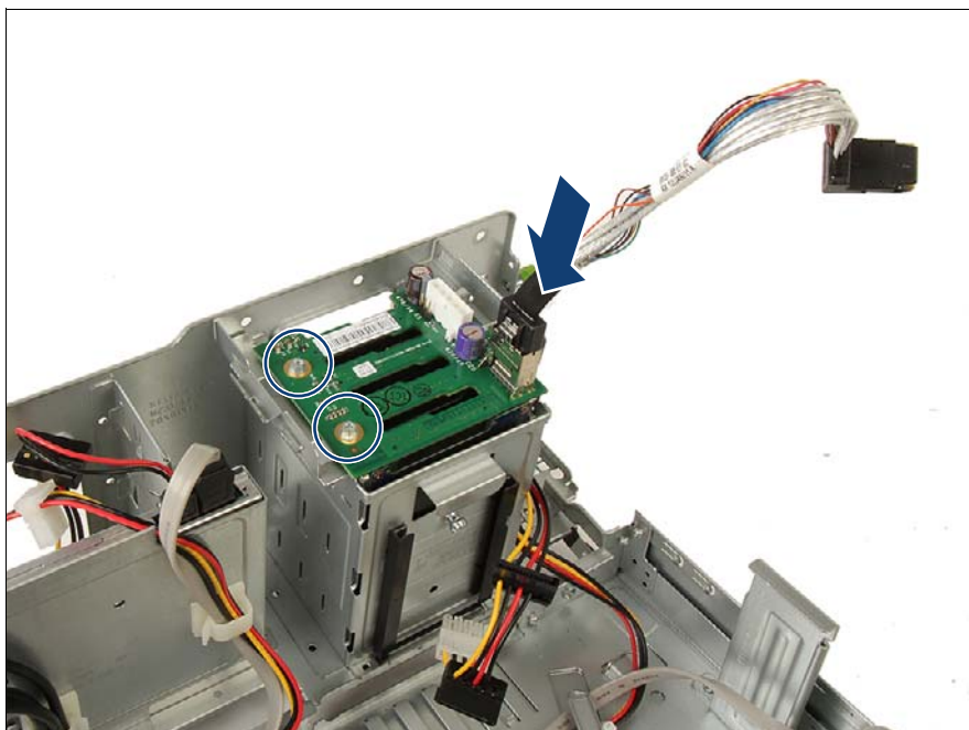
図 57: 2.5 インチ HDD SAS/SATA バックプレーンへのケーブルの接続
