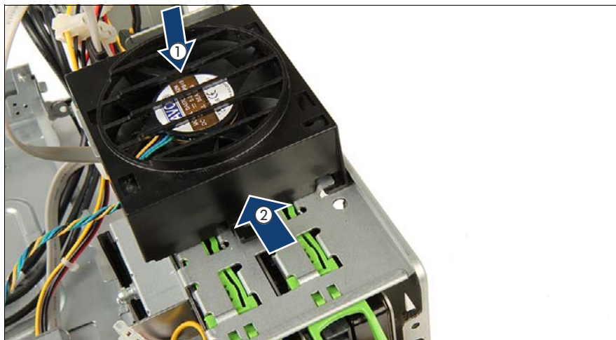
図 72: HDD ファンモジュールの取り付け
