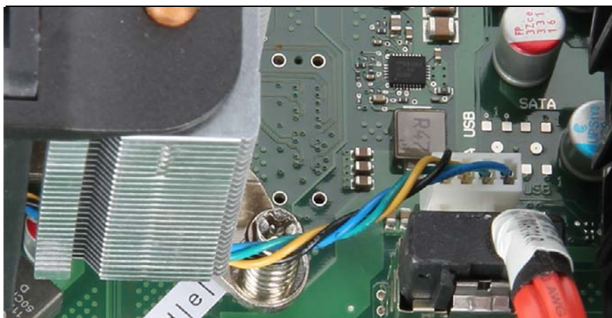
図 132: ヒートシンクを取り付ける (B)
