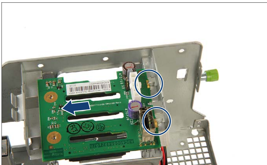
図 55: 2.5 インチ HDD SAS/SATA バックプレーンの取り外し
