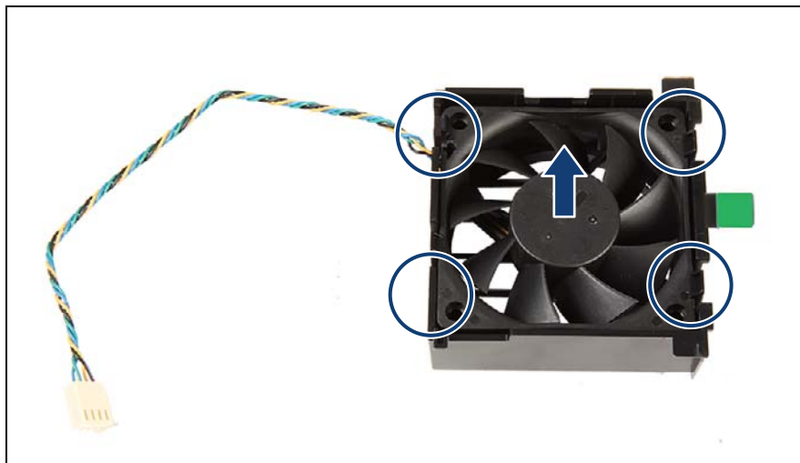
図 63: ホルダーからのファンの取り外し
