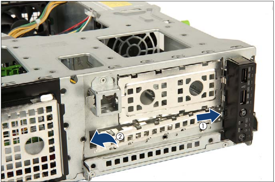
図 145: ODD フィラーカバーを挿入します。
