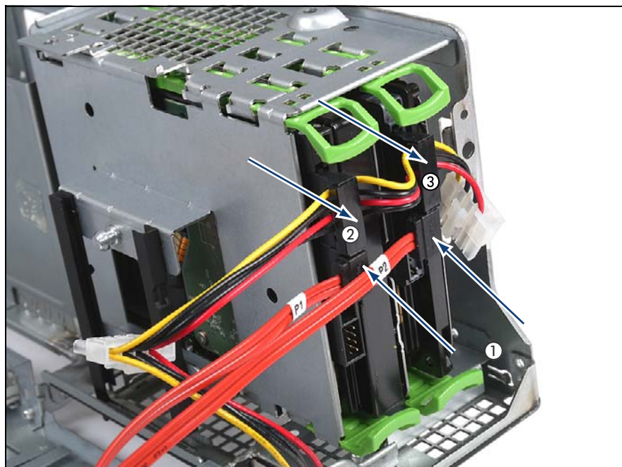
図 47: ケーブルの接続
