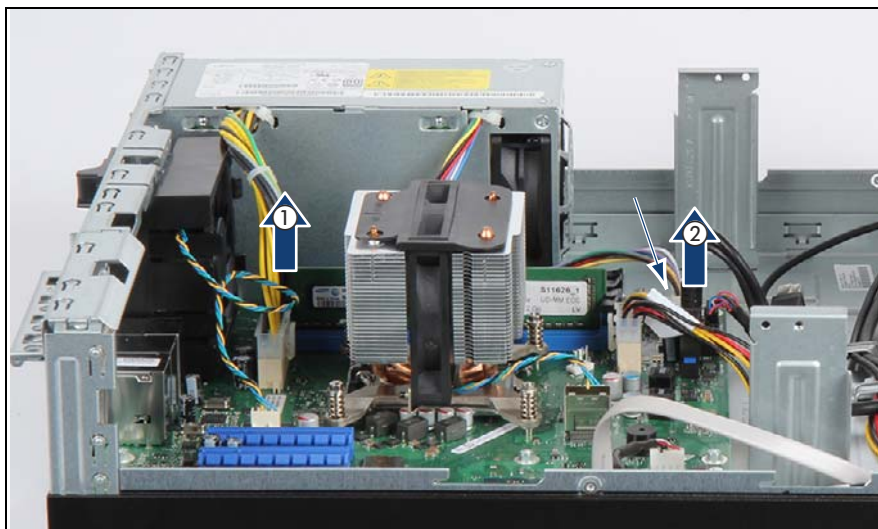
図 29: 内部電源ケーブルの取り外し
