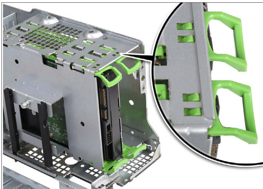
図 46: 3.5 インチ HDD モジュールの取り付け
