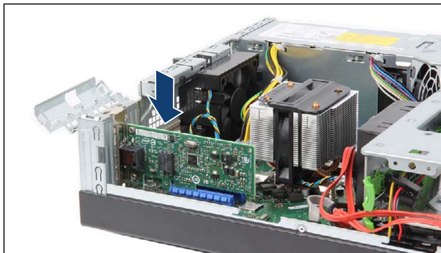
図 82: 拡張カードの取り付け
