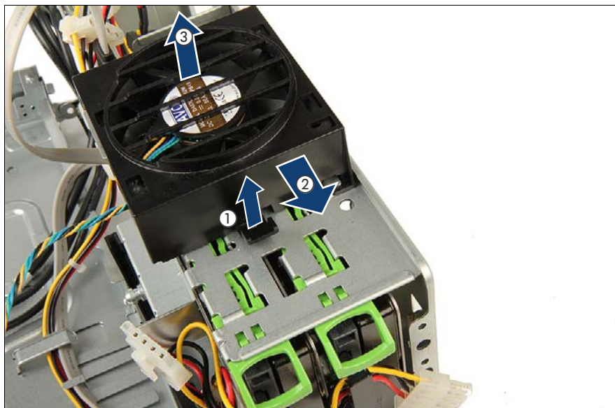
図 68: HDD ファンモジュールの取り外し
