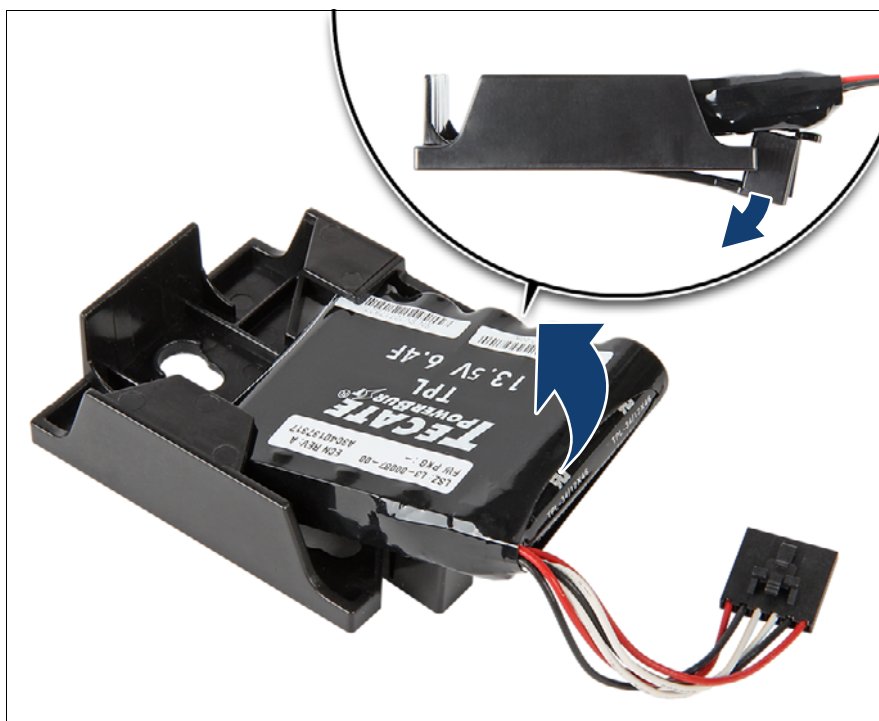
図 98: FBU を FBU ホルダーから取り外す
