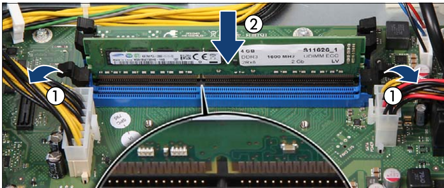
図 120: メモリモジュールの取り付け
