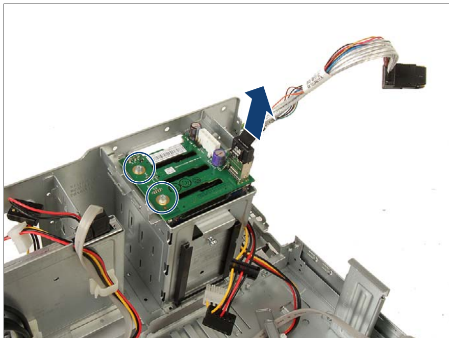
図 54: 2.5 インチ HDD SAS/SATA バックプレーンからのケーブルの取り外し
