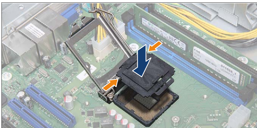
図 200: ソケット保護カバーを取り付けます（故障しているシステムボード）(A)
