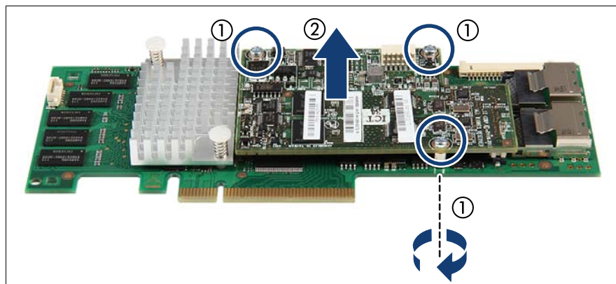
図 85: TFM の取り外し
