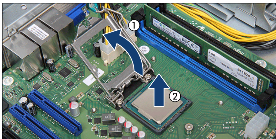
図 123: プロセッサの取り外し
