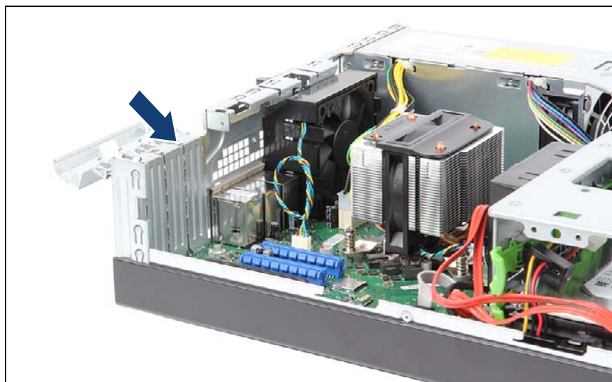
図 84: PCI スロットブラケットの取り付け
