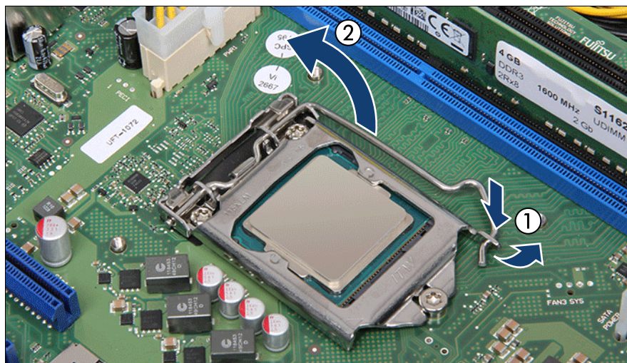
図 122: ソケットレバーのラッチを外す
