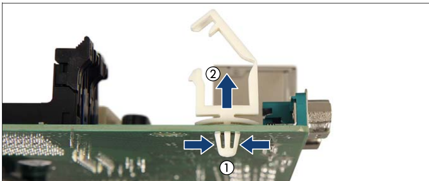
図 194: 電源ケーブルクランプの取り外し
