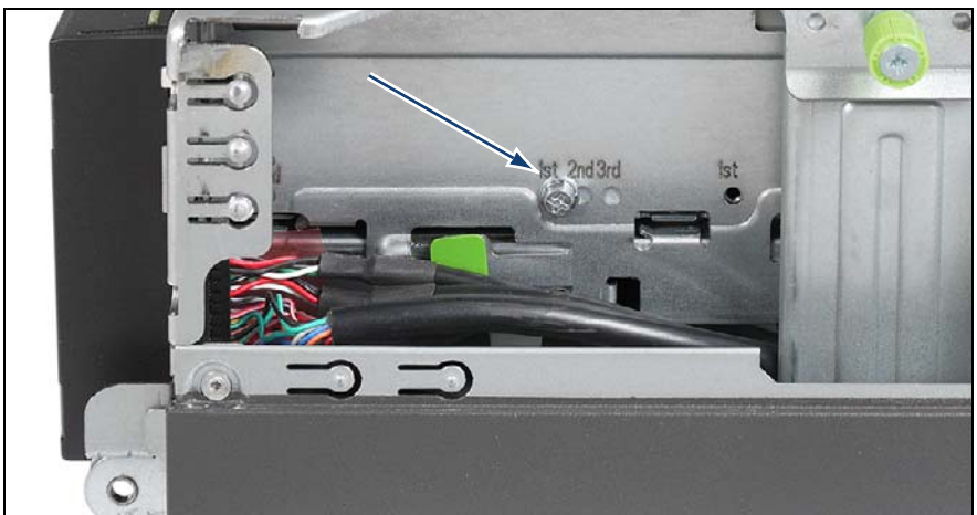
図 150: ネジの挿入
