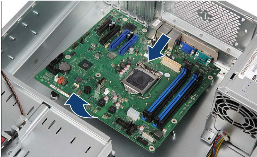
図 193: システムボードの取り外し
