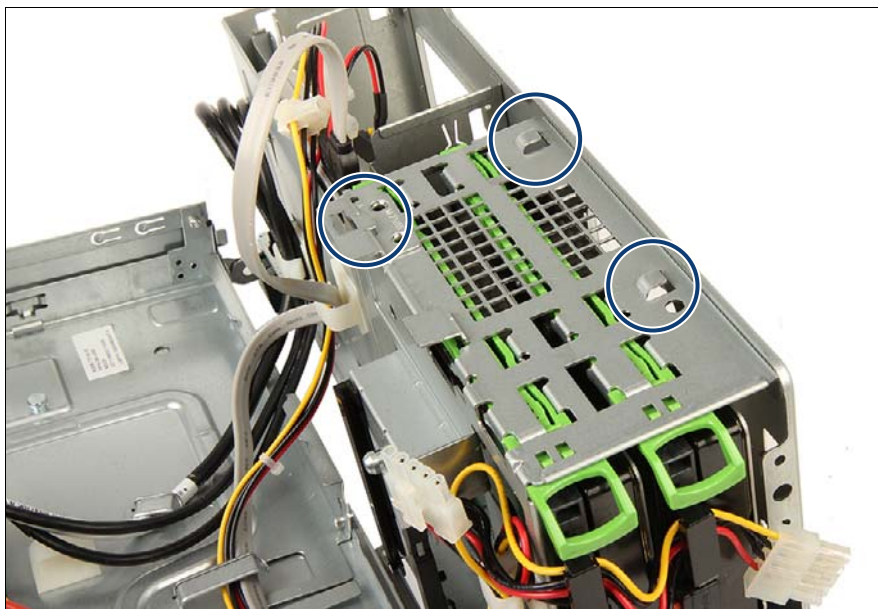
図 71: 保持ブラケットの再取り付け
