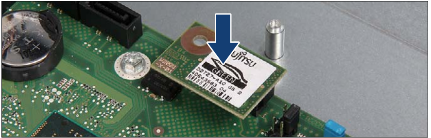
図 186: TPM の取り付け
