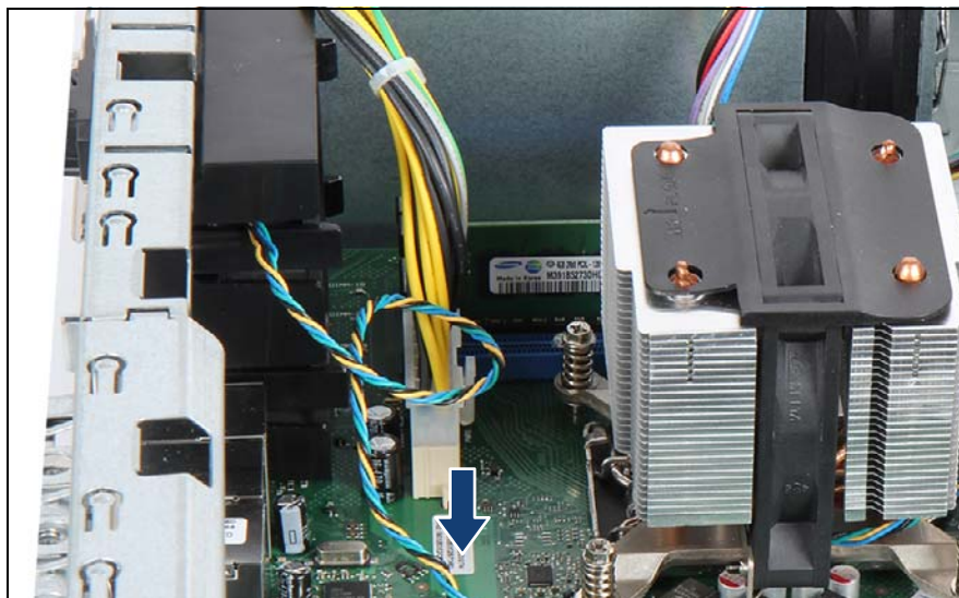
図 67: システムファンケーブルの接続
