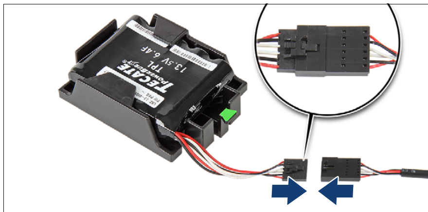
図 90: FBU への FBU アダプタケーブルの接続
