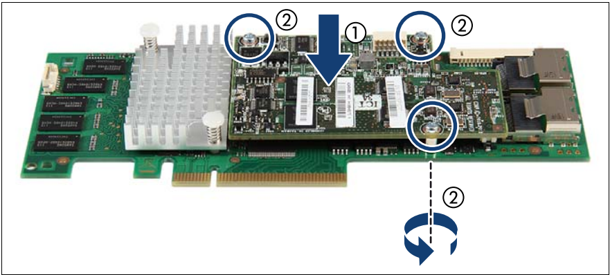
図 87: TFM の取り付け
