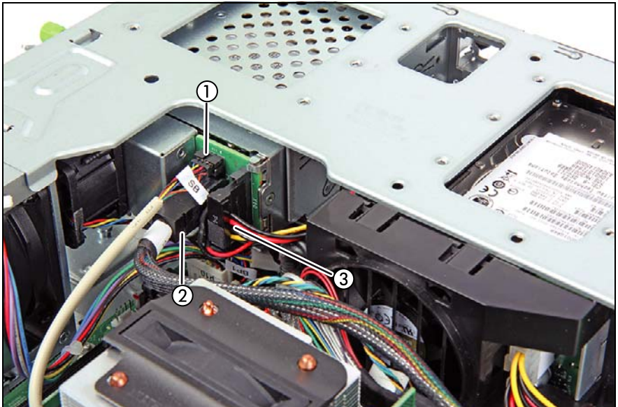
図 160: ベイ追加オプションの取り付け
