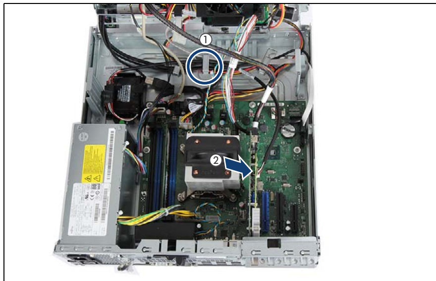
図 93: FBU のケーブル配線
