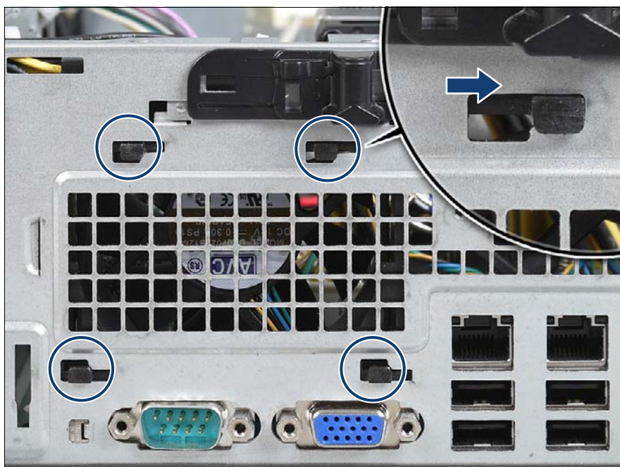
図 66: システムファンモジュールの取り付け (B)
