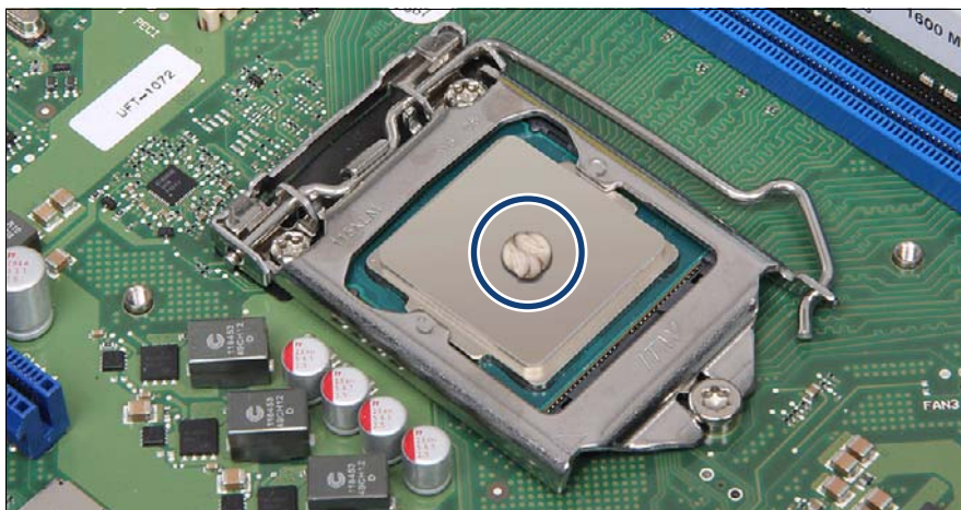
図 129: サーマルペーストの塗布
