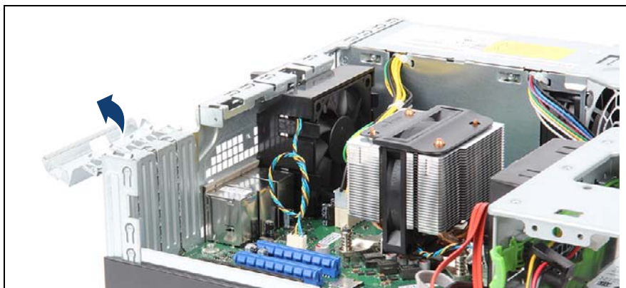
図 80: PCI スロットブラケットのクランプを開ける
