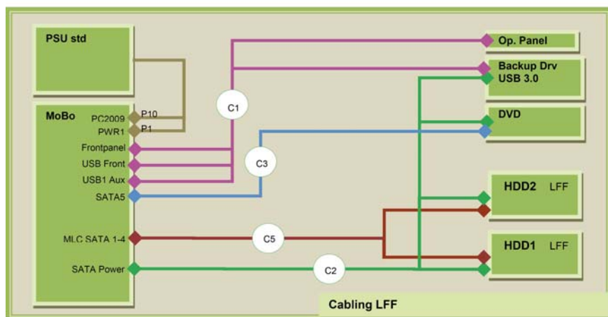
図 203: ケーブル配線 - 2x 3.5 インチ HDD モデル (LFF)
