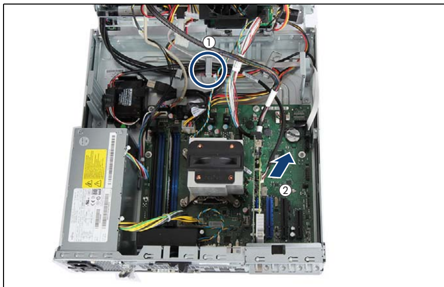
図 95: FBUホルダーの取り外し
