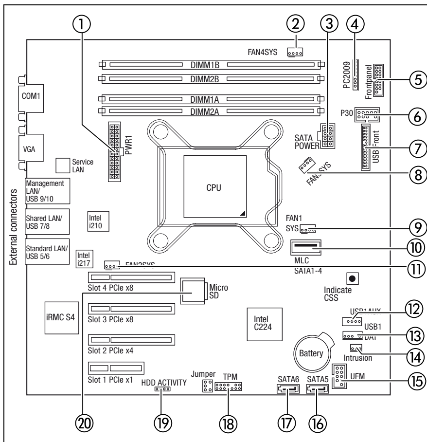
図 209: システムボード D3239 の内部コネクタ
