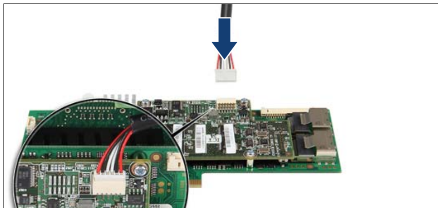
図 92: TFM への FBU アダプタケーブルの接続
