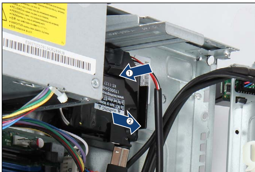
図 91: FBU ホルダーの取り付け
