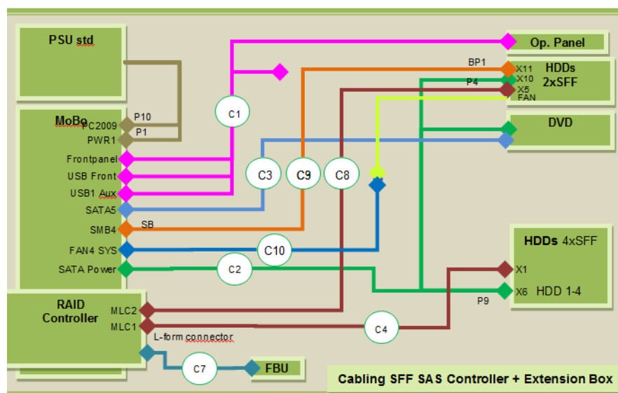
図 205: ベイ追加オプションとのケーブル配線
