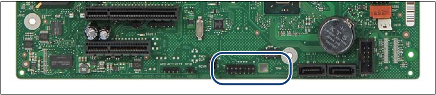
図 184: TPM の取り付け位置
