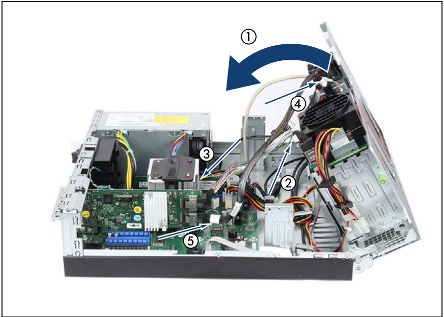
図 19: フロントケースを閉じる
