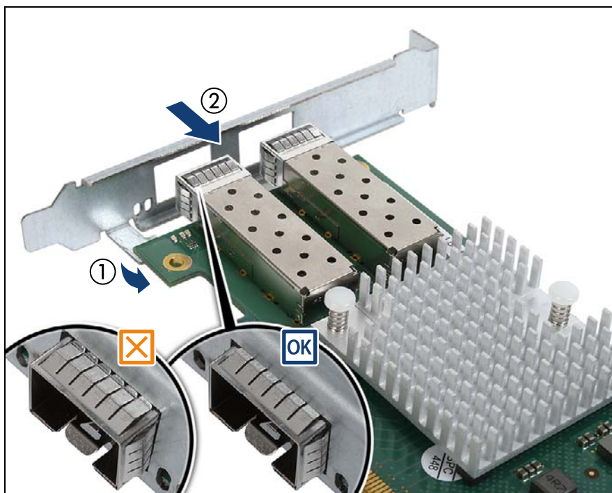
図 106: ネットワークアダプタ D2755 - スロットブラケットの取り付け (A)
