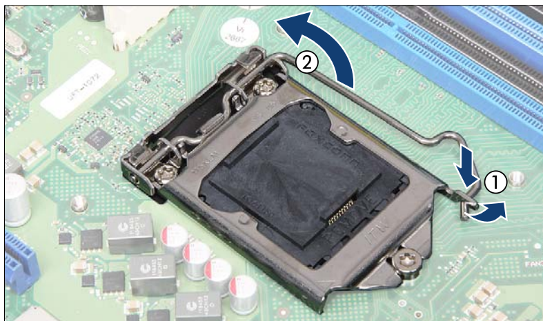
図 198: ソケットレバー（新しいシステムボード）のラッチを外します。
