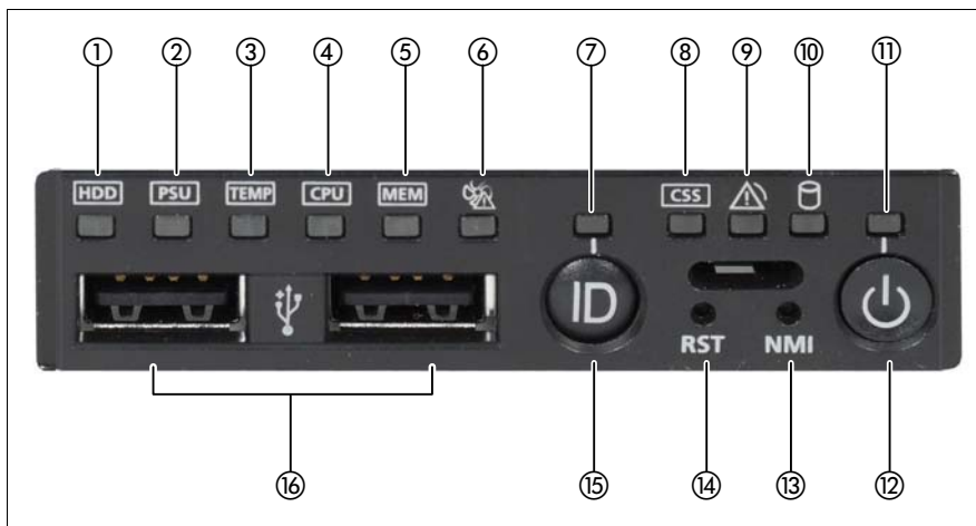
図 214: 前面 (表示ランプとコントロール)
