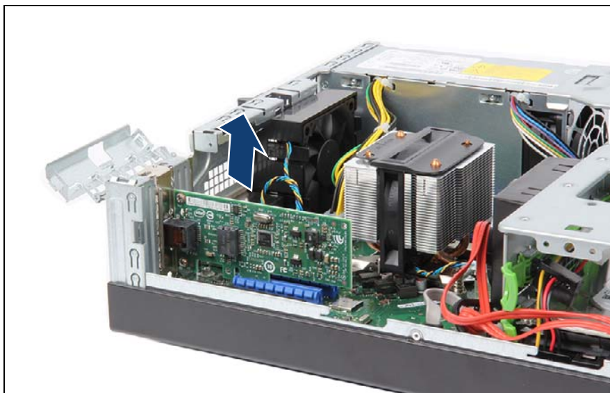
図 83: 拡張カードの取り外し
