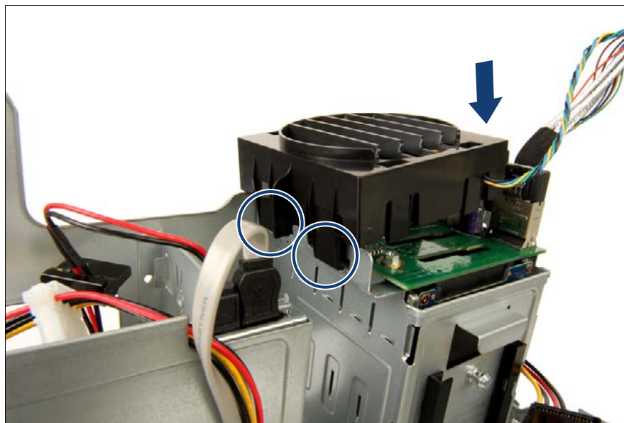
図 78: HDD ファンモジュールホルダーの挿入
