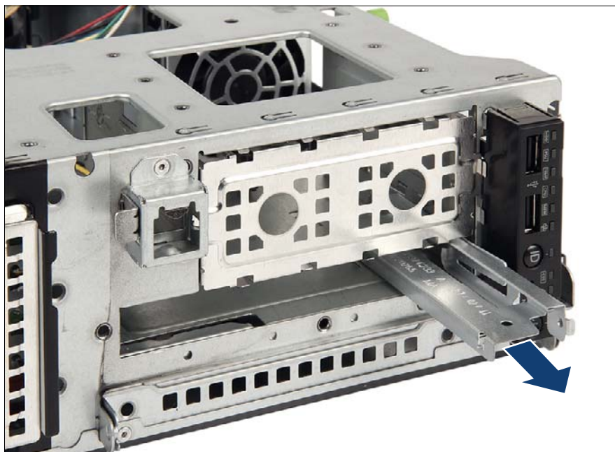
図 135: ODD 取り付けブラケットの取り外し
