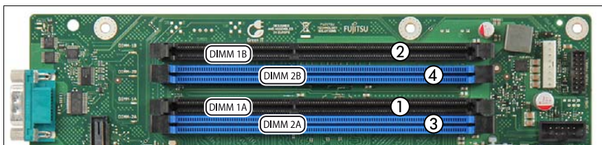
図 118: メモリの概観
