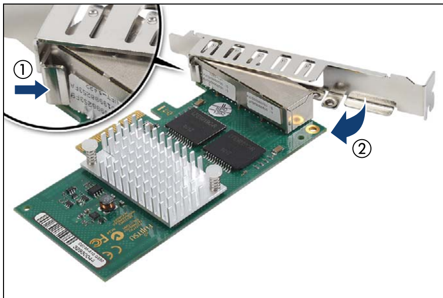
図 103: ネットワークアダプタ D2745 - スロットブラケットの取り付け (A)
