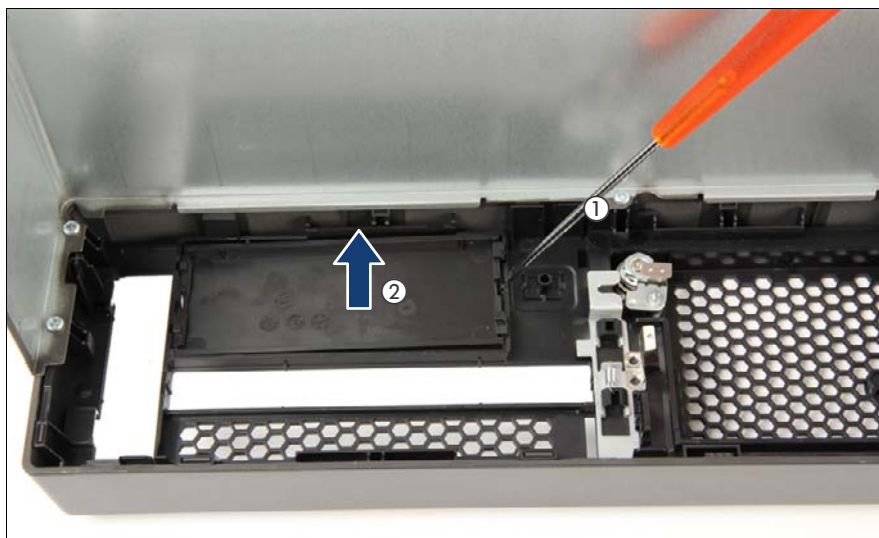
図 147: ダミーカバーの取り外し
