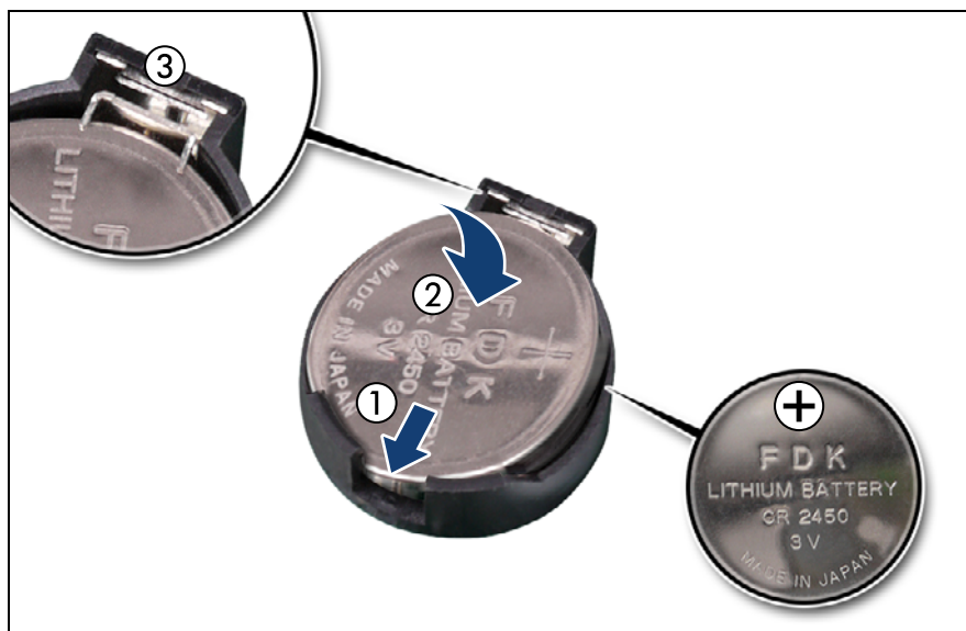
図 174: CMOS バッテリーの取り付け
