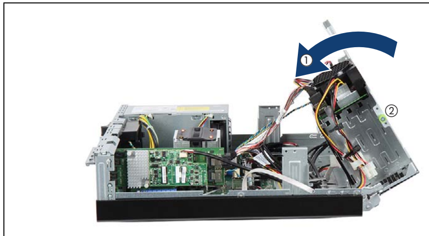
図 18: フロントケースを閉じる
