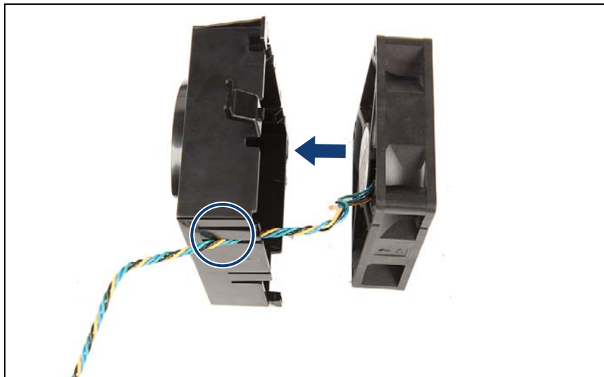
図 70: 3.5 インチファンホルダーへのファンの取り付け
