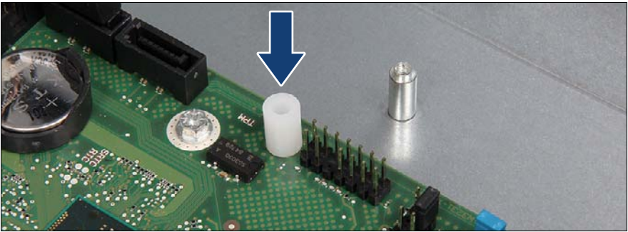
図 185: TPM スペースーの取り付け
