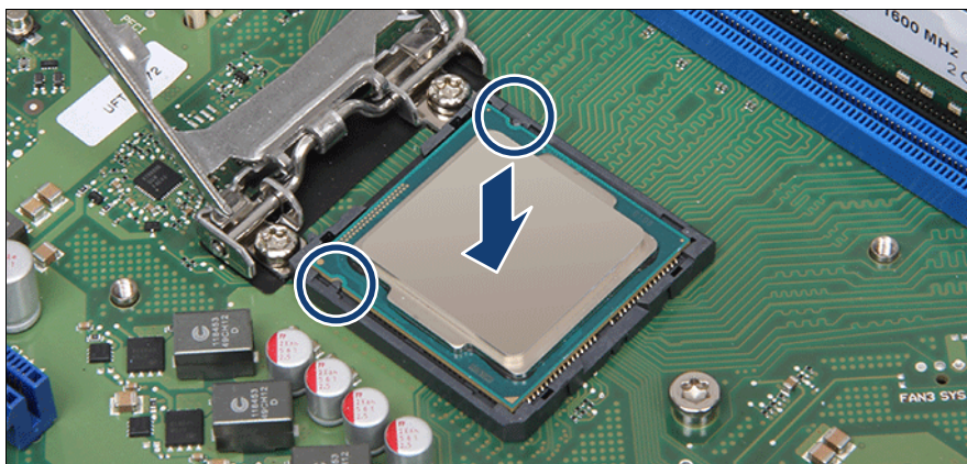
図 124: プロセッサを取り付ける
