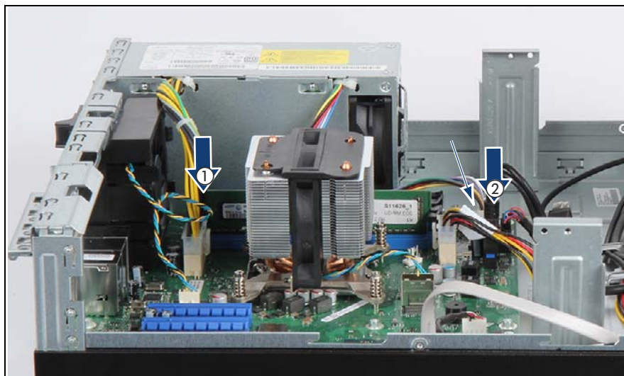
図 34: 内部電源ケーブルの接続
