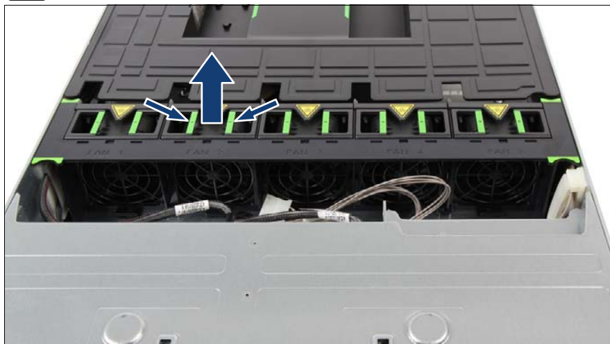
図 65: システムファンの取り外し
