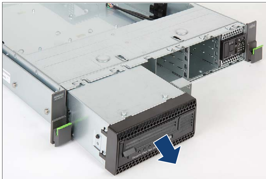
図 226: ドライブページの取り外し
