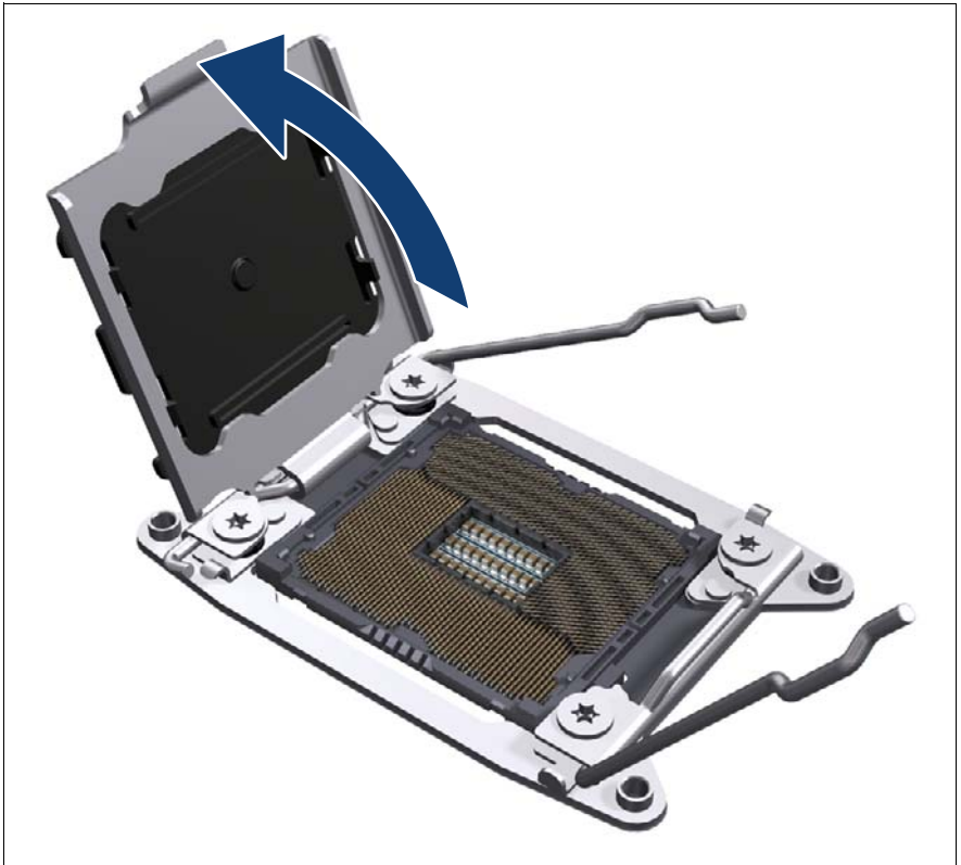
図 146: ロードプレートを開く (B)
