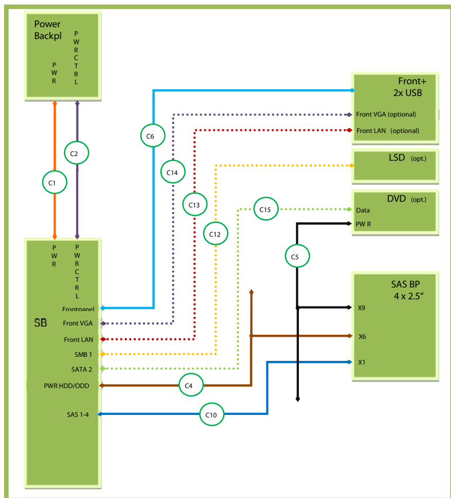
図 338: SAS オンボードコネクタによる 4x 2.5 インチ HDD モデルのケーブル配線
