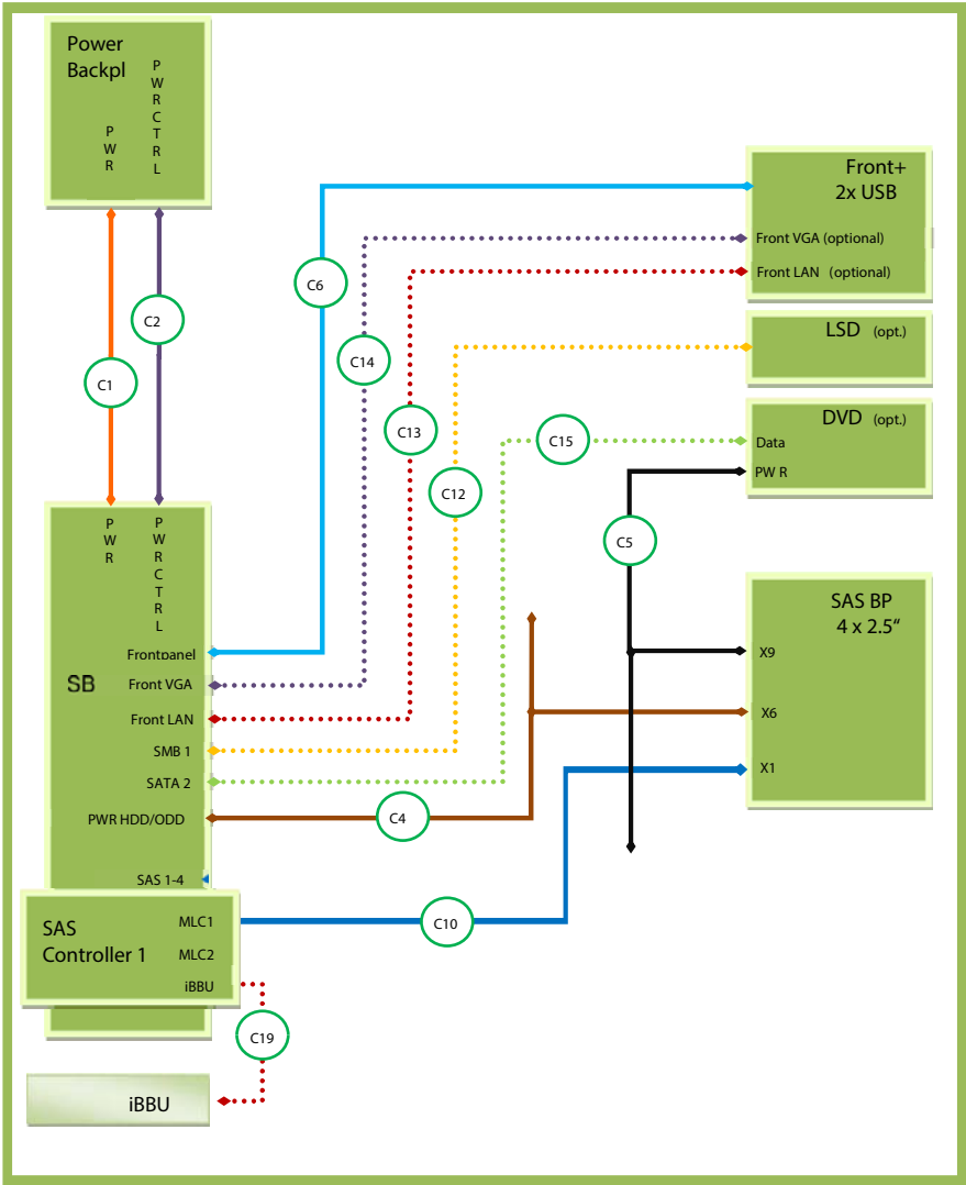
図 339: SAS コントローラによる 4x 2.5 インチ HDD モデルのケーブル配線
