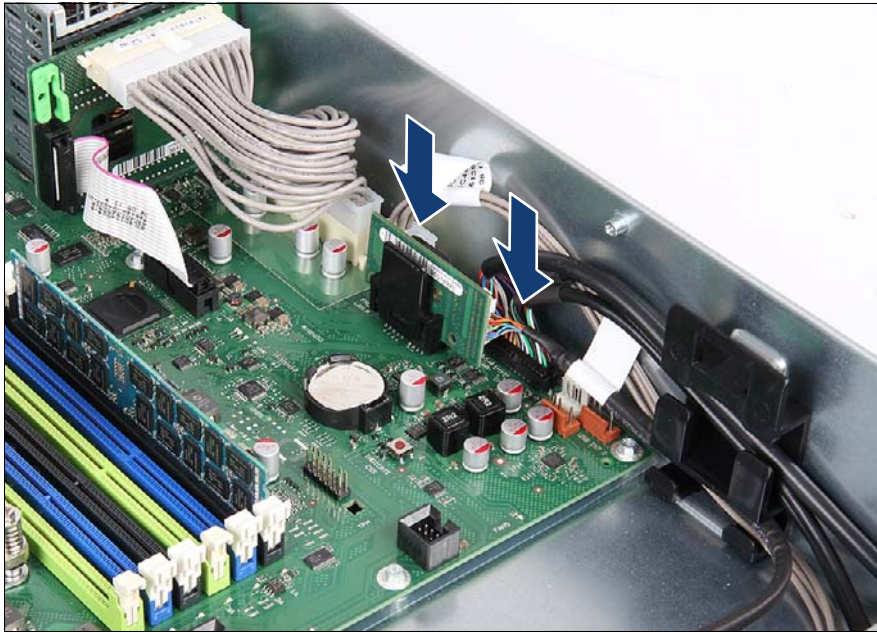
図 255: フロントパネルケーブルの接続
