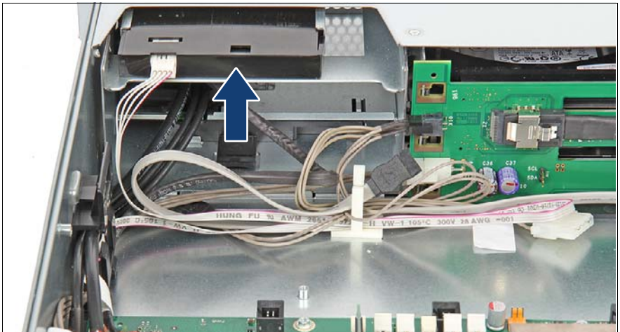
図 182: ODD ダミーモジュールの取り外し
