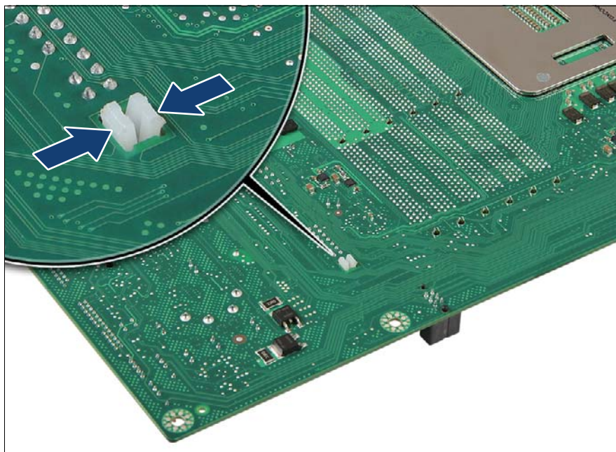
図 285: TPM スペーサーの取り外し
