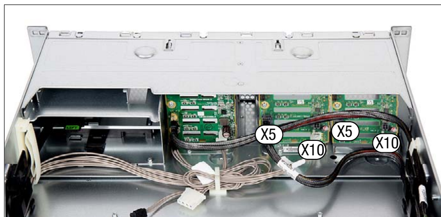
図 326: SAS ケーブルの接続
