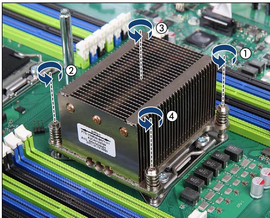
図 167: プロセッサヒートシンクの取り外し (A)
