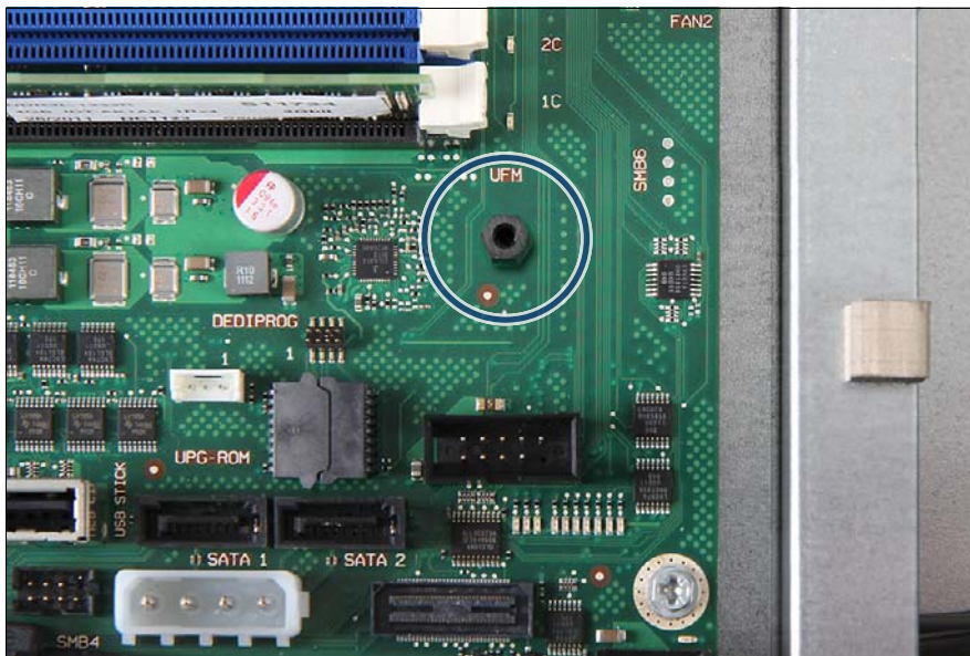
図 274: UFM を取り外す (B)
