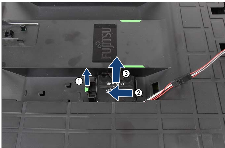
図 124: 送風ダクトからの FBU ホルダーの取り外し (A)
