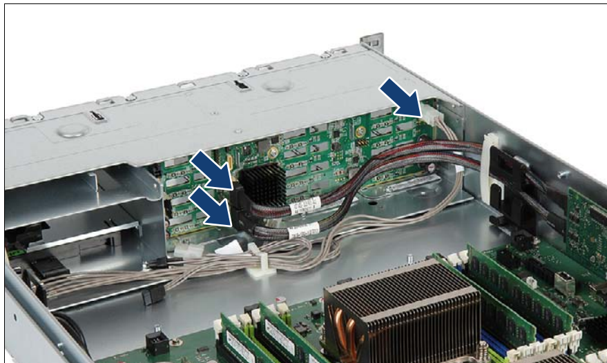
図 61: 12x 2.5 インチ HDD SAS バックプレーンからのケーブルの取り外し
