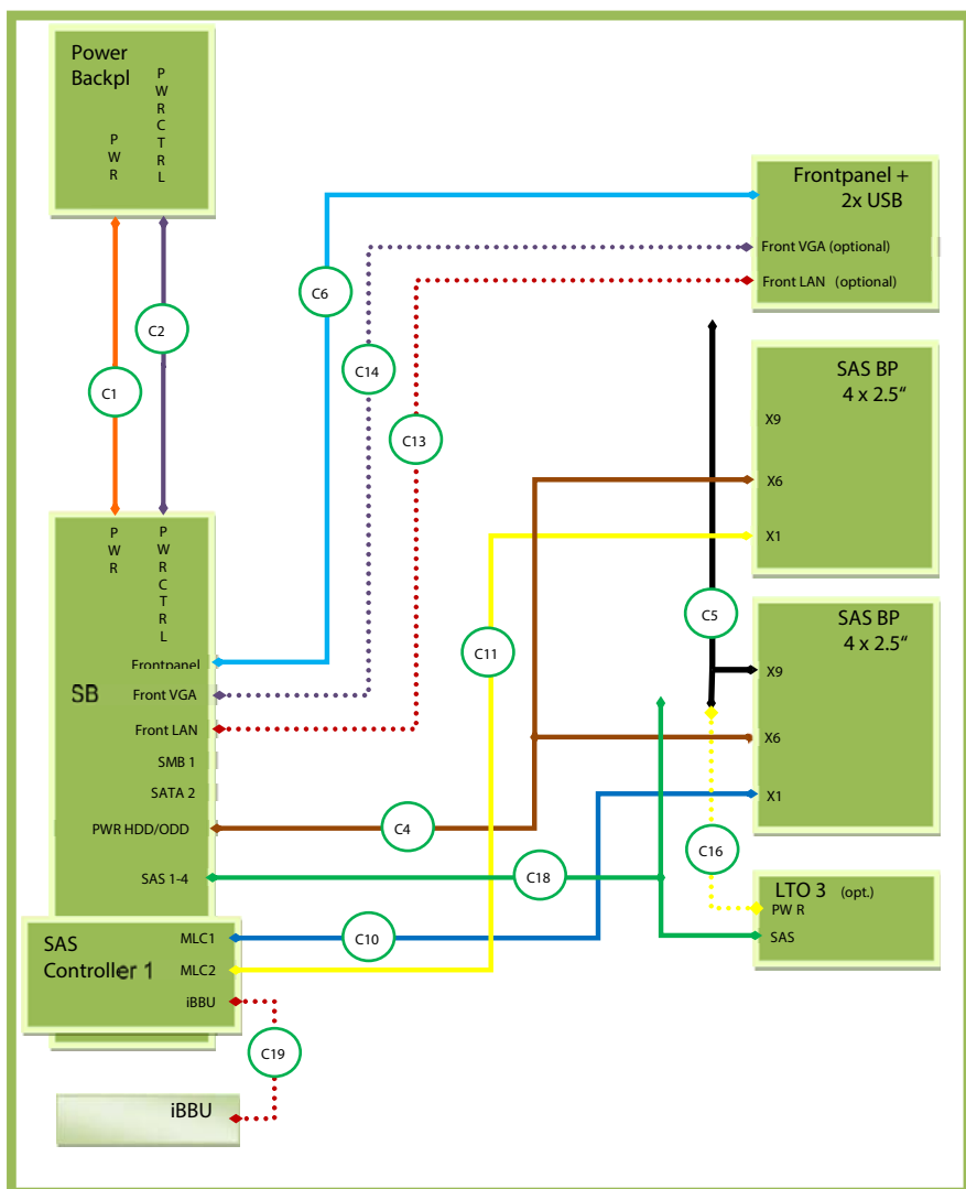
図 346: ケーブル配線 - LTO3 テープドライブ 8x 2.5 インチ HDD モデル
