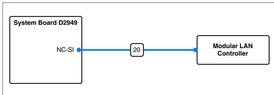
図 355: Modular LAN NCSI サイドバンドのケーブル配線
