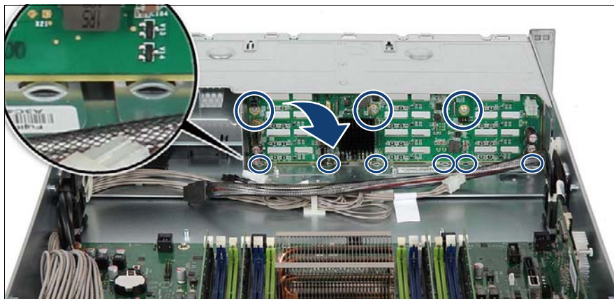
図 62: 2.5 インチ HDD SAS バックプレーンの取り外し (A)
