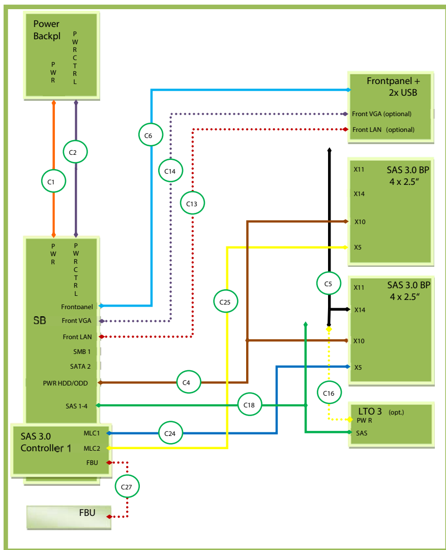
図 352: ケーブル配線 - 8x2.5 インチ SAS 3.0 HDD + LTO3 モデル
