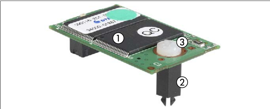
図 270: UFM キット
