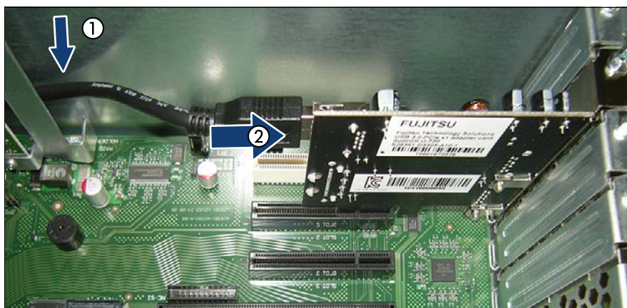
図 209: USB ケーブルの USB 3.0 インタフェースカードへの接続
