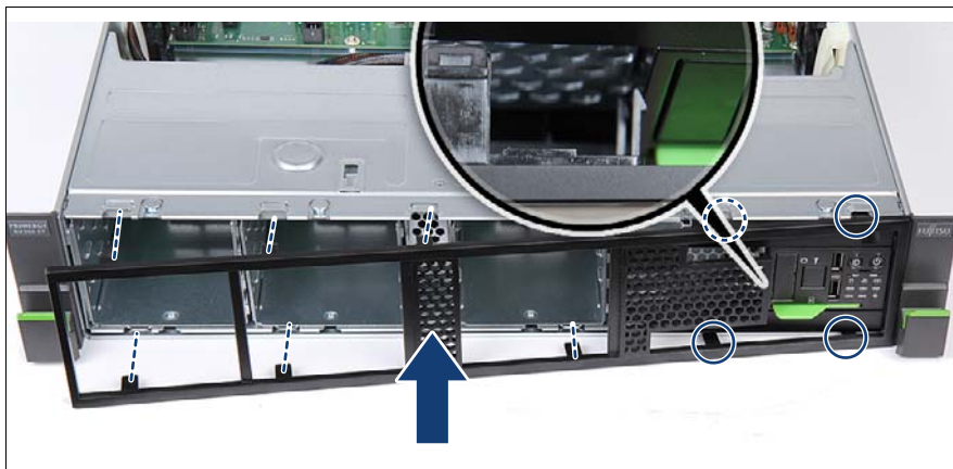
図 304: マルチケース付き構成でのフロントカバーの取り付け
