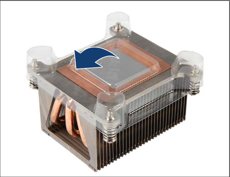
図 164: ヒートシンク保護カバーの取り外し
