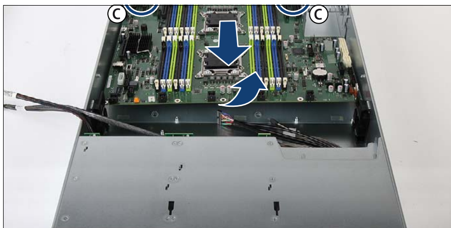
図 295: システムボードの取り外し
