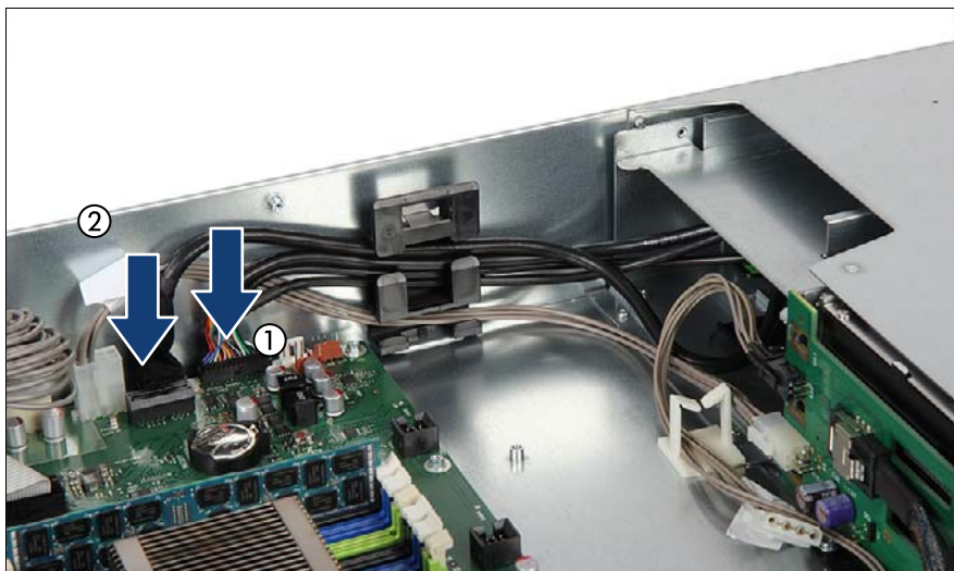
図 243: フロントパネルケーブルの接続
