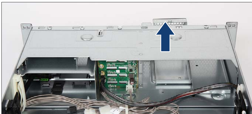
図 306: 2.5 インチダミーケージの取り外し
