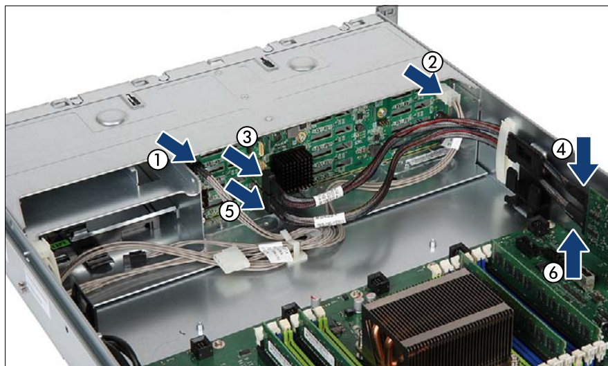
図 317: SAS ケーブルの接続
