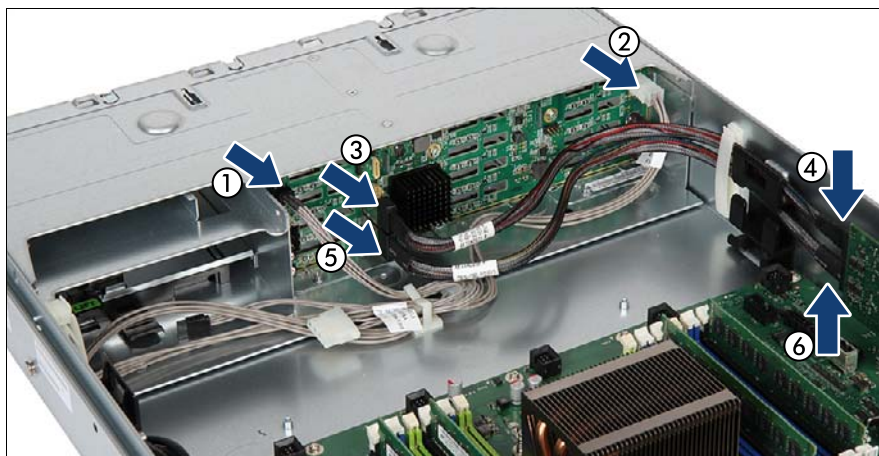
図 335: SAS ケーブルの接続
