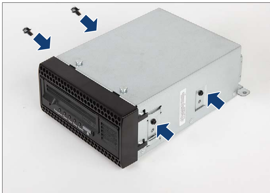
図 219: LTO ドライブのドライブケースへの固定
