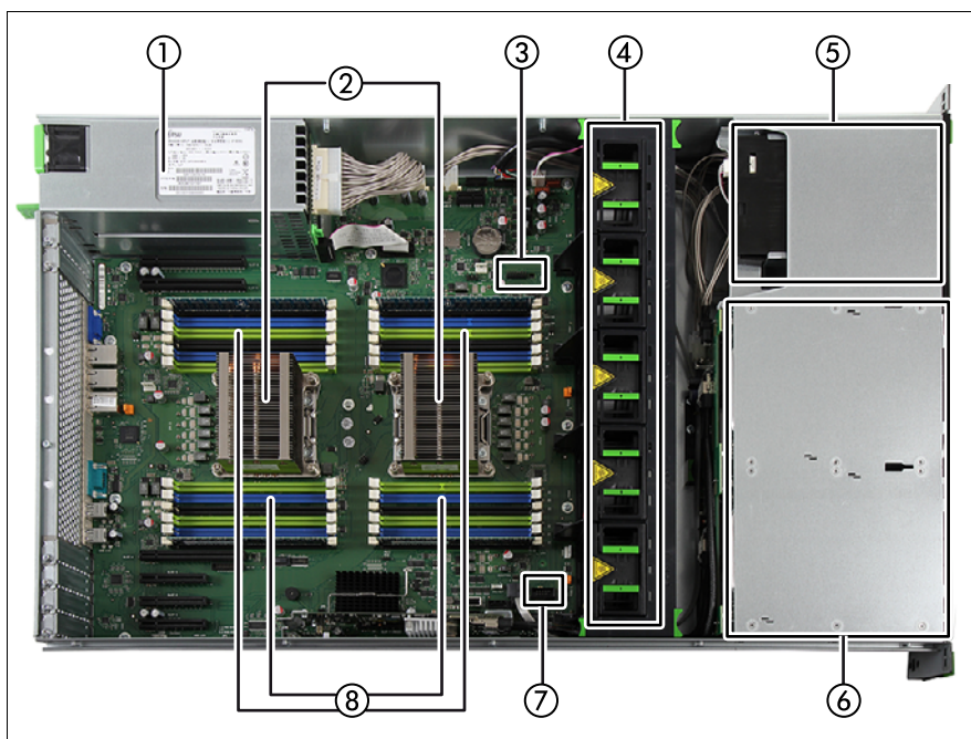
図 358: PRIMERGYRX300 S8 内部 (例: 2.5 インチ HDD モデル)
