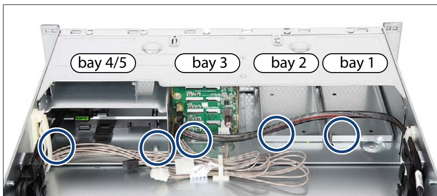
図 302: HDD ケージとフロントパネルケージの取り外し
