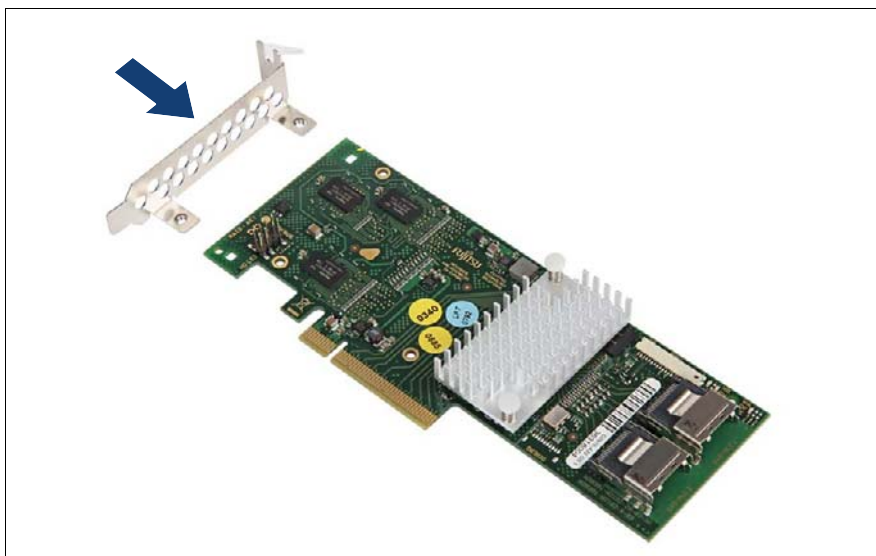
図 73: 標準スロットブラケットの取り付け (A)
