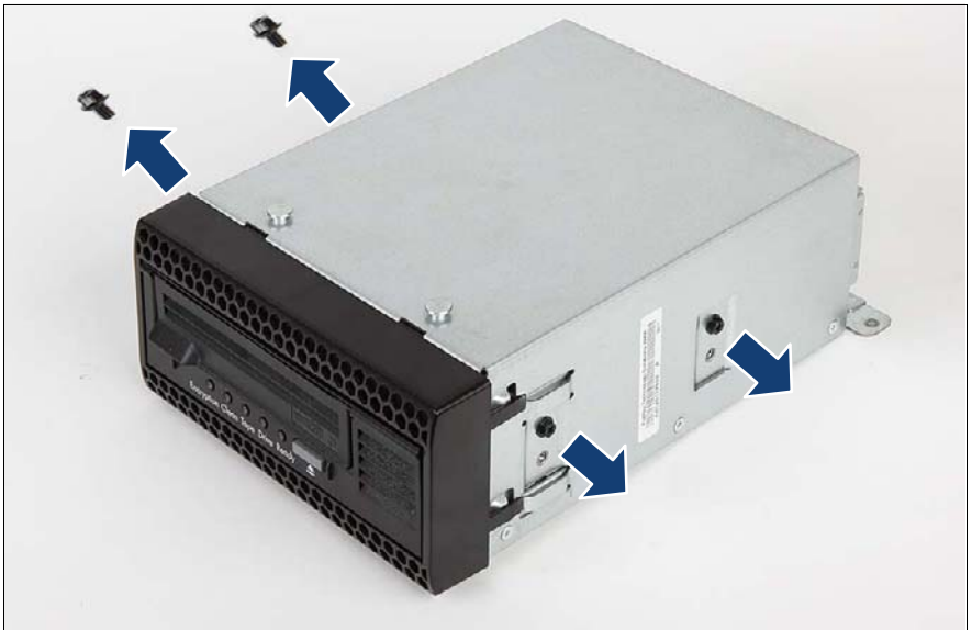
図 228: ネジの取り外し
