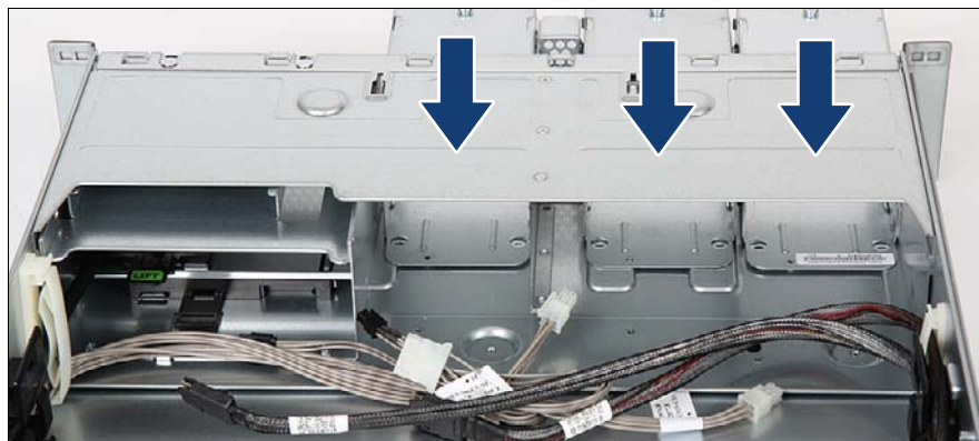
図 314: HDD ケージの取り付け
