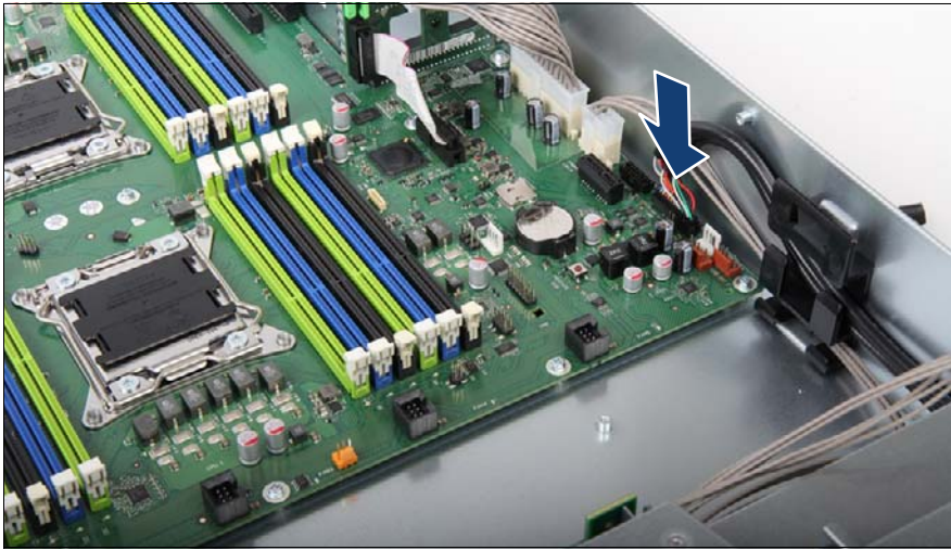
図 239: フロントパネルケーブルの接続
