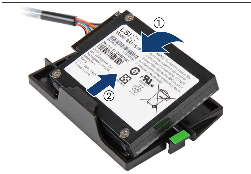
図 109: BBU ホルダーからの BBU の取り外し
