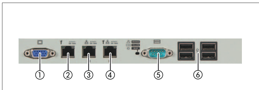
図 361: PRIMERGYRX300 S8 背面
