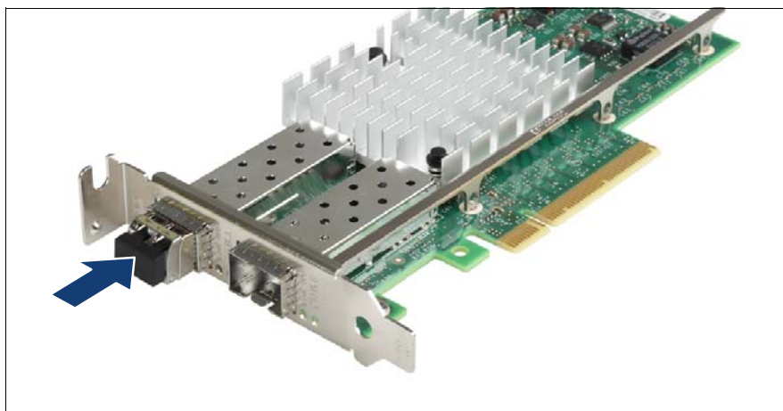
図 131: 光ポート保護プラグの取り付け
