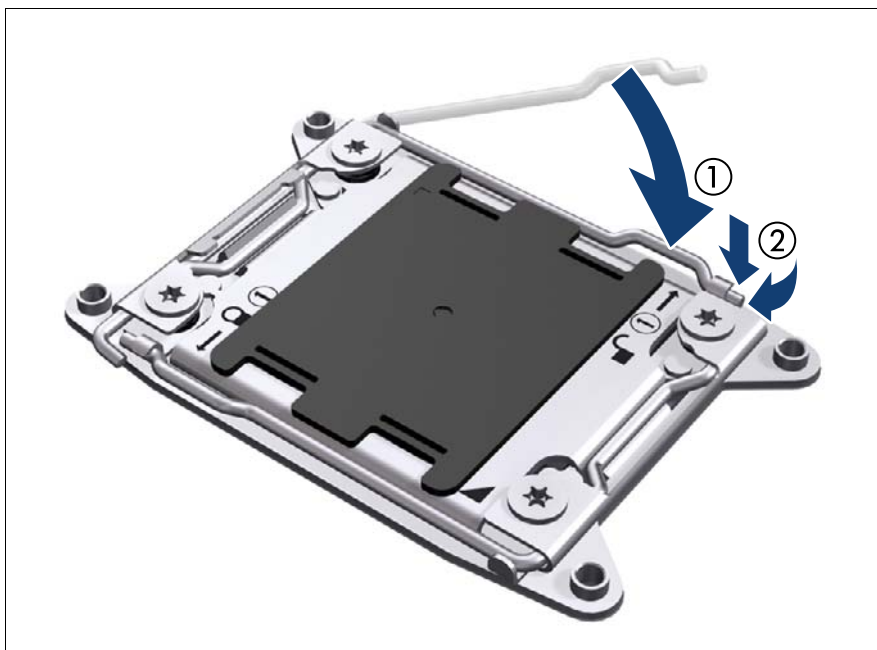
図 161: ソケットリリースレバー 1 を閉じます。
