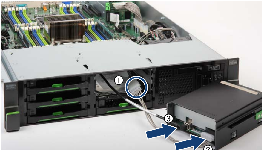
図 194: テープ /RDX ドライブへのケーブルの接続
