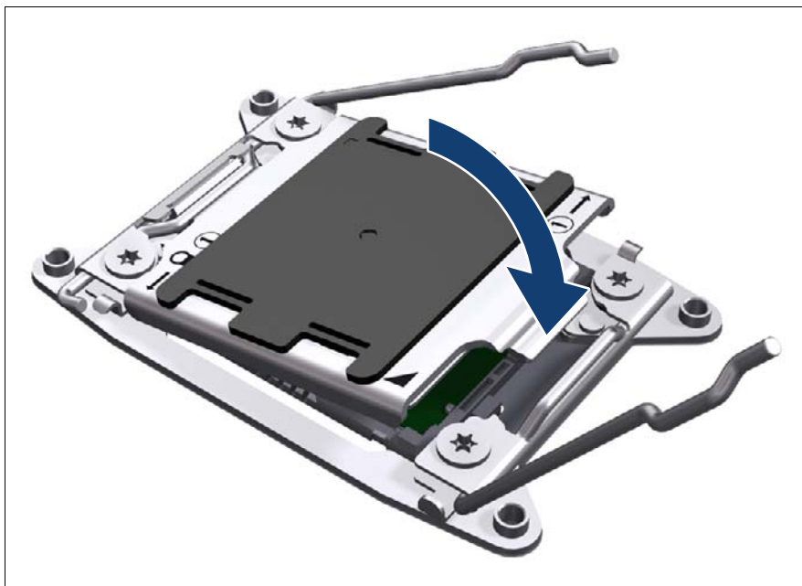
図 148: ロードプレートを閉じる
