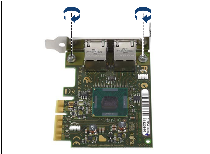
図 76: ネットワークアダプタ D2735 - スロットブラケットの取り付け (B)
