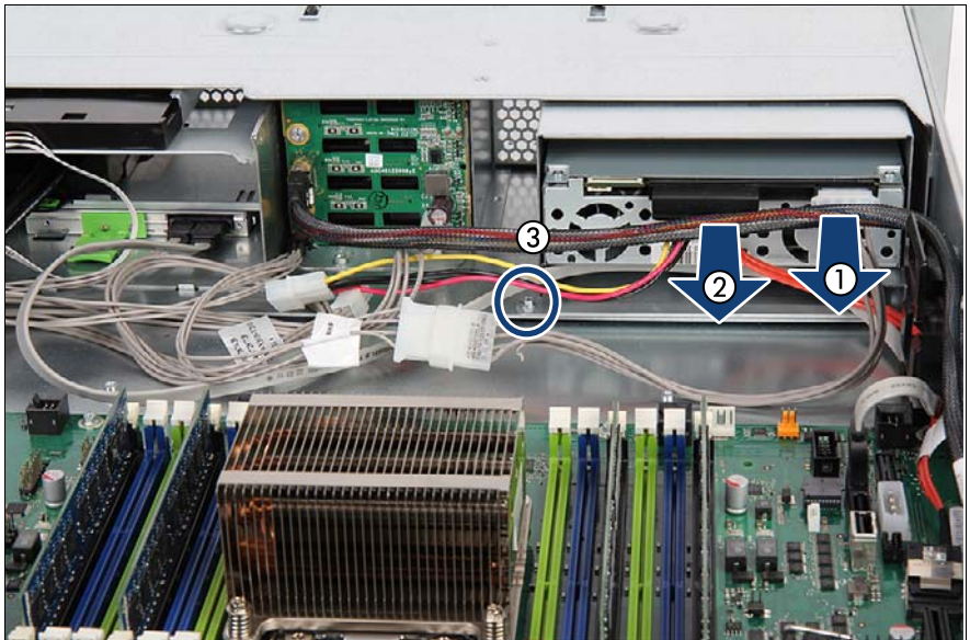
図 225: ドライブケースの解除
