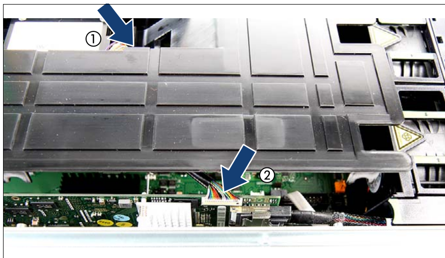
図 106: コントローラへの BBU の接続
