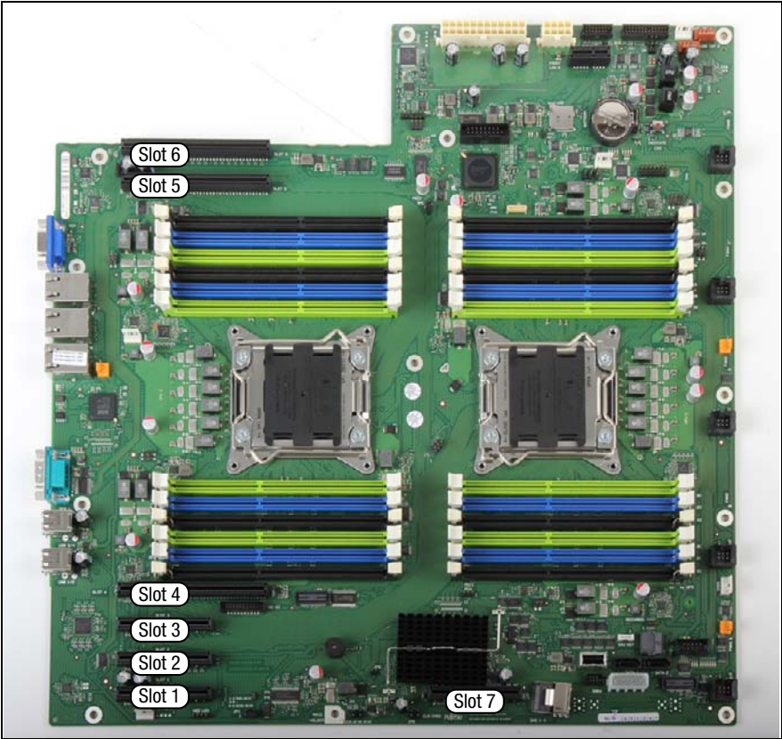
図 72: PCI スロットの概観
