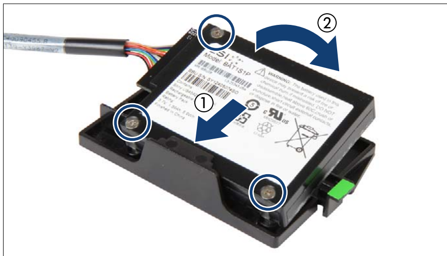
図 103: BBUホルダーへのBBUの取り付け（例B）
