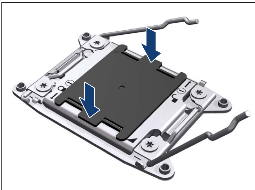
図 159: ソケット保護カバーの取り付け (B)
