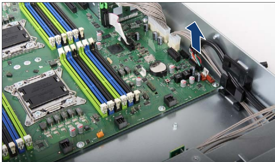
図 234: フロントパネルモジュールのケーブルの取り外し
