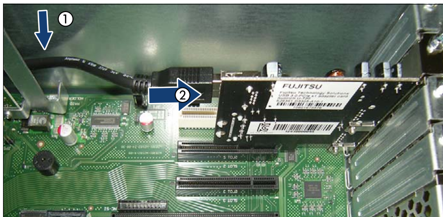
図 198: USB ケーブルの USB 3.0 インタフェースカードへの接続
