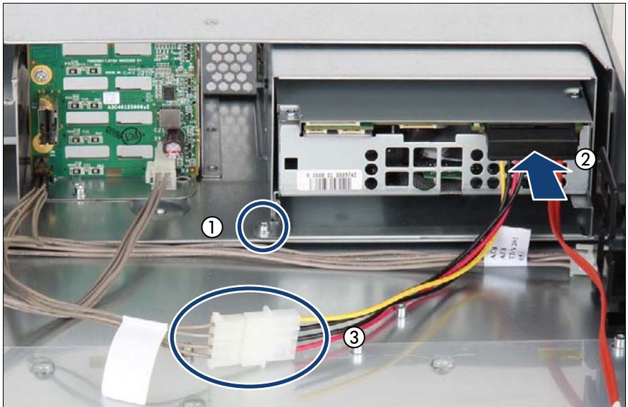
図 222: LTO4/5/6 へのケーブルの接続
