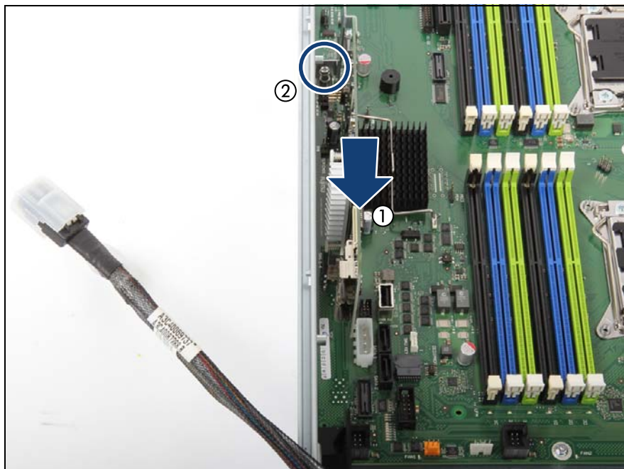
図 92: SAS RAID コントローラの取り付け
