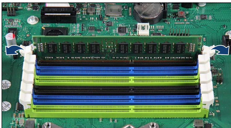
図 140: メモリモジュールの取り外し (A)
