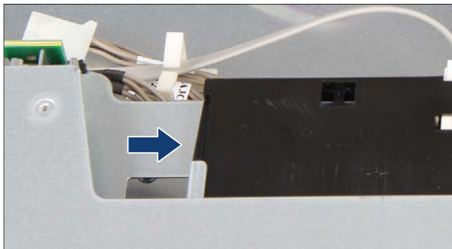
図 179: LSD モジュールのロック解除
