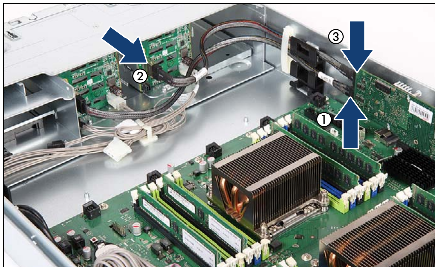
図 310: SAS ケーブルの接続
