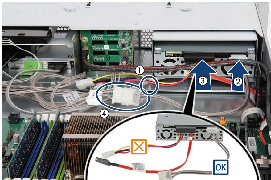
図 223: LTO3 へのケーブルの接続
