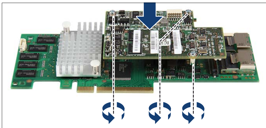
図 114: TFM キットの取り付け (A)
