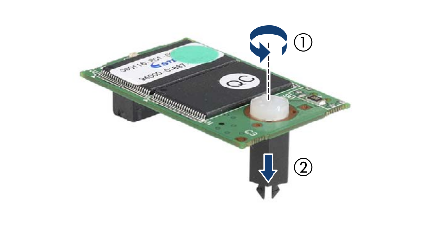
図 275: 新しい UFM の準備
