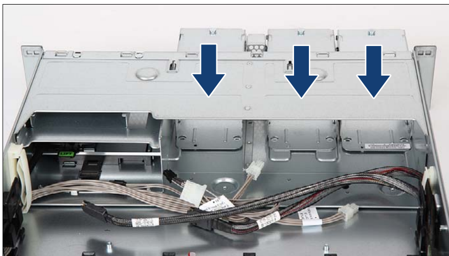
図 332: HDD ケージの取り付け
