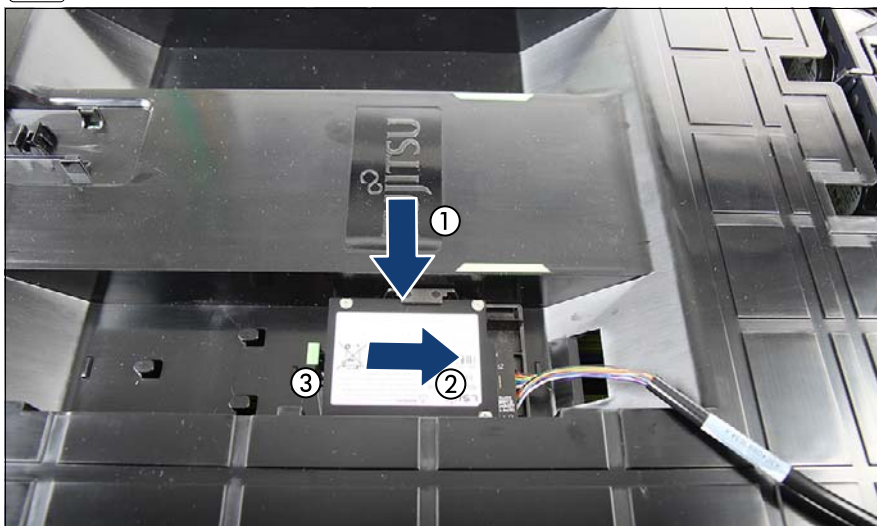
図 105: BBU ホルダーの取り付け (B)
