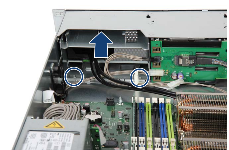
図 264: フロントパネルケースの取り外し
