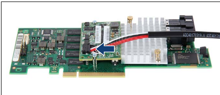
図 122: TFM の取り付け (C)
