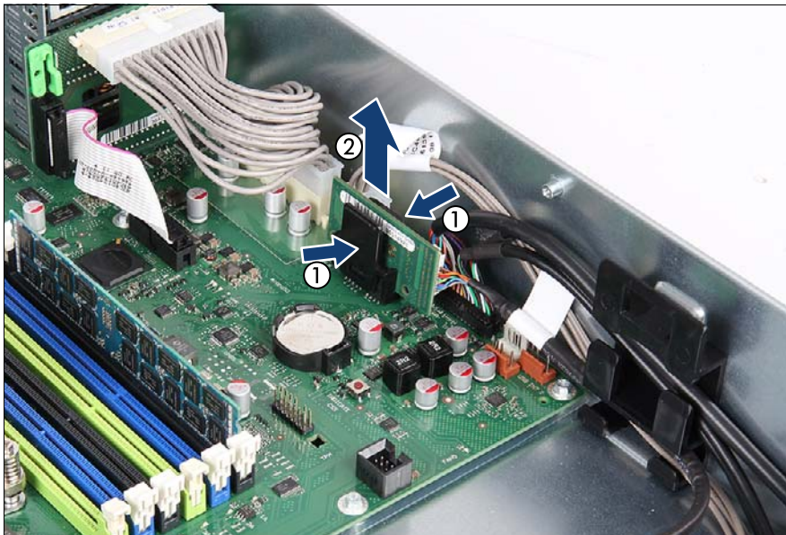
図 235: フロントパネルモジュールのケーブルの取り外し
