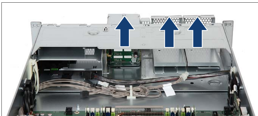
図 311: HDD ケージと 2.5 インチダミーケージの取り外し
