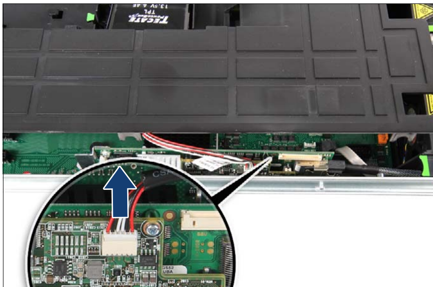
図 123: FBU ケーブルの取り外し
