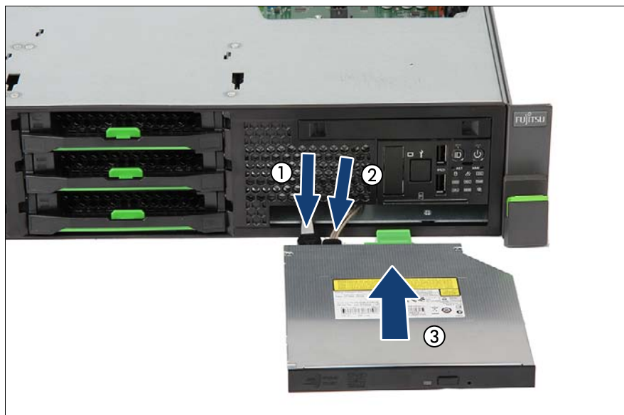
図 186: ODD の取り付け
