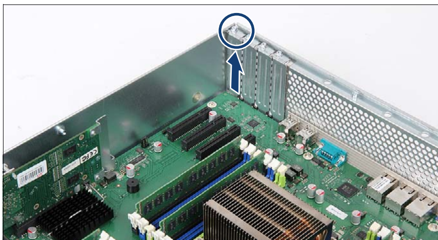
図 86: スロットブラケットの取り外し (B)
