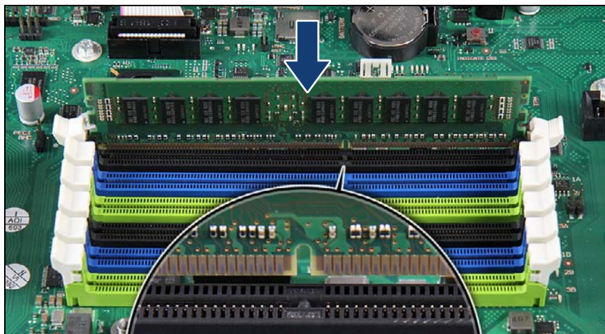
図 138: メモリモジュールの取り付け (B)
