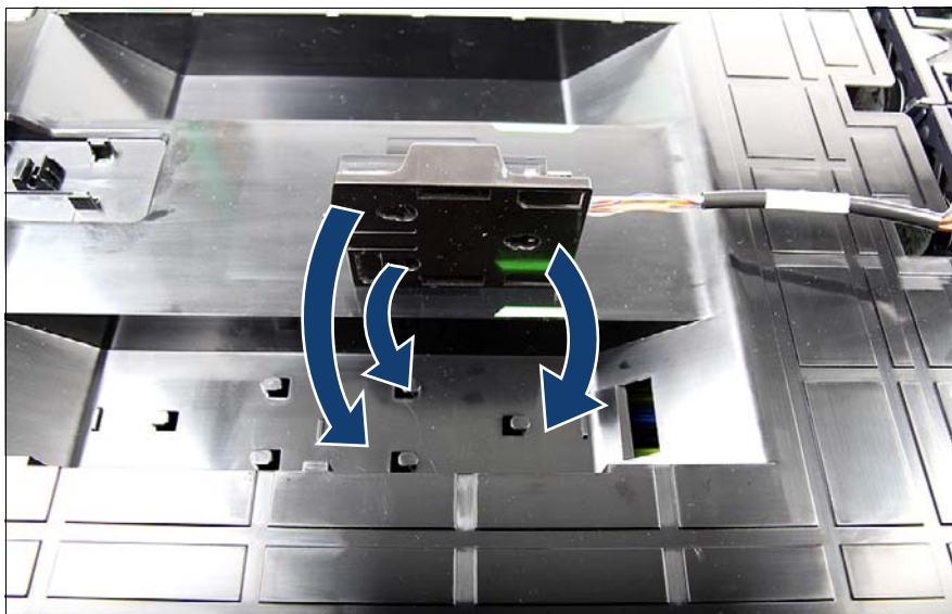
図 104: BBU ホルダーの取り付け (A)
