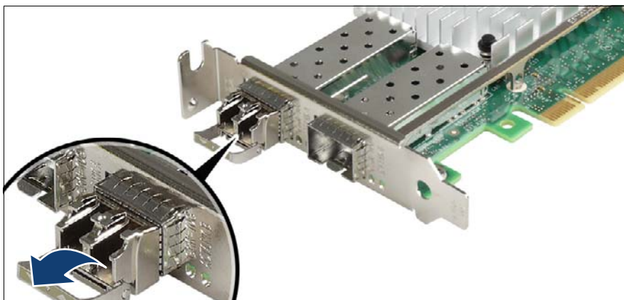
図 134: ロッキングハンドルのラッチ解除
