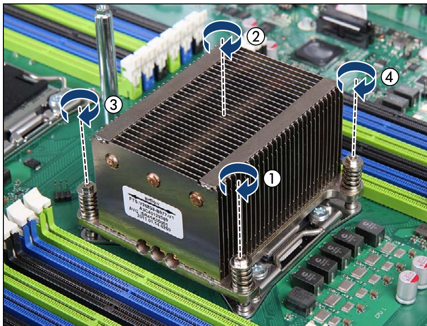
図 166: ヒートシンクを取り付ける (B)
