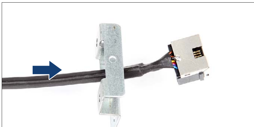
図 261: 前面 LAN ケーブルの取り外し
