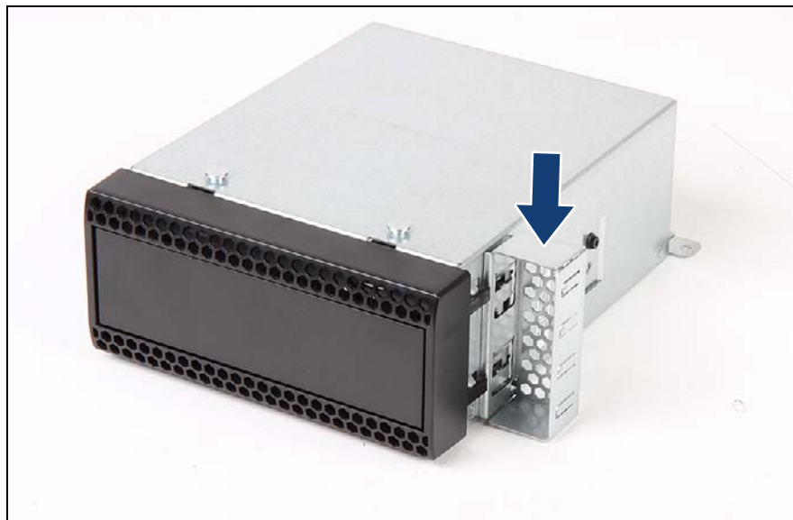
図 232: カバープレートの取り付け
