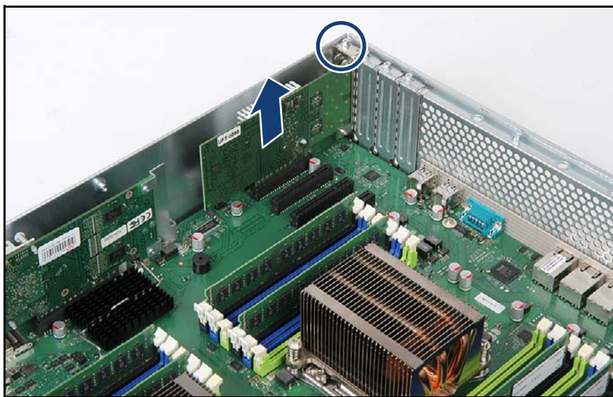
図 89: 拡張カードの取り外し (A)
