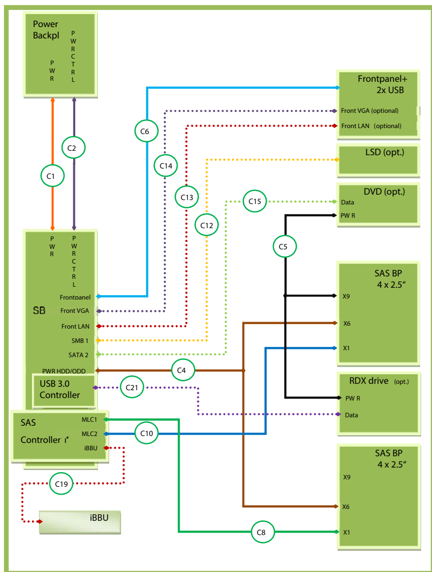
図 344: RDX ドライブ搭載 8x 2.5 インチ HDD モデルの USB 3.0 インタフェースカードによるケーブル配線
