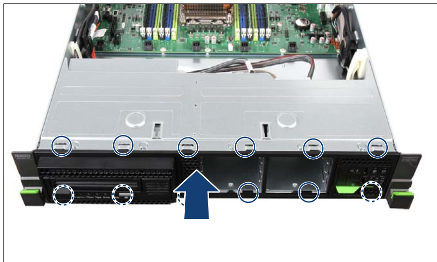
図 305: 小型フロントパネルケーシング付き構成でのフロントカバーの取り付け
