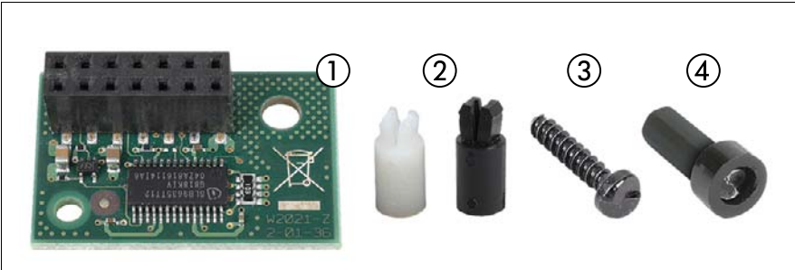
図 278: TPM キット
