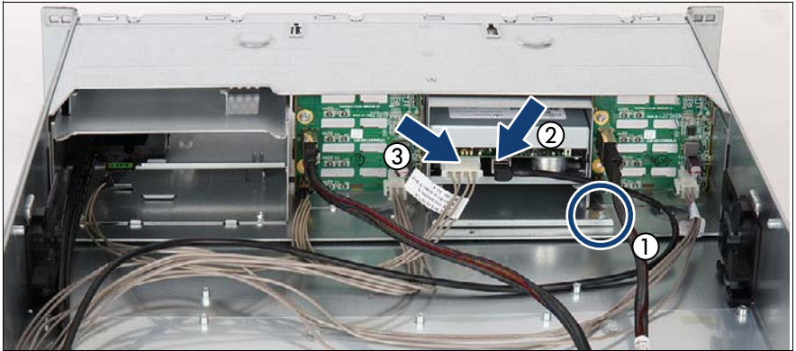
図 210: ケーブルのテープ /RDX ドライブからの取り外し
