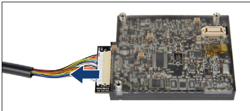
図 110: BBU からの BBU ケーブルの取り外し
