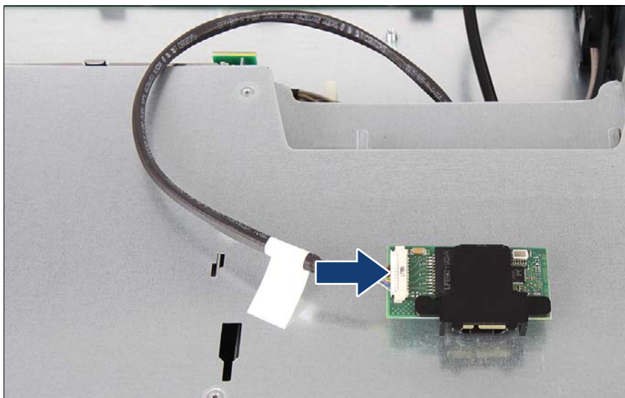
図 254: 前面 LAN ボードに前面 LAN ケーブルの接続
