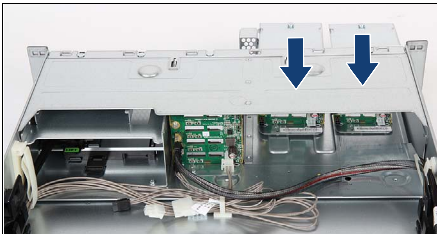
図 325: HDD ケージの取り付け
