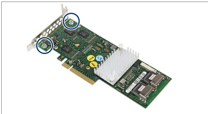
図 74: 標準スロットブラケットの取り付け (B)
