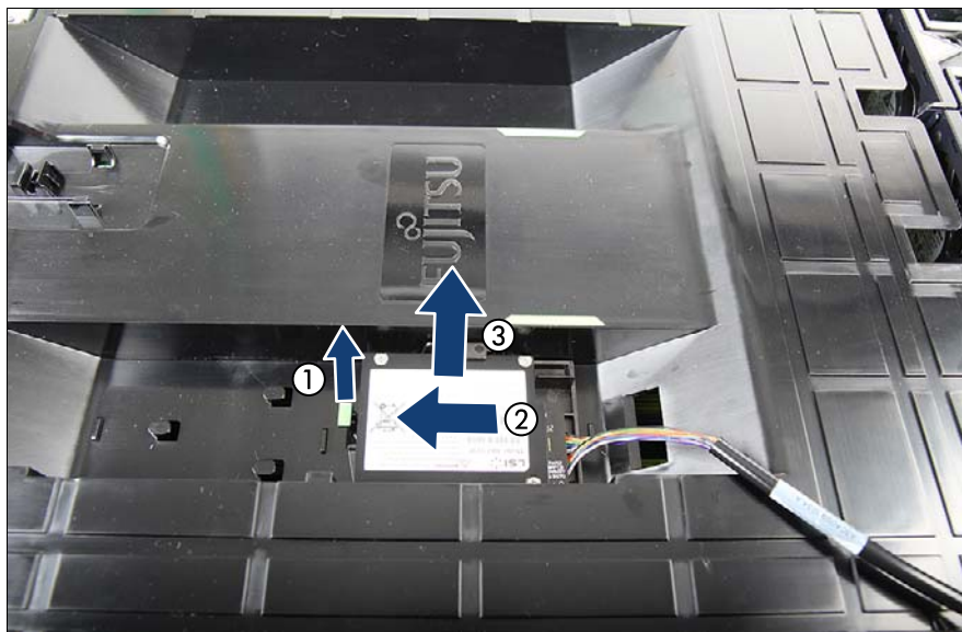
図 108: 送風ダクトからの BBU ホルダーの取り外し (A)
