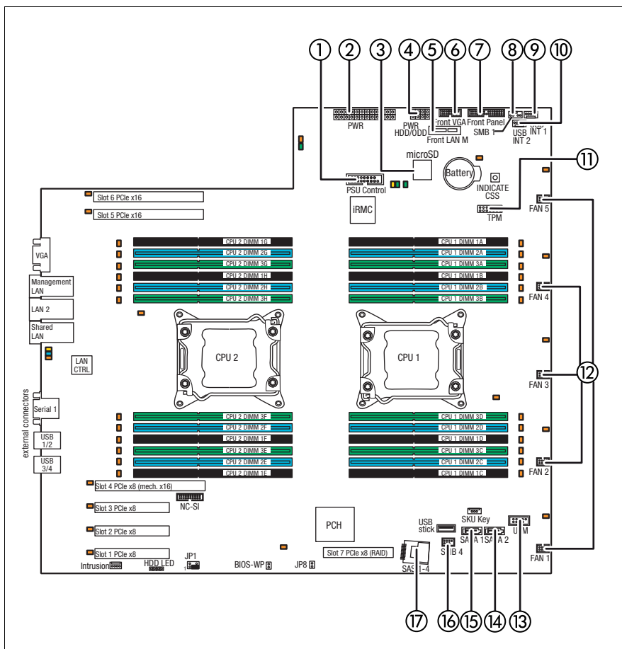
図 359: システムボード D2939 の内部コネクタ
