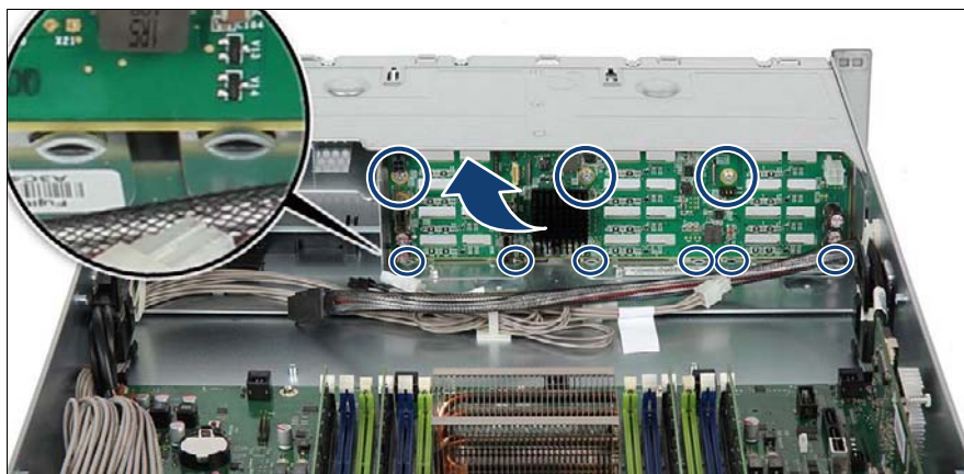
図 63: 12x 2.5 インチ HDD SAS バックプレーンの取り付け (A)
