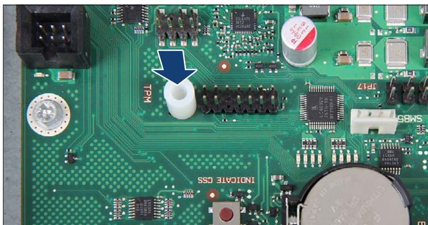
図 280: TPM スペーサーの取り付け
