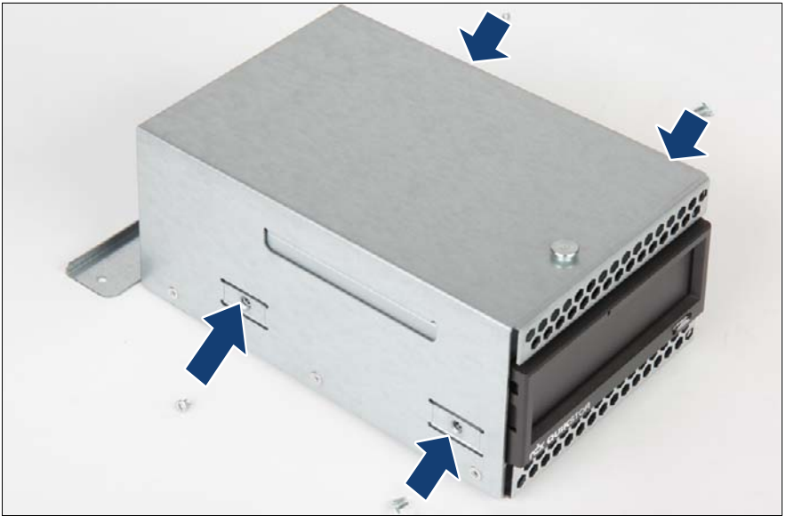
図 204: テープ/RDX ドライブのドライブケースへの固定
