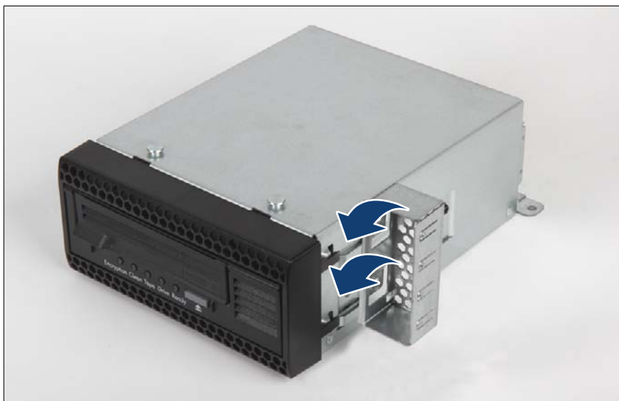
図 220: カバープレートの接続
