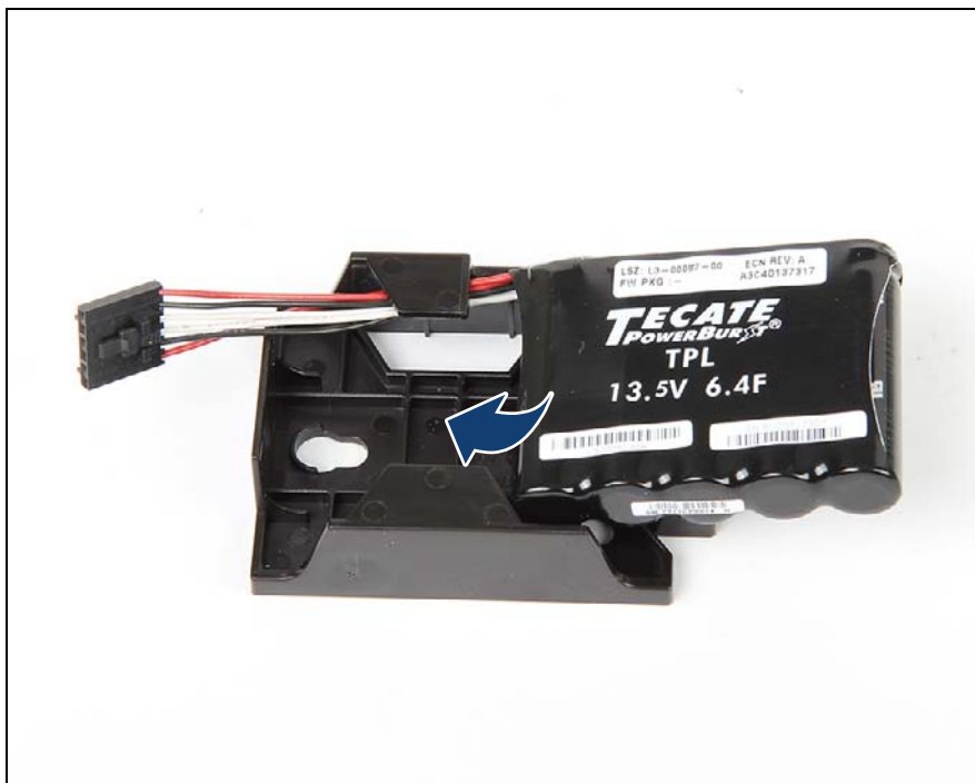
図 111: FBU ホルダーへの FBU の取り付け (A)
