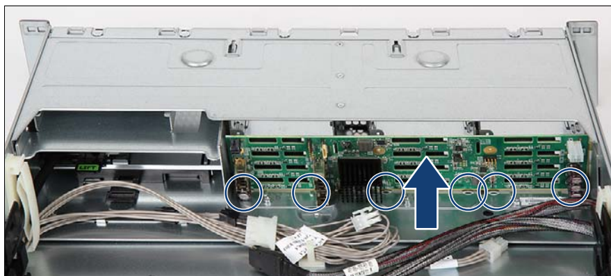
図 315: 12x 2.5 インチ HDD バックプレーンの取り付け
