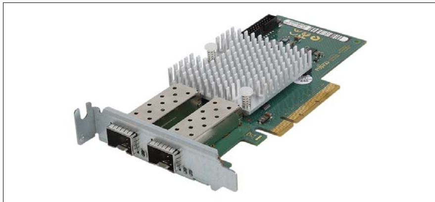
図 83: ネットワークアダプタ D2755 - スロットブラケットの取り付け (C)
