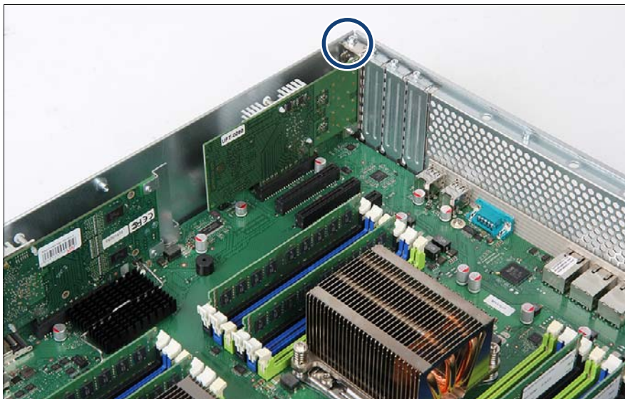
図 88: 拡張カードの取り付け (B)
