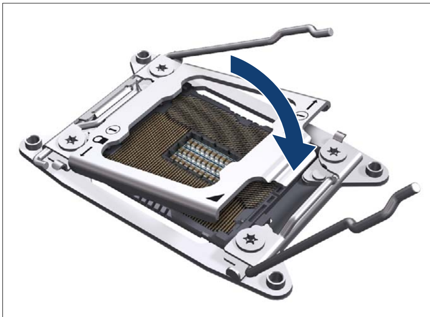
図 157: ロードプレートを閉じる
