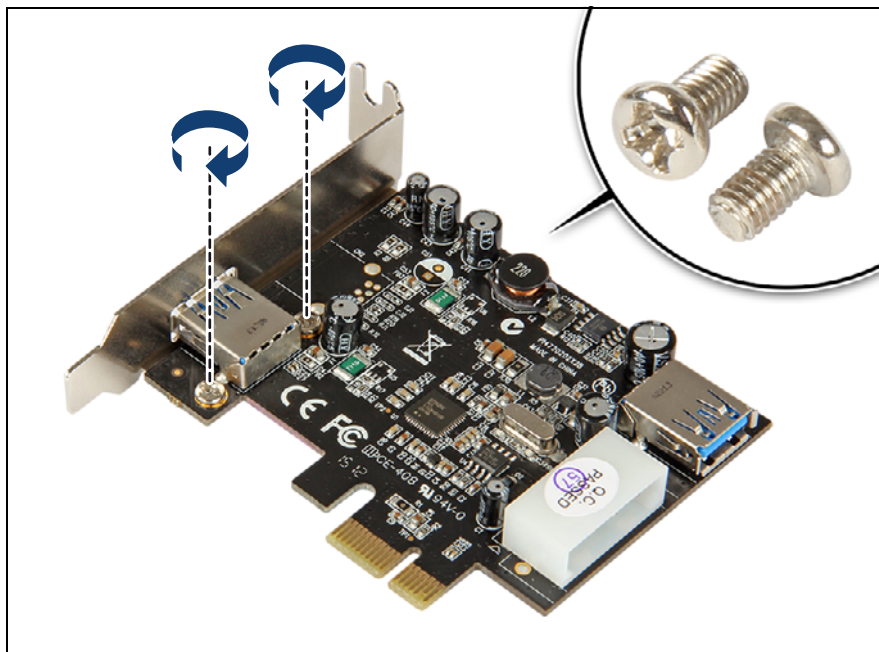
図 85: PCI スロットブラケットの取り付け (B)
