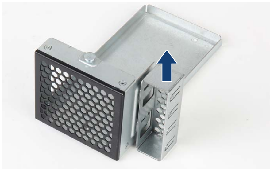
図 307: カバープレートの 2.5 インチダミーケースからの取り外し
