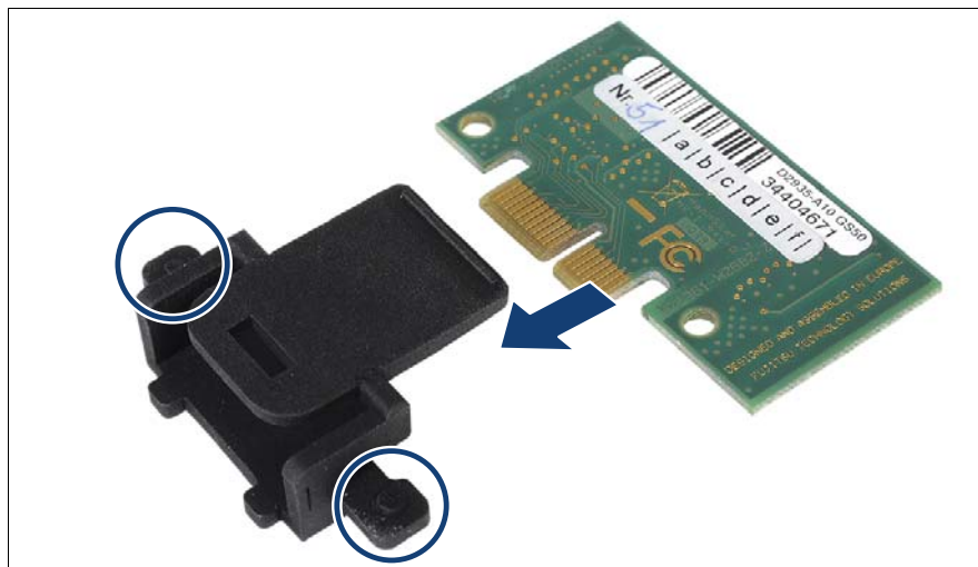
図 253: 前面 LAN ボードの組み立て (A)
