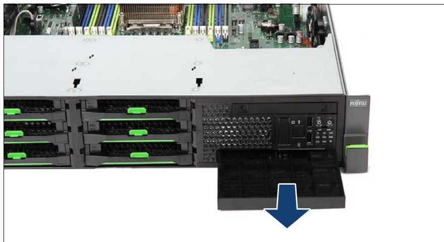
図 183: ダミーモジュールの取り外し
