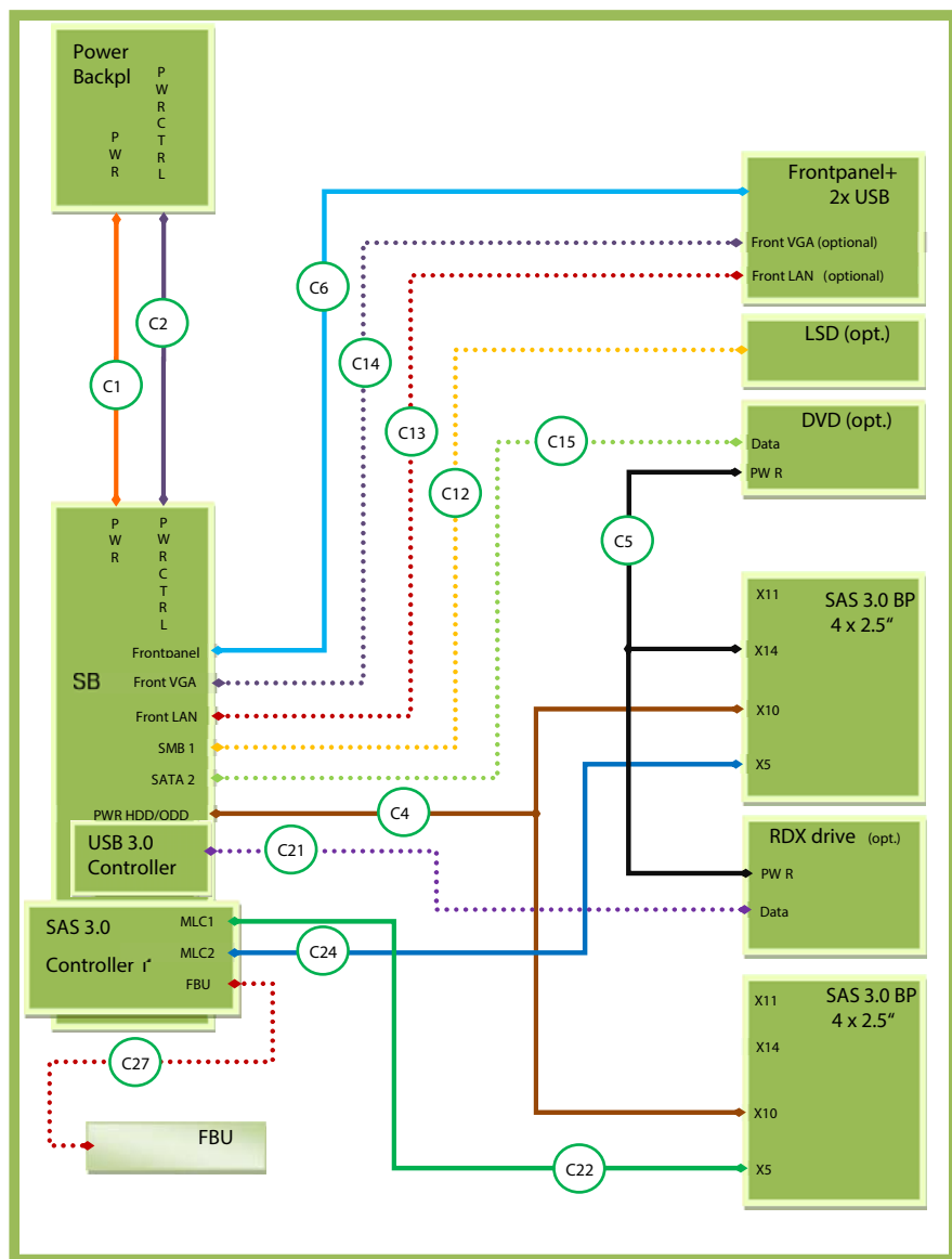
図 351: ケーブル配線 - 8x 2.5 インチ SAS 3.0 HDD モデル + RDX (USB3.0) モデル
