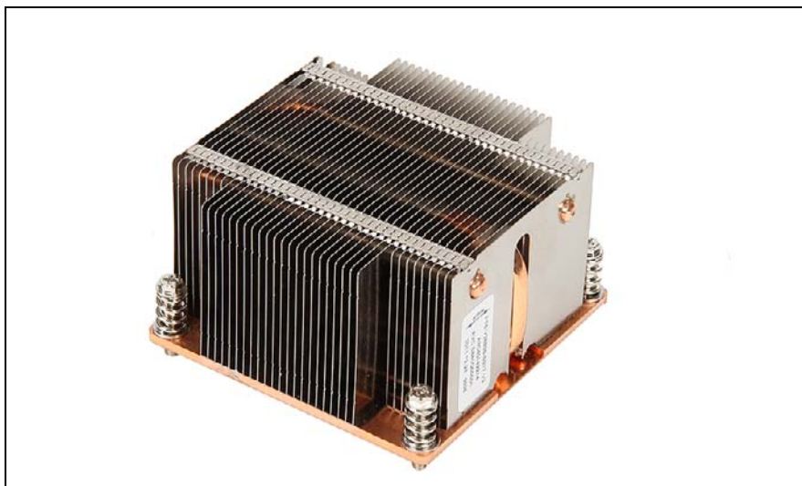
図 163: ハイパフォーマンスプロセッサヒートシンク V26898-B977-V3
