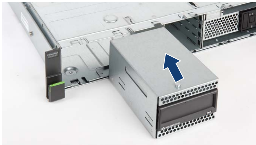
図 205: テープ/RDX ドライブの取り付け
