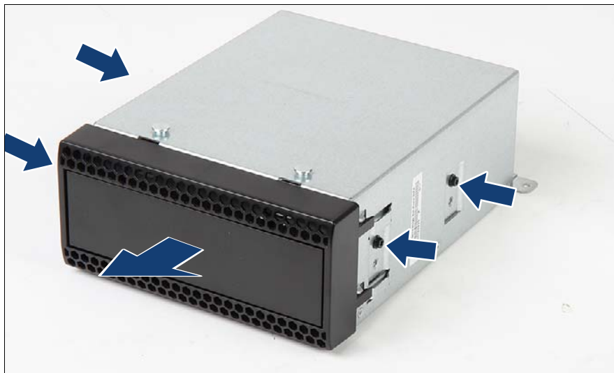
図 217: テープドライブのダミーモジュールの取り外し
