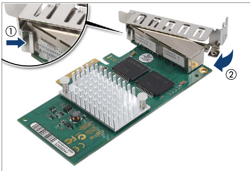
図 78: ネットワークアダプタ D2745 - スロットブラケットの取り付け (A)
