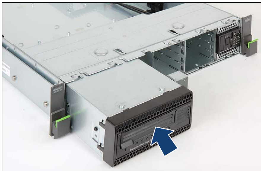
図 221: LTO ケージの挿入
