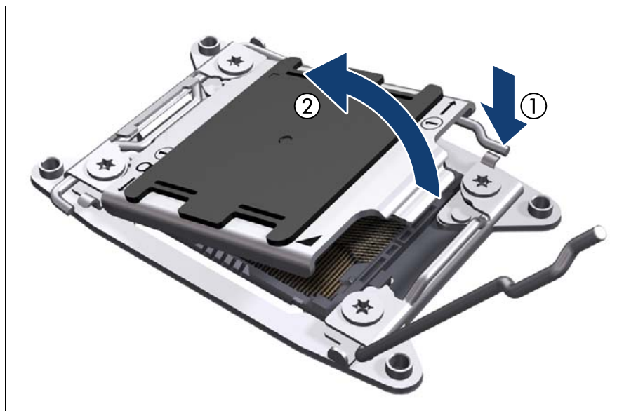
図 145: ロードプレートを開く (A)
