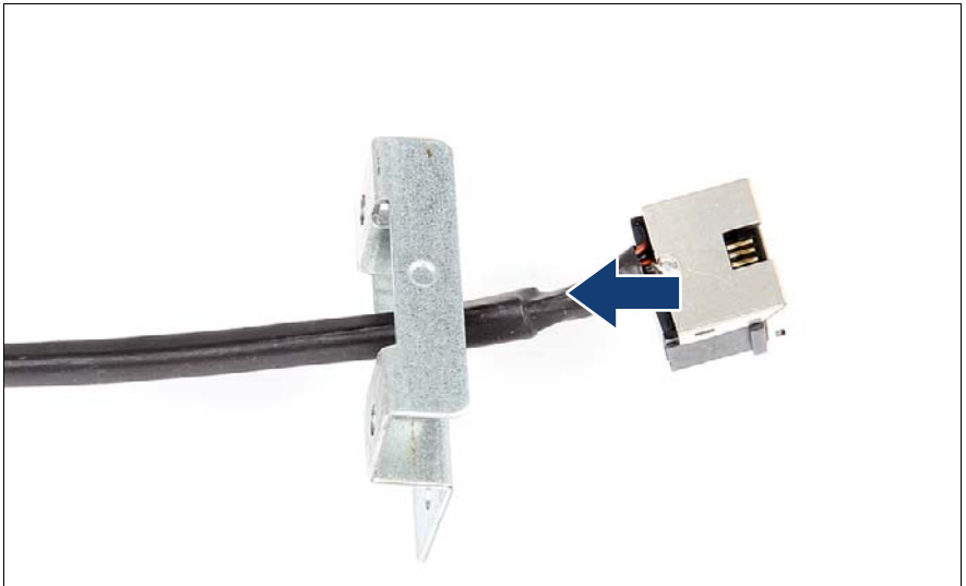
図 250: 前面 LAN コネクタの取り付け
