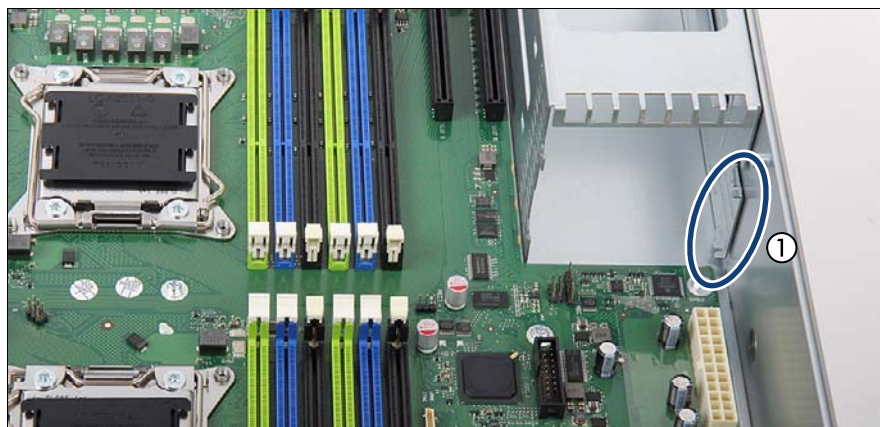
図 27: パワーバックプレーンの取り付け (A)
