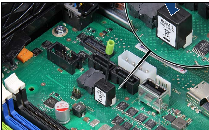
図 289: オンボード SAS 有効化キーの取り付け位置
