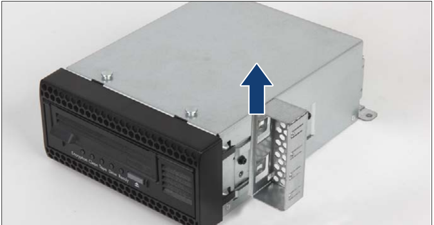
図 227: カバープレートの取り外し
