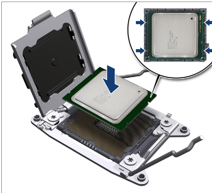
図 147: プロセッサを取り付ける
