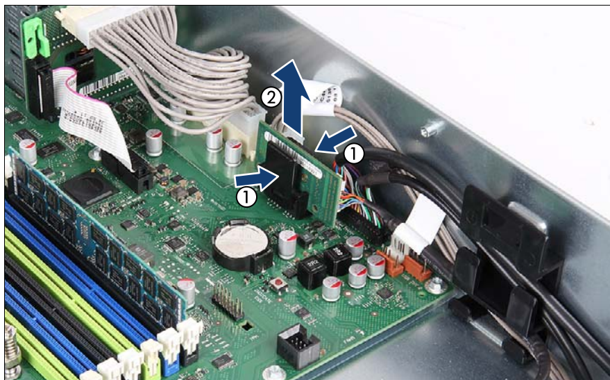
図 256: 前面 LAN ボードの取り外し
