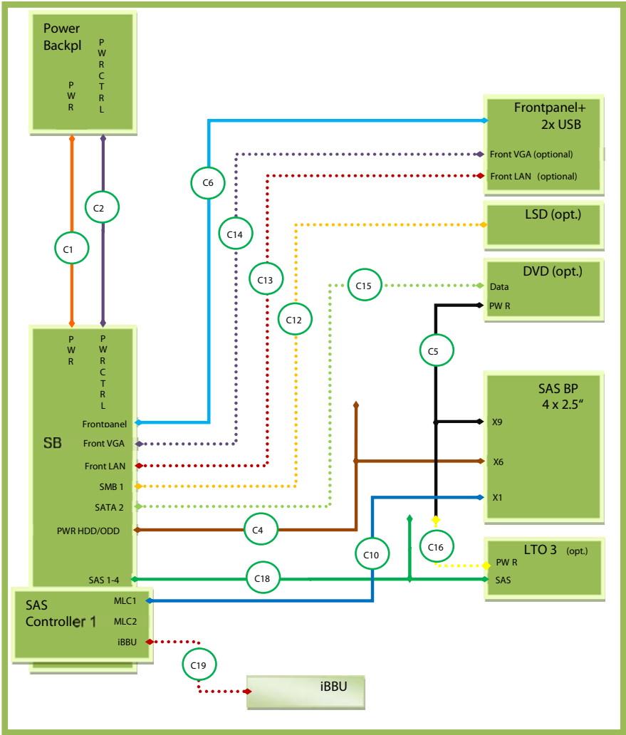
図 341: ケーブル配線 - LTO3 ドライブ搭載 4x 2.5 インチ HDD モデル
