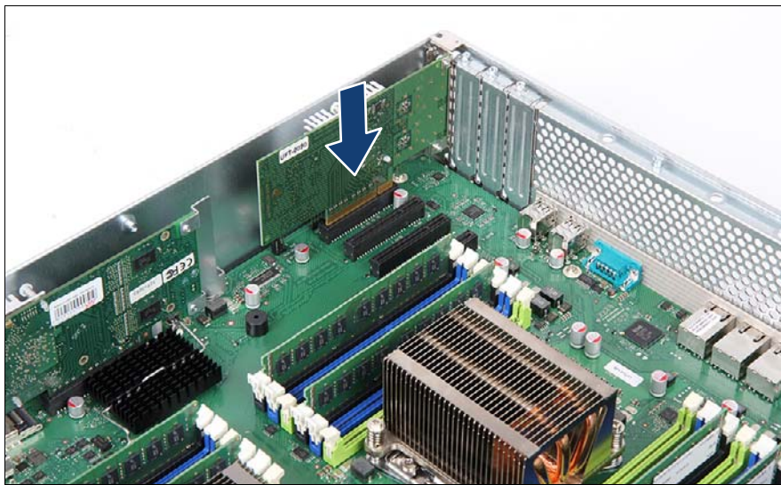
図 87: 拡張カードの取り付け (A)
