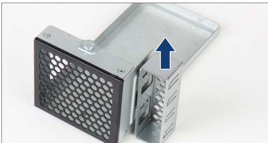
図 319: カバープレートの 2.5 インチダミーケーシングからの取り外し
