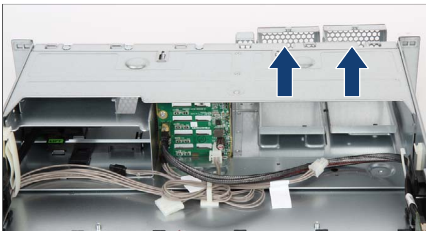
図 318: 2.5 インチダミーケーシングの取り外し
