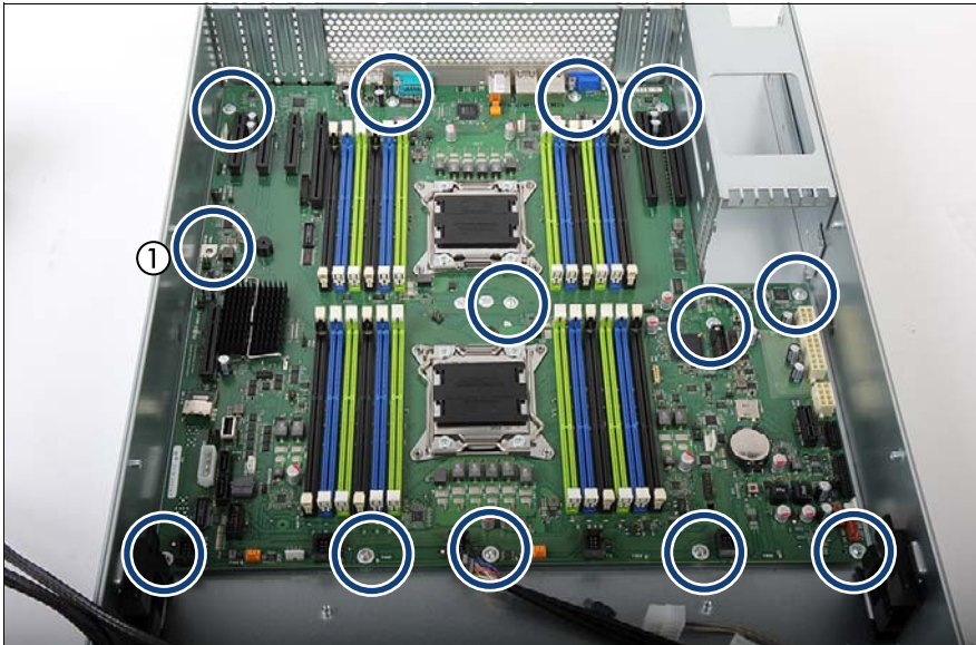
図 294: システムボードの取り外し
