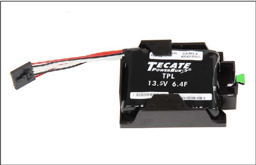
図 112: FBU を FBU ホルダーへの取り付け (B)
