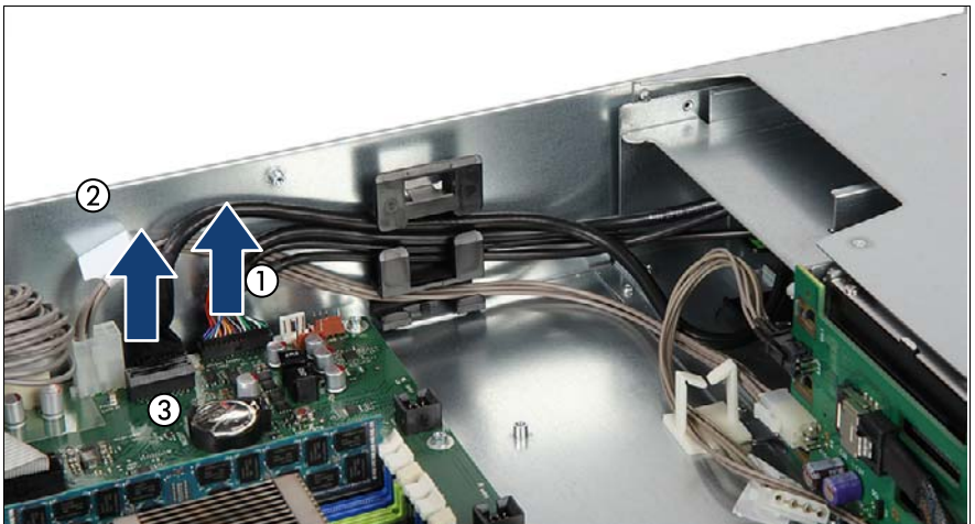
図 244: 前面の VGA ケーブルの取り外し
