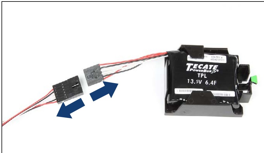
図 125: FBU からの FBU アダプタケーブルの取り外し
