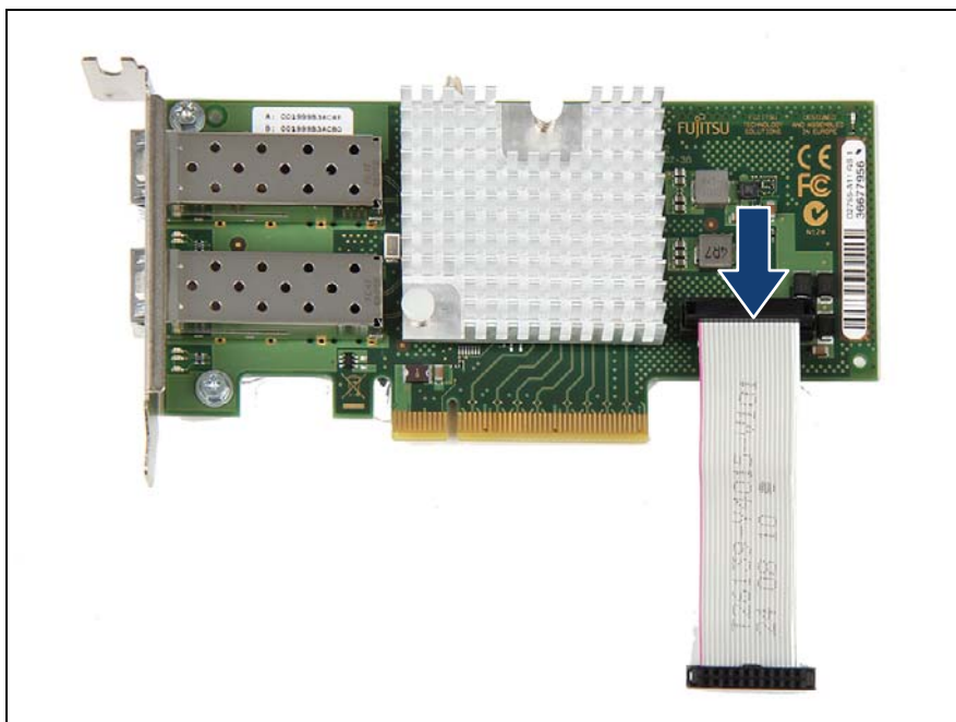
図 96: NCSI サイドバンドケーブルの接続
