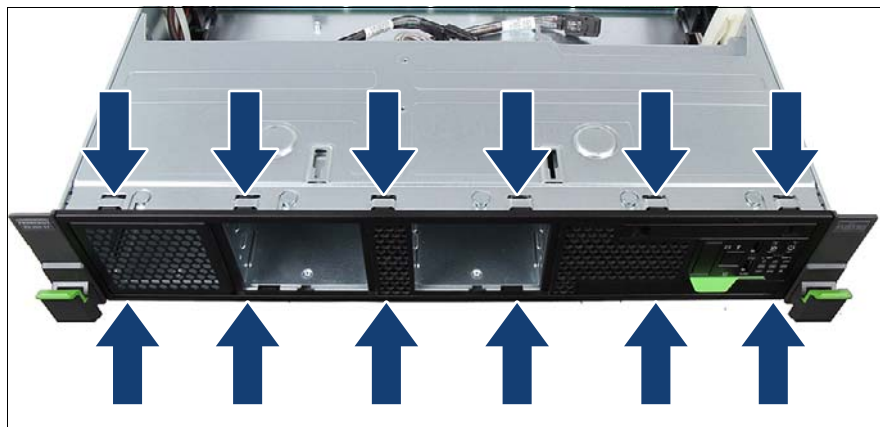
図 298: ラックフロントカバーの取り外し (A)
