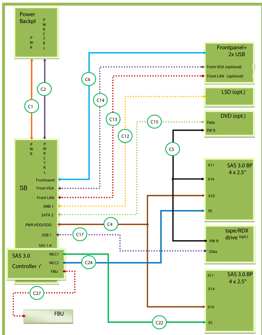
図 350: ケーブル配線 - 8x 2.5 インチ SAS 3.0 HDD モデル + DAT/RDX (USB2.0) モデル
