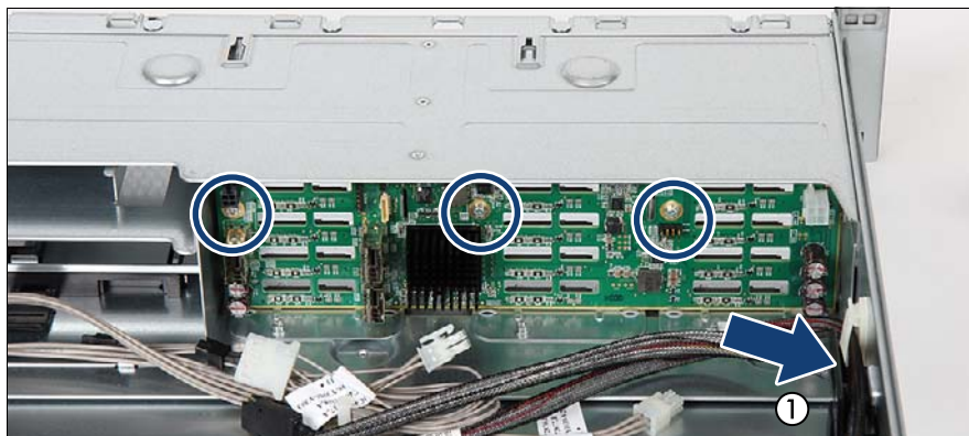
図 334: 12x 2.5 インチ HDD バックプレーンの取り付け
