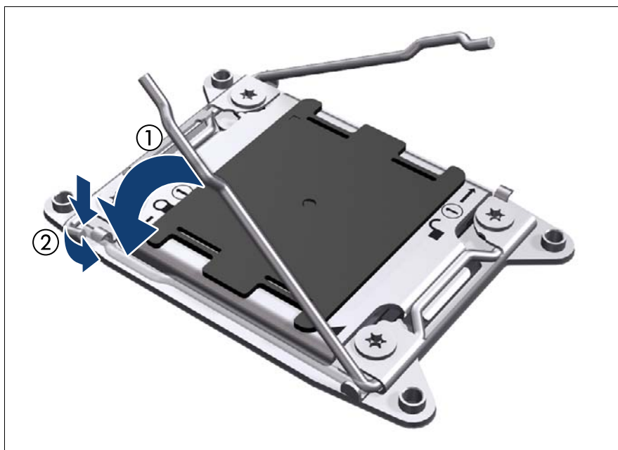
図 150: ソケットリリースレバー 2 を閉じます。
