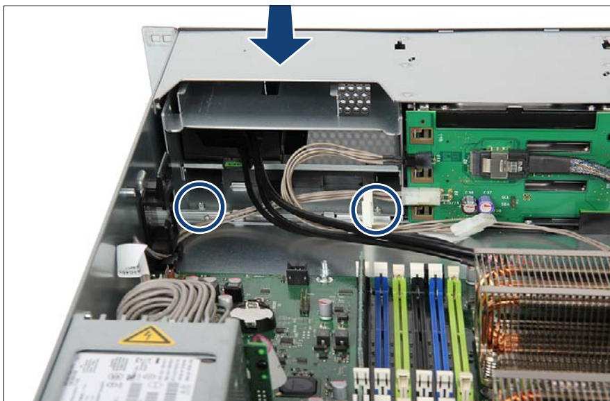
図 266: フロントパネルケージの挿入
