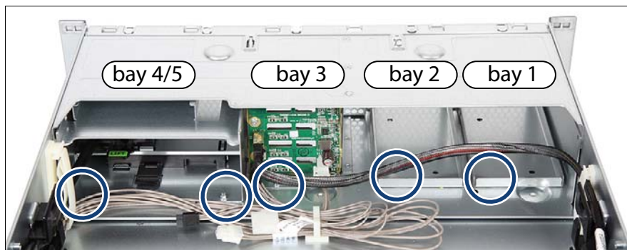
図 303: HDD ケージとフロントパネルケージの取り付け
