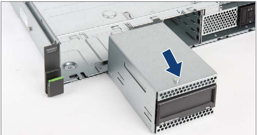
図 211: ドライブケースの解除
