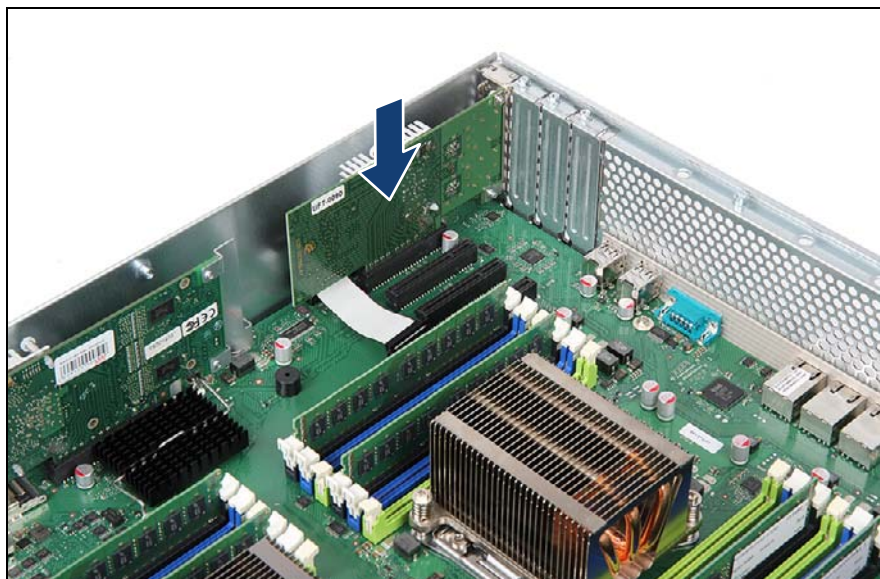
図 97: Modular LAN コントローラの取り付け
