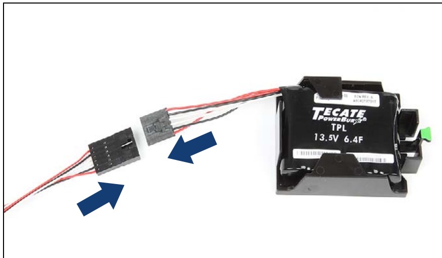
図 115: FBU への FBU アダプタケーブルの接続
