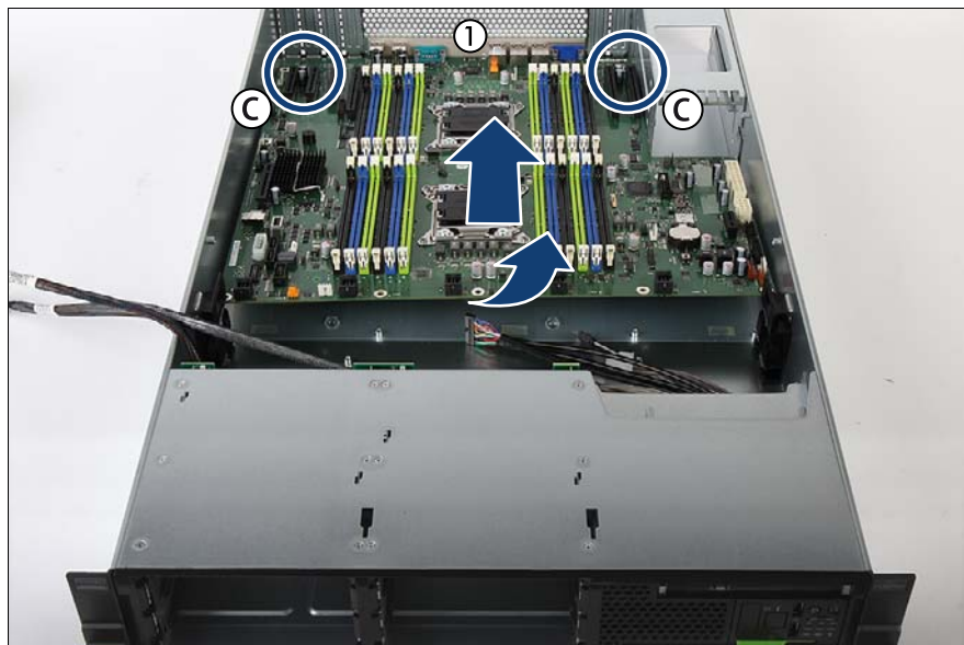
図 296: システムボードの取り付け
