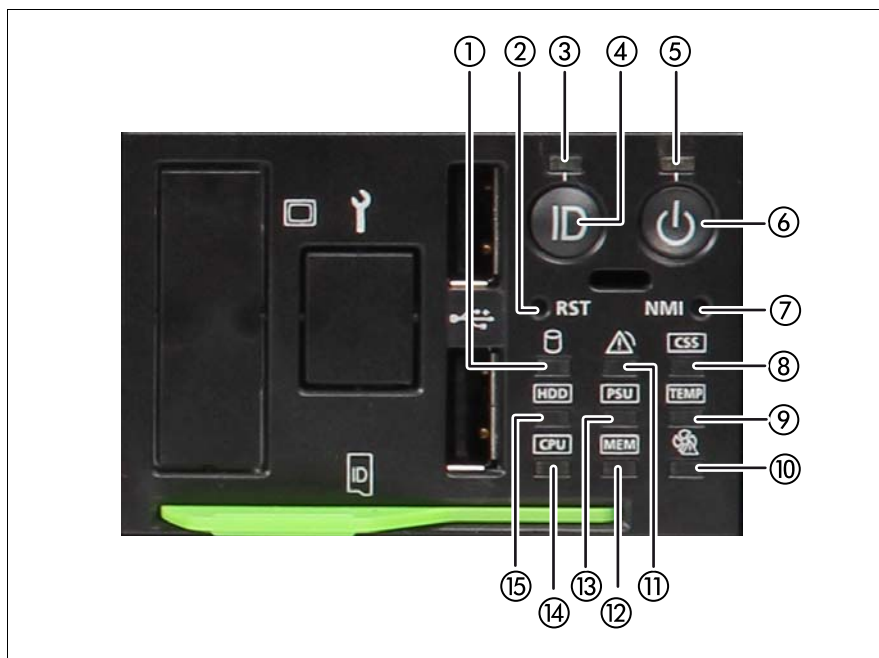
図 364: 前面 : 表示ランプとコントロール
