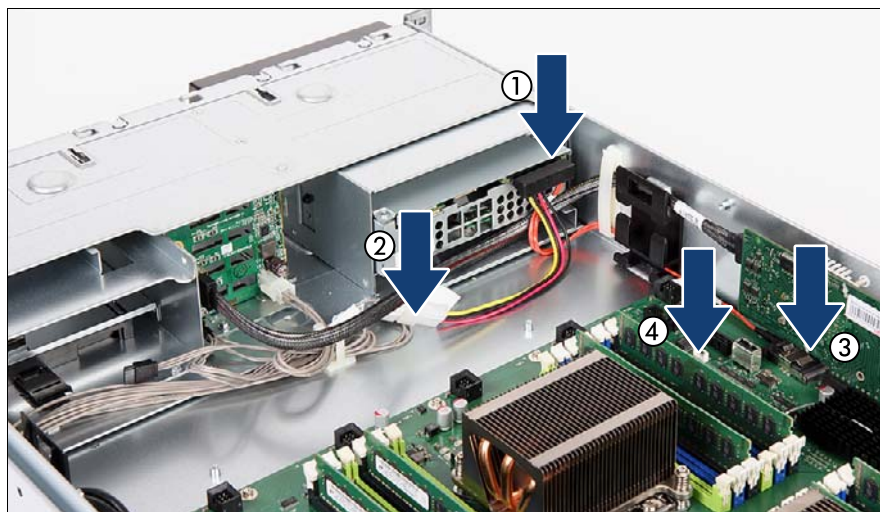
図 321: LTO ドライブケーブルの接続
