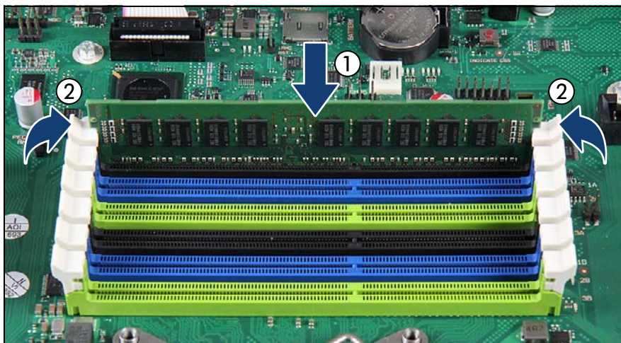
図 139: メモリモジュールの取り付け (C)
