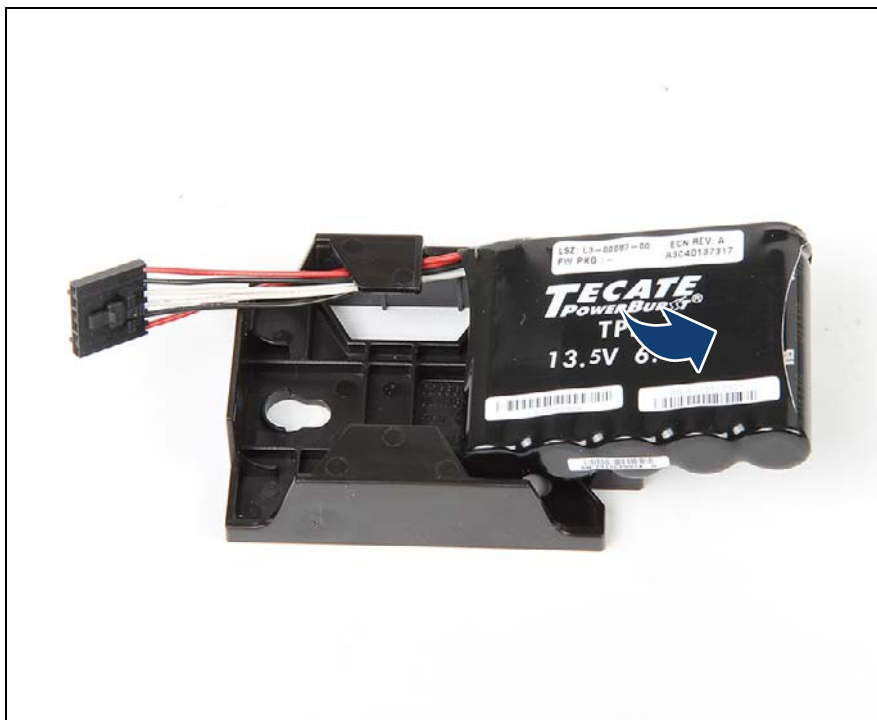
図 126: FBU をホルダーから取り外す
