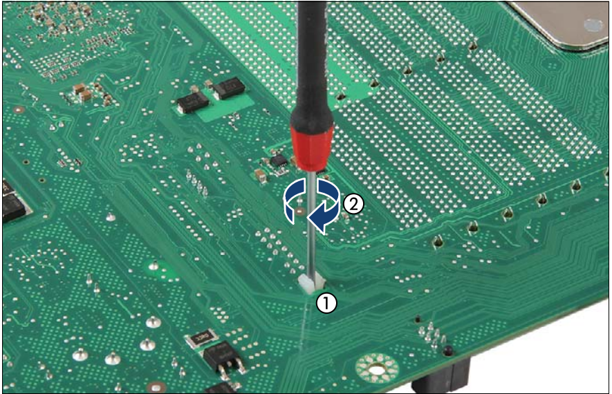
図 284: TPM 用ネジの取り外し
