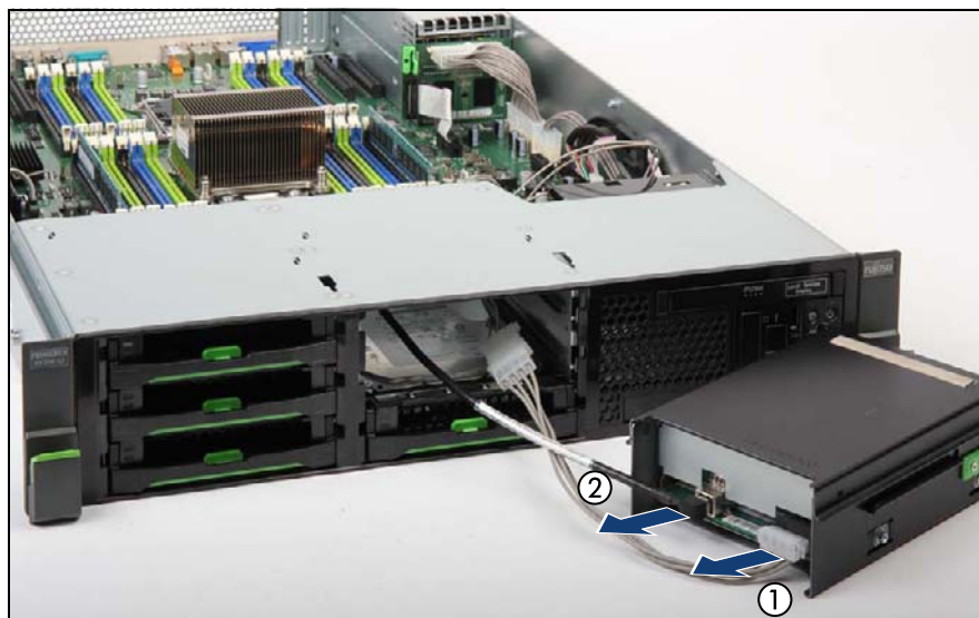
図 200: ケーブルのテープ /RDX ドライブからの取り外し
