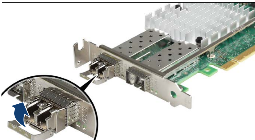
図 130: ロッキングハンドルのラッチ留め
