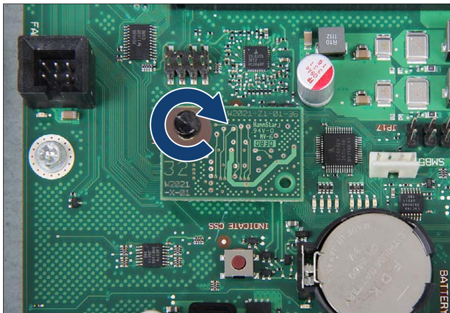
図 283: TPM の固定
