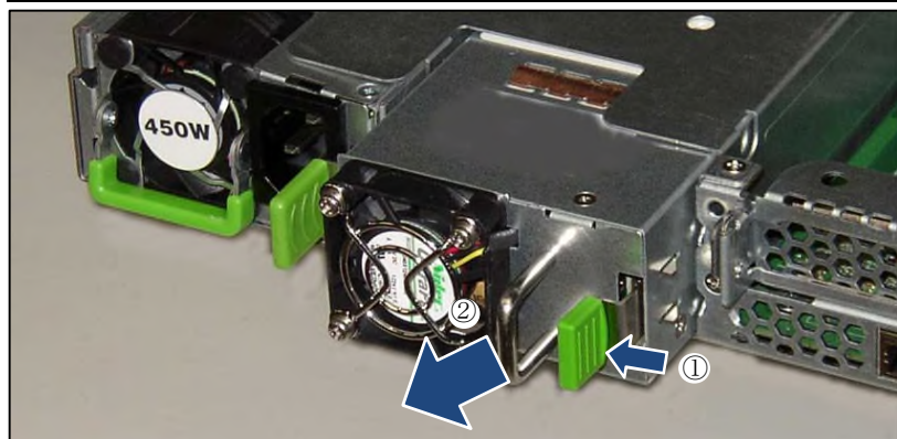
図 10 : FJBU の取り外し (RX200 S7/RX200 S8/RX100 S8)
