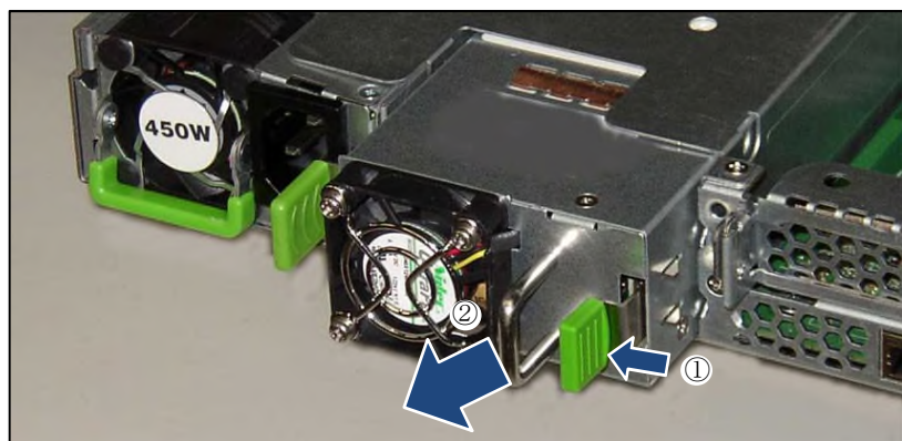
図 14 : FJBU の取り外し (RX200 S7/RX200 S8/RX100 S8)
