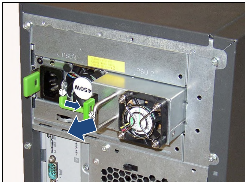
図 9 : FJBU の取り外し (TX140 S1/TX140 S2/TX150 S8)
