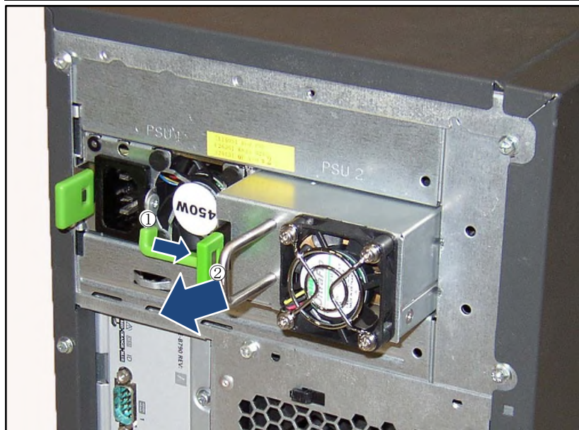
図 13 : FJBU の取り外し (TX140 S1/TX140 S2/TX150 S8)
