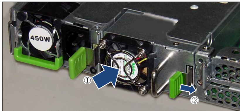
図 12 : FJBU の取り付け (RX200 S7/RX200 S8/RX100 S8)
