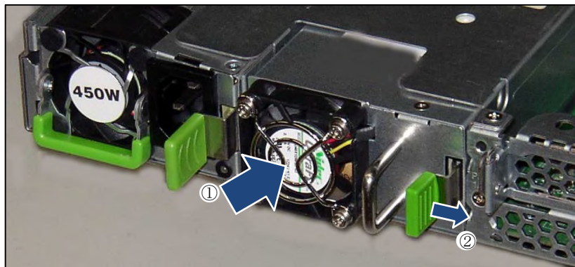
図 8 : FJBU の取り付け (RX200 S7/RX200 S8/RX100 S8)
