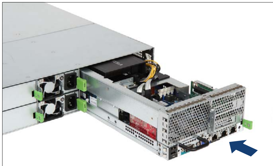
図 3: サーバノードの取り付け
