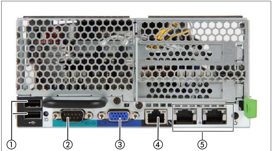
図 4: サーバノードの接続パネル
