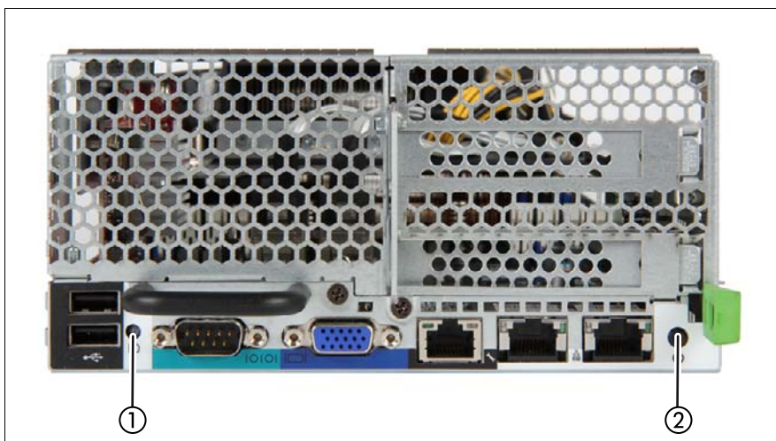
図 5: サーバノードの制御と表示ランプ
