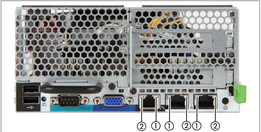
図 6: LAN 表示ランプ
