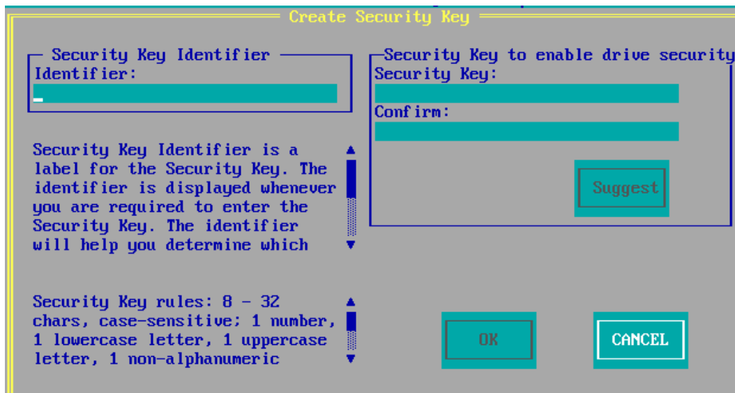
図 14 Enable Security (24.7.0-0061)
