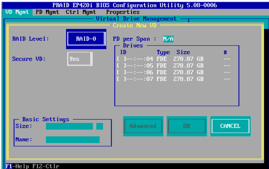
図 13 Create VD (24.7.0-0061)
