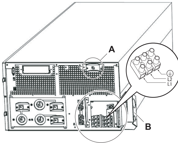
図 2：UPS 入力端子配置
