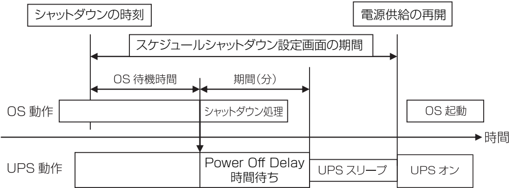
シャットダウンシーケンス
