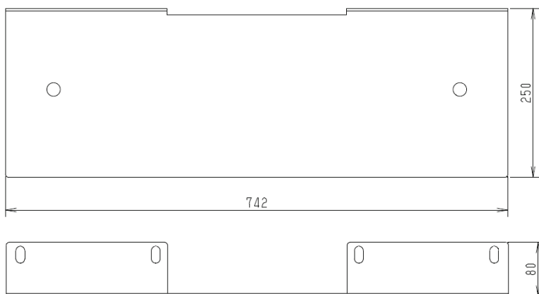
後面用パーツ
