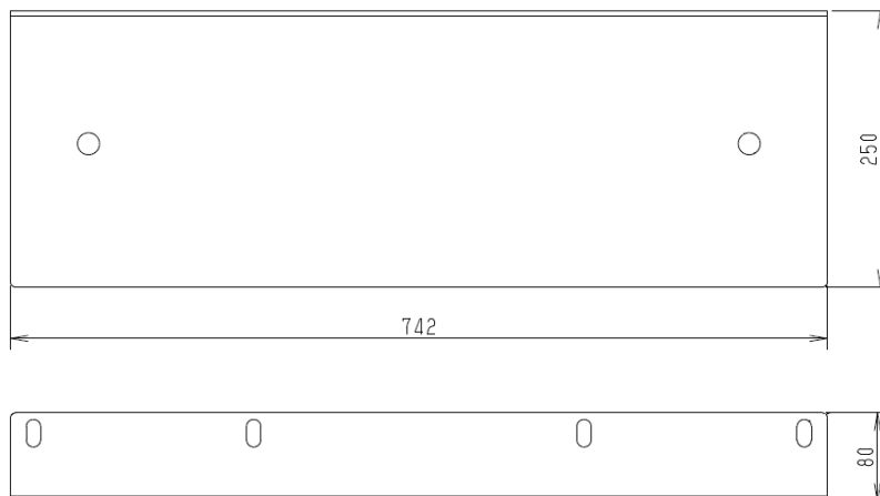
前面用パーツ
