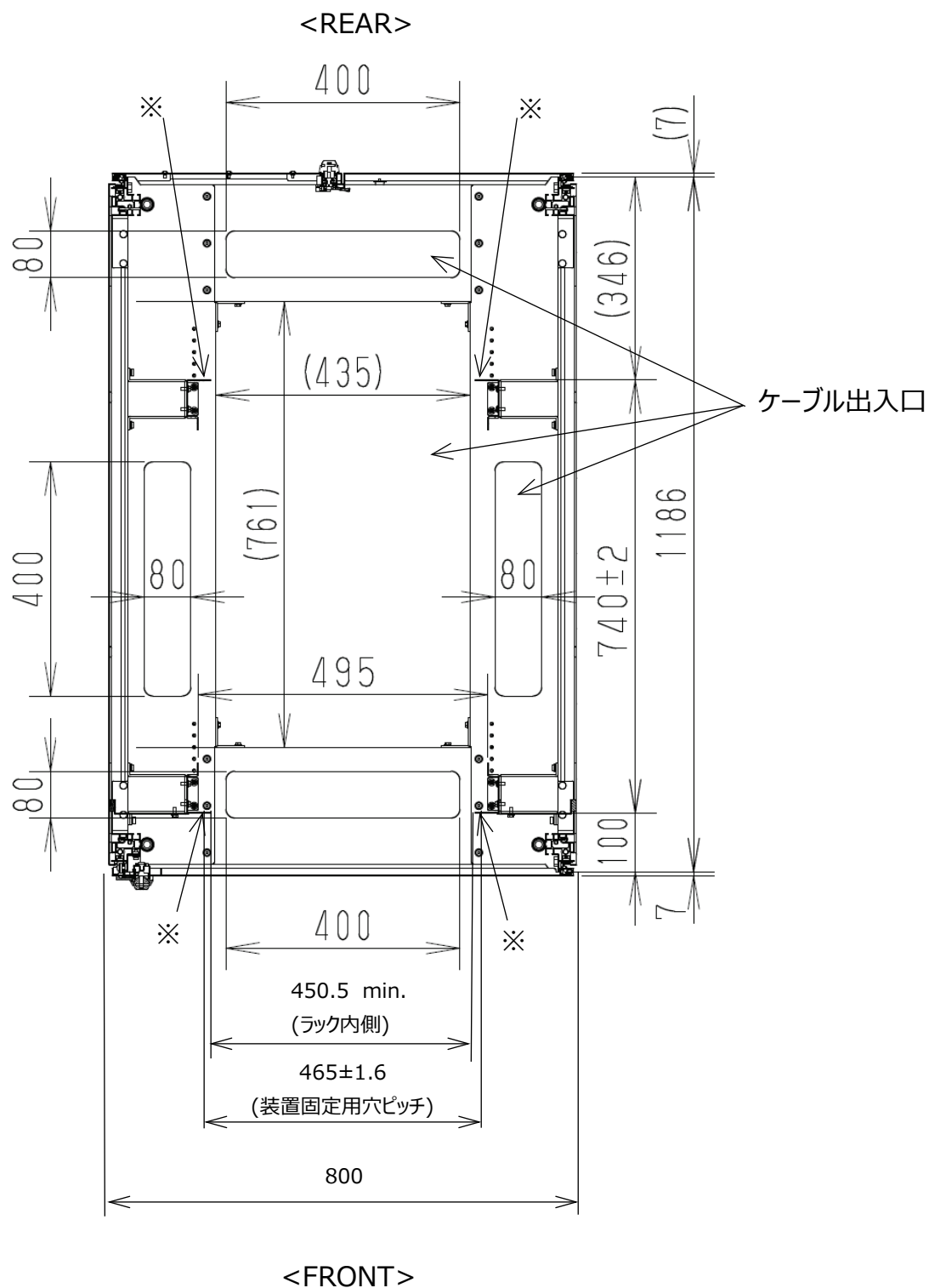
図 4: ラック内部の柱関係寸法図
