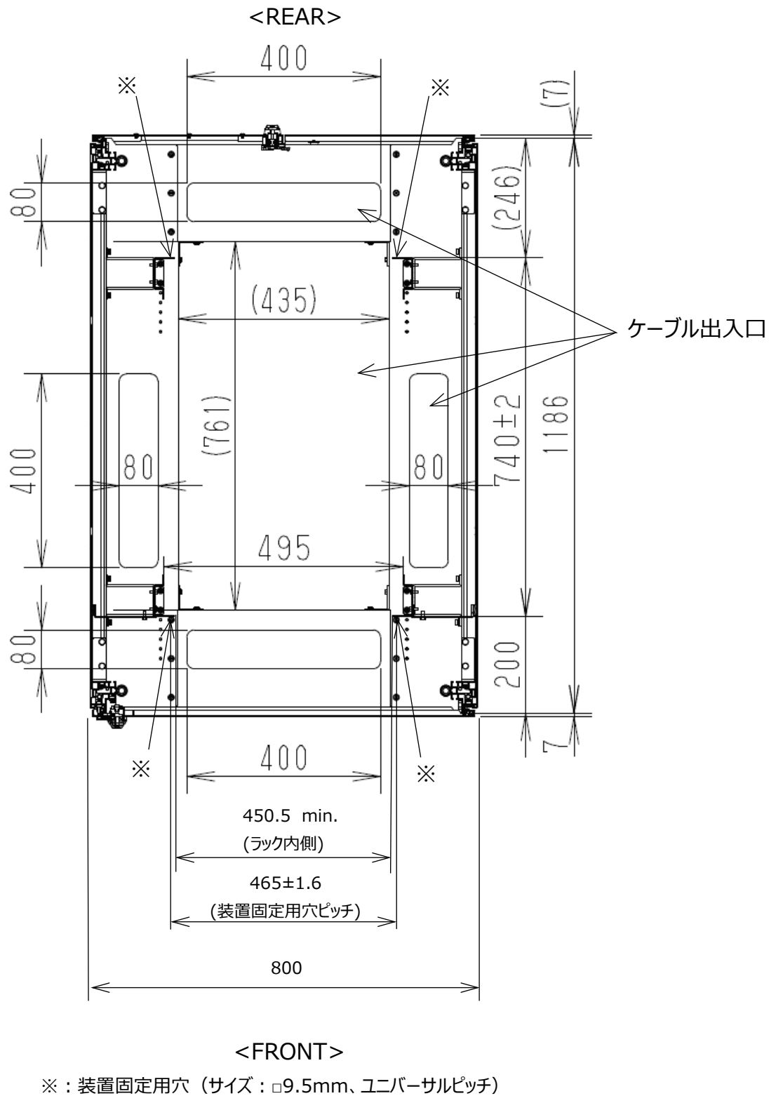
図 3: ラック内部の柱関係寸法図
