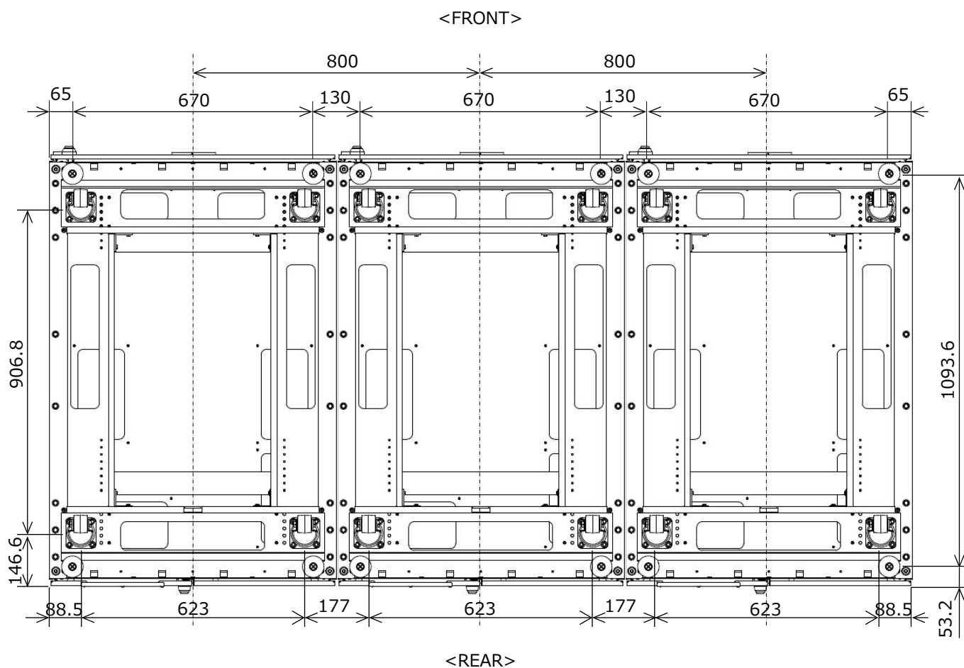
図 2: 床面寸法図
