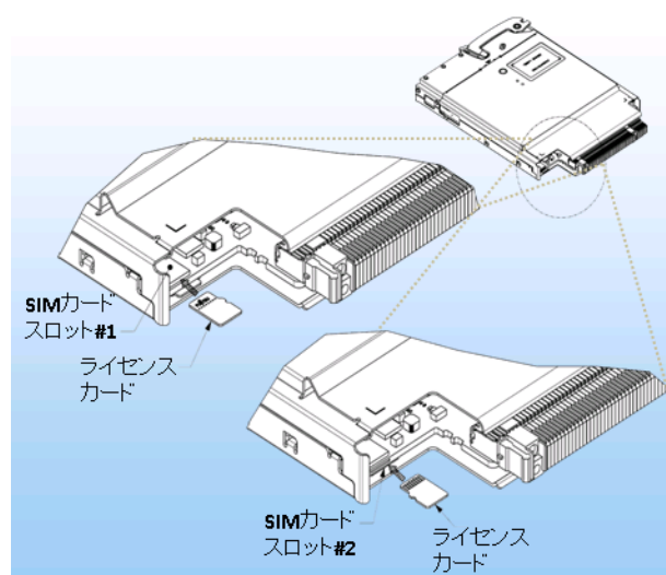
PRIMERGY コンバージドファブリックスイッチブレード (10Gbps 18/8+2)への搭載
