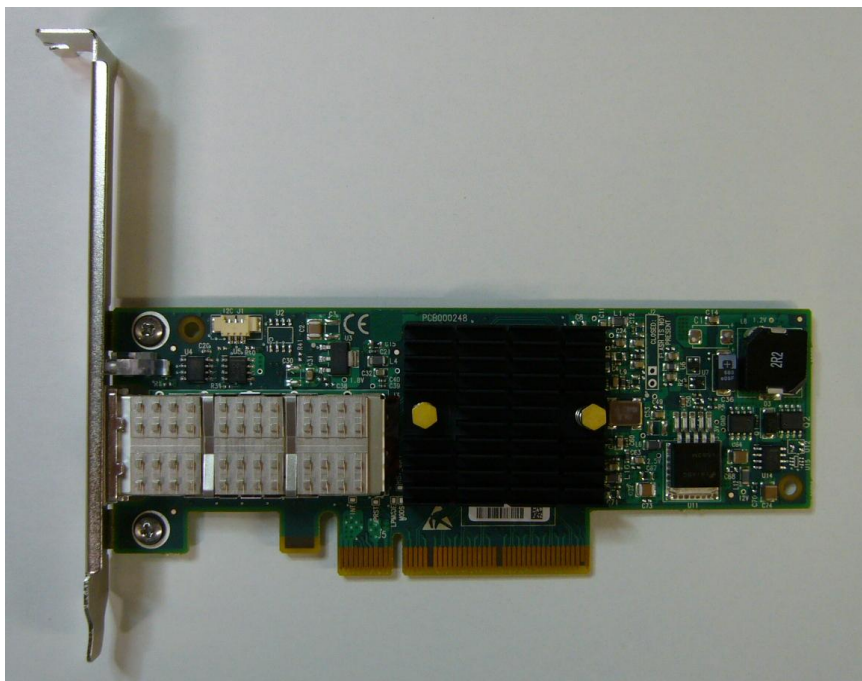
部品面(Full Heightブラケット)
