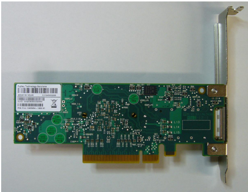
半田面 (Full Height ブラケット)
