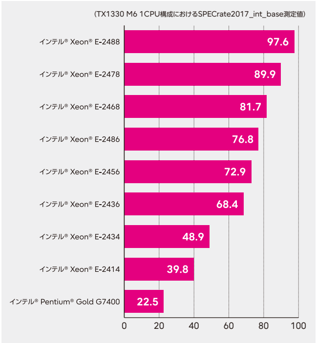
CPU別性能比較グラフ (1Way)
