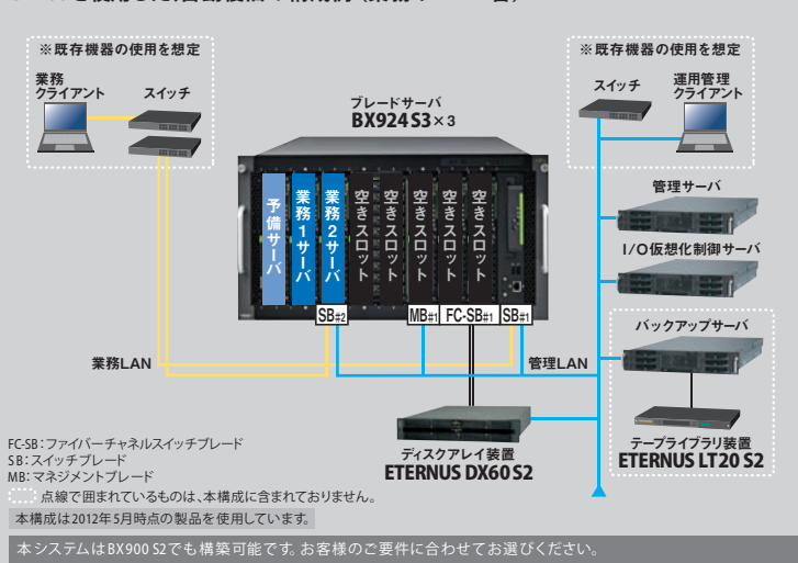
BX400を使用した、自動復旧の構成例 (業務サーバ2台)
