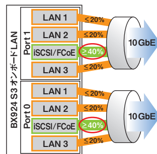
10G LAN コネクションブレード接続時 (UMC 機能設定例)
