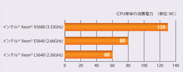
CPU別電力消費比較グラフ
