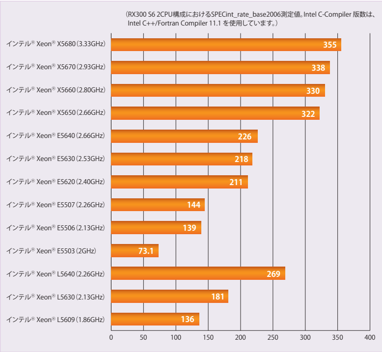
CPU別性能比較グラフ
