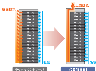
排気方式の比較
