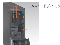
SAS/HDDディスク4台搭載時
