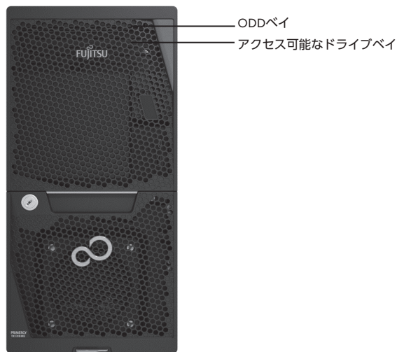
[タワーベースユニット (3.5インチ HDD/SSD×4/250W電源×1、Board Management Controller対応)]
