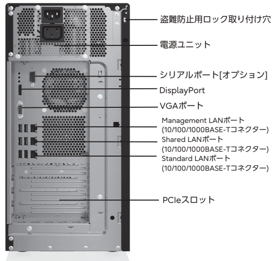
[タワーベースユニット (3.5インチ HDD/SSD×4/250W電源×1、Board Management Controller対応)]
