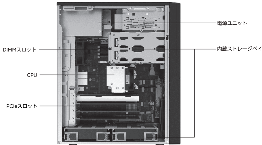
【サーバ本体前面】 →
