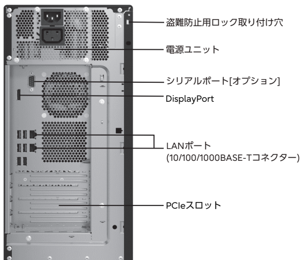
[タワーベースユニット (3.5インチ HDD/SSD×4/250W電源×1)]
