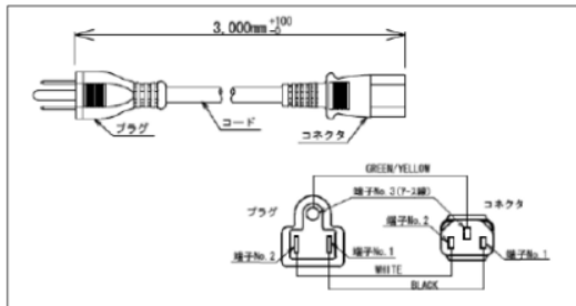
【NEMA 5-15】
