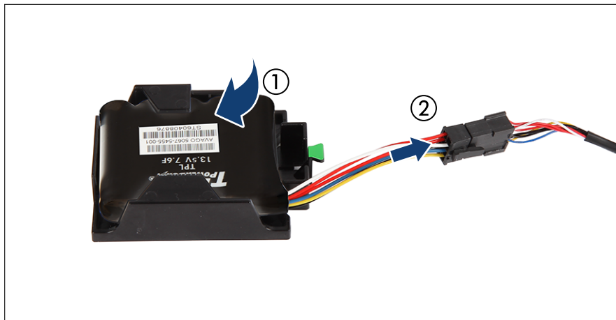
図 7: FBU ホルダーへの FBU の取り付け
