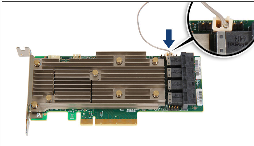
図 5: グローバルドライブアクティビティ LED ケーブルの接続
