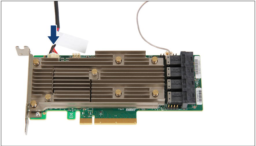
図 6: FBU アダプタケーブルの接続
