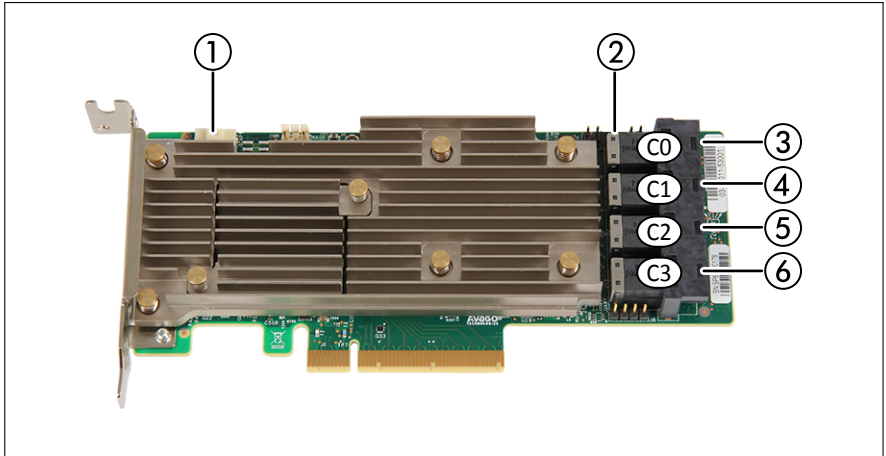
図 4: PRAID EP540i/EP580i ボードの配置
