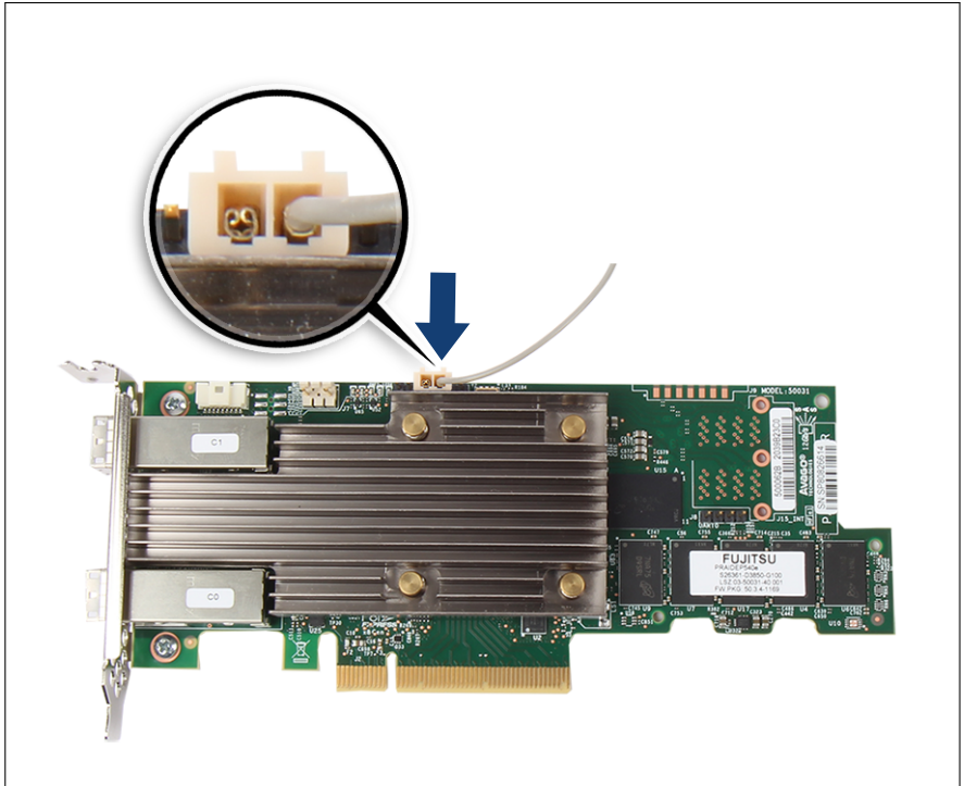
図 4: グローバルドライブアクティビティ LED ケーブルの接続
