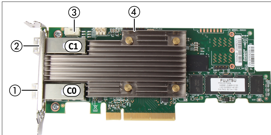
図 3: PRAID EP540e ボードの配置
