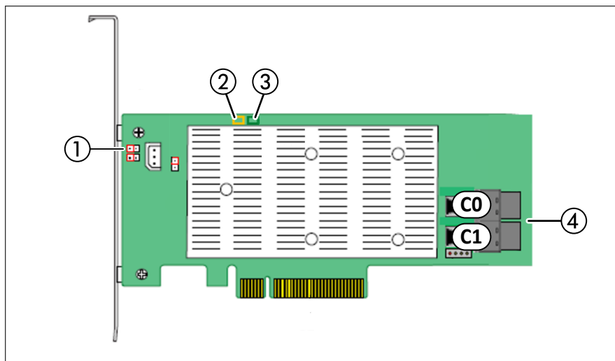
図 3: PRAID CP500i ボードの配置
