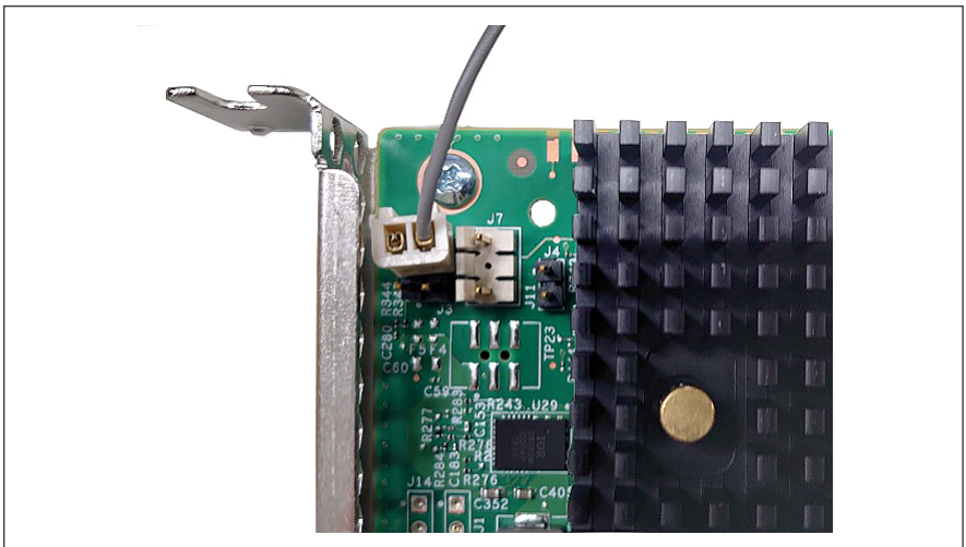
図 4: グローバルドライブアクティビティ LED ケーブルの接続
