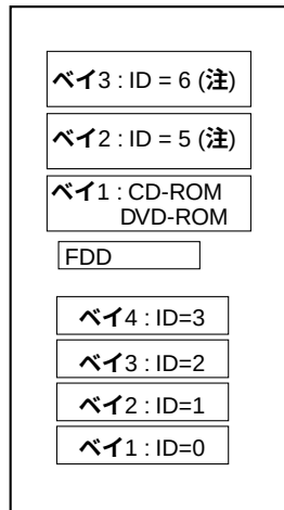
[ペDESTALタイプ時正面図]
