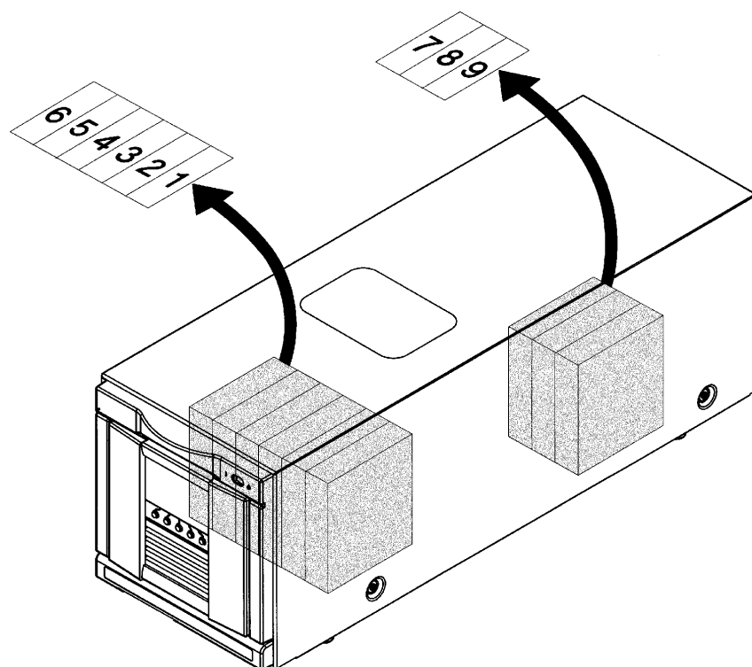
図 1.3 内部図（概要）
