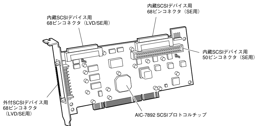
図1-1外観図
