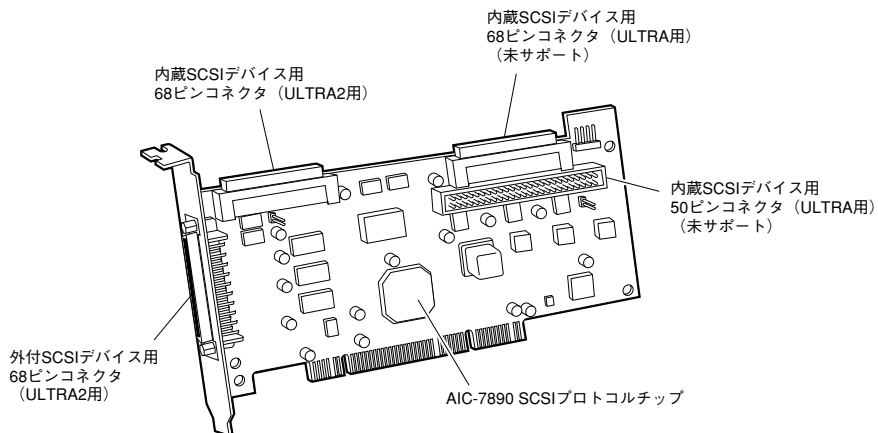
図1-1外観図
