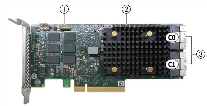
図 3: PRAID EP680i ボードの配置
