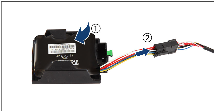
図 6: FBU ホルダーへの FBU の取り付け
