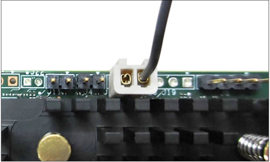
図 4: グローバルドライブアクティビティ LED ケーブルの接続
