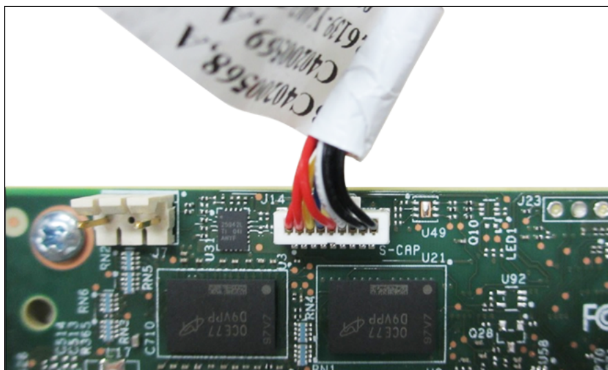
図 5: FBU アダプタケーブルの接続
