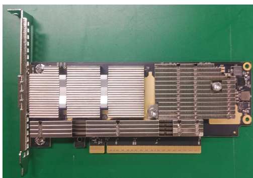
図 2: IB HCAカード(400Gbps) 部品面
