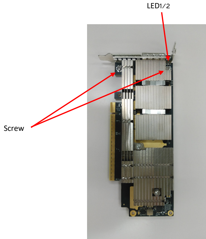
図 7: IB HCAカードの部品名称(カード共通)
