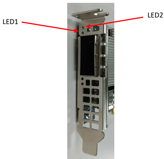
図 6: IB HCAカードのLED(カード共通)
