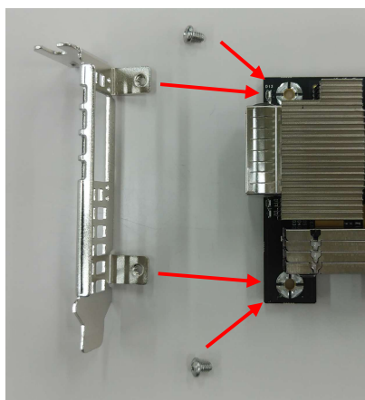
図 8: シングルポートカードの取付け方法
