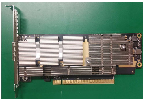
図 1: IB HCAカード(200Gbps) 部品面
