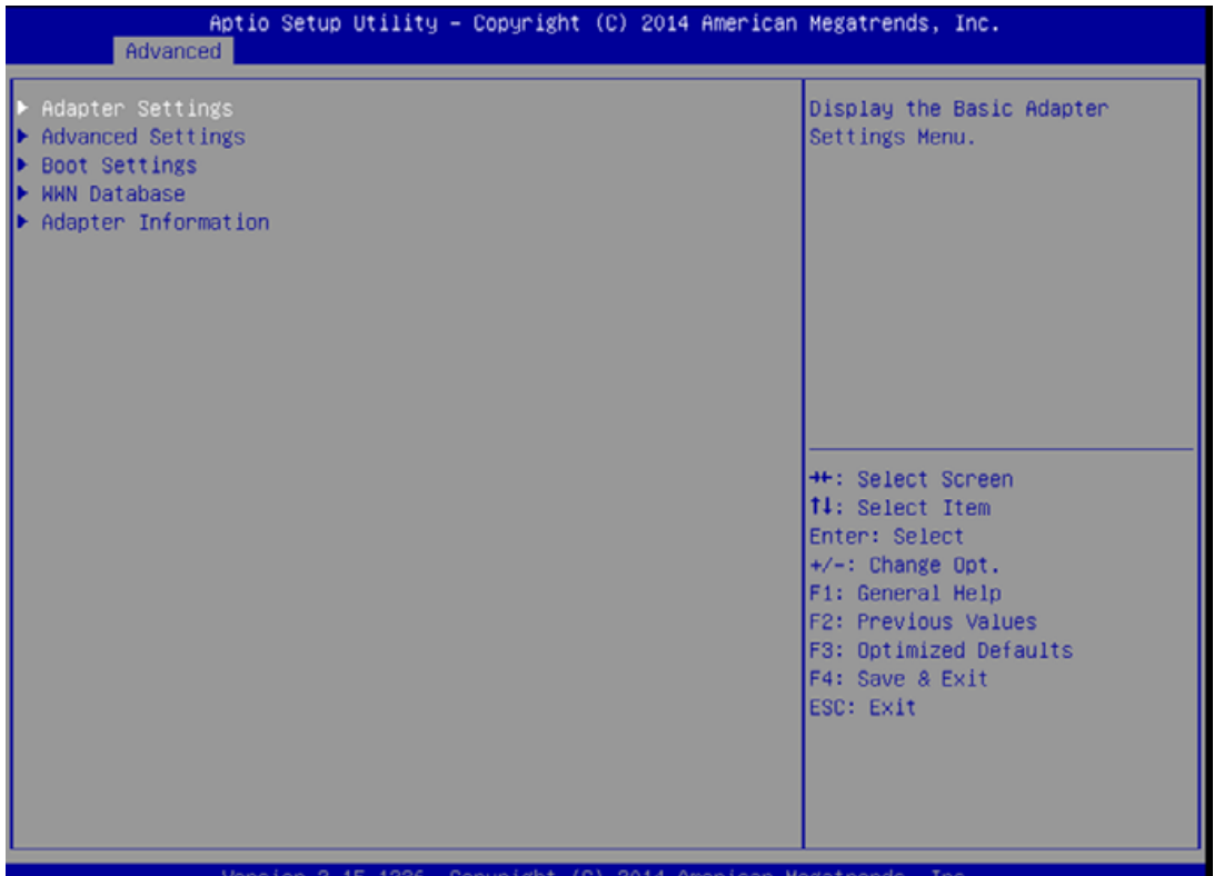
図 13 : HII Main メニュー
