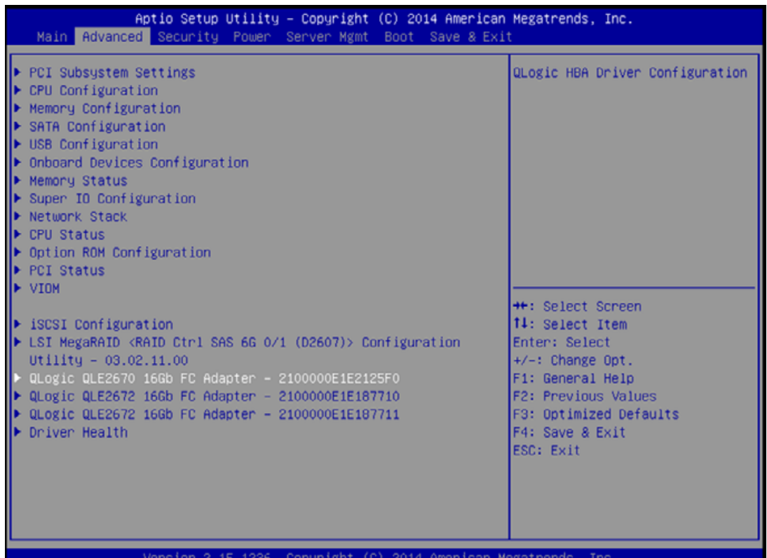
図 12: アダプタの選択
