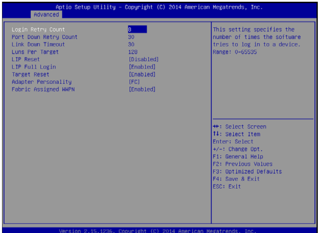
図 17: Advanced Setting ウィンドウ
