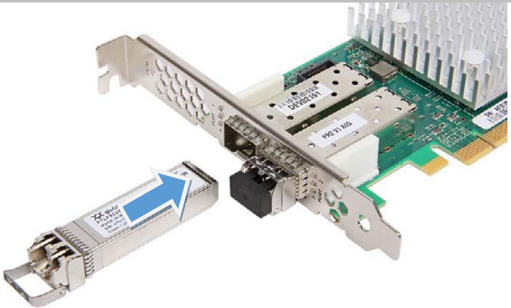
図 6：光トランシーバモジュールの取り外し
