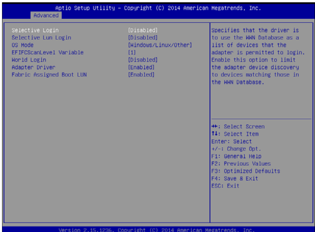
図 18: Boot Settings ウィンドウ
