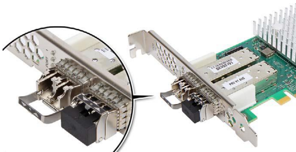
図 3：光トランシーバモジュールのロッキングハンドルのラッチ解除
