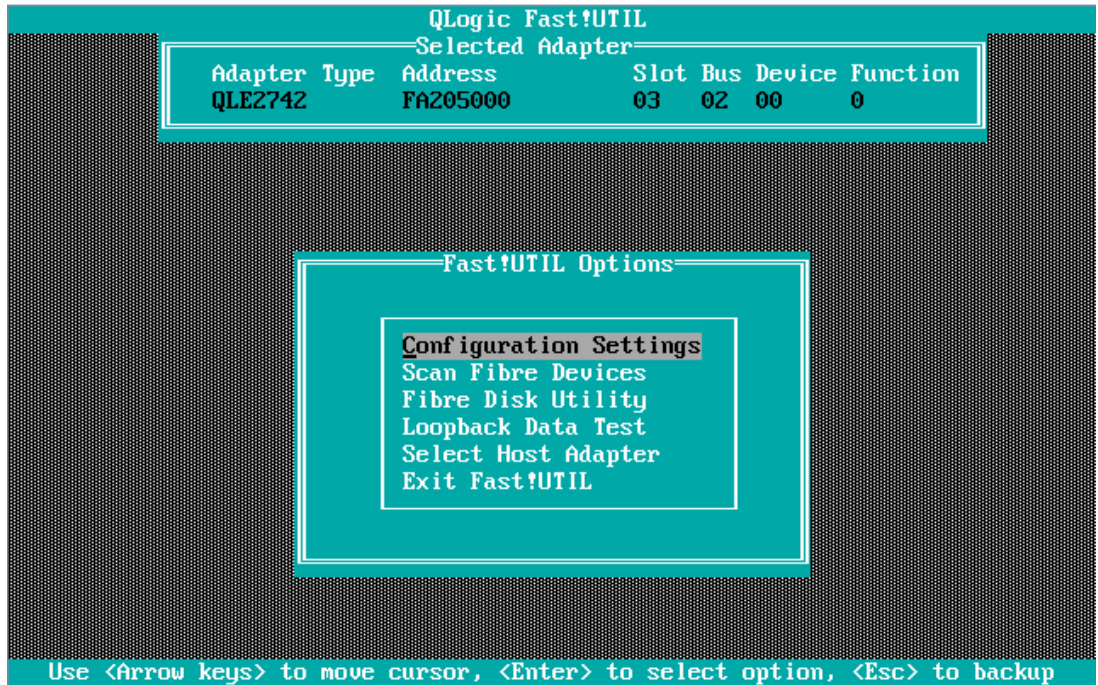
図 11: 「Fast!UTIL Option」メニュー
