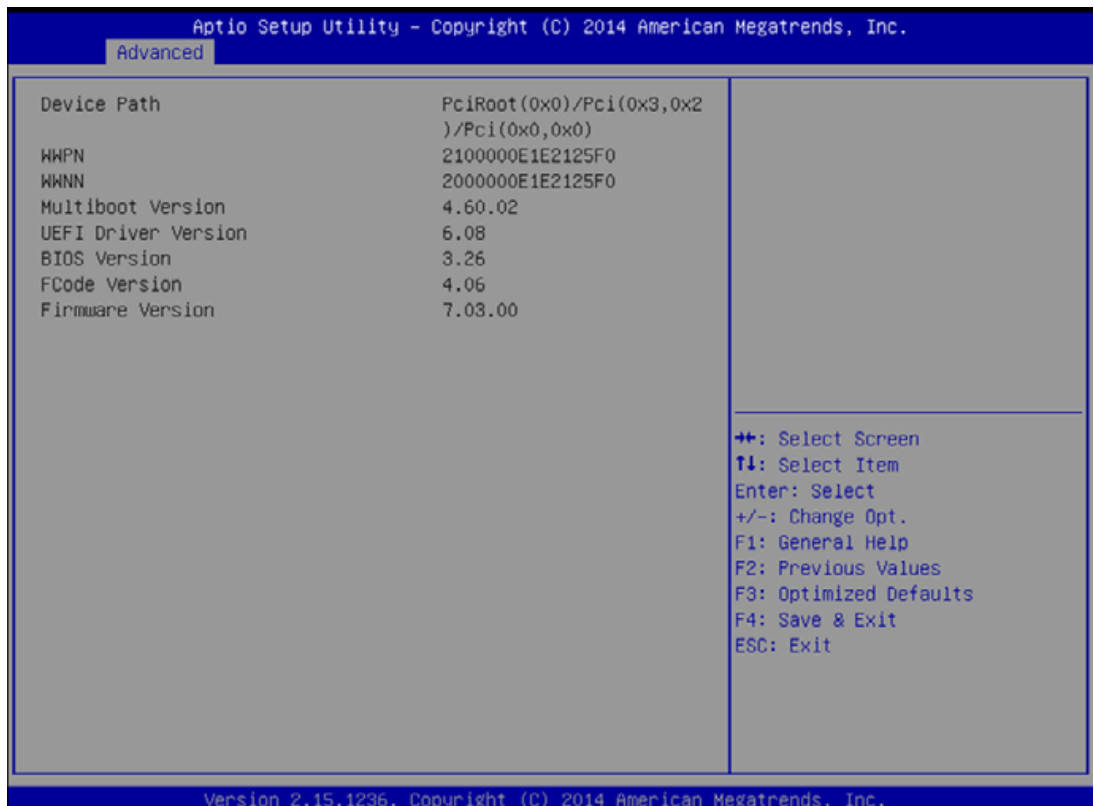
図 20 : Adapter Information ウィンドウ
