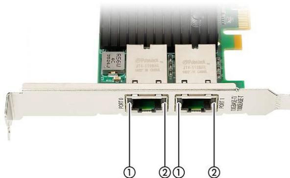
図 2-2 アダプタの LED 表示
