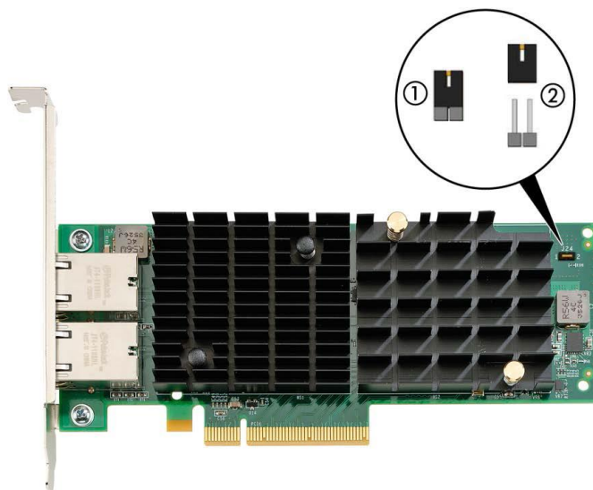
図 5-1 セキュアファームウェアジャンパーJ24
