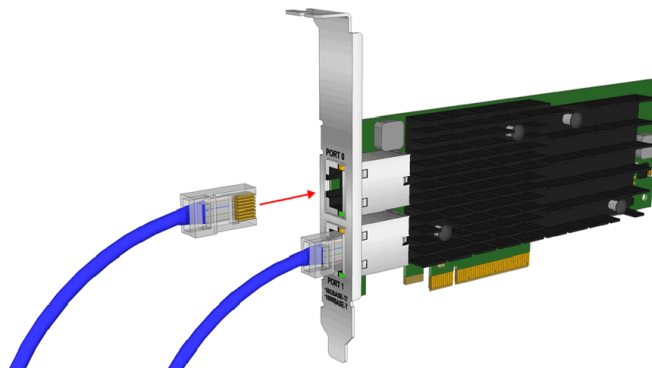
図 3-1 CAT ケーブルの接続
