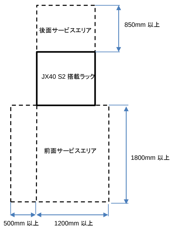
図 2.3 設置エリアとサービスエリア（JX40 S2 を搭載する場合- 2）
