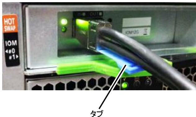
図 5.7 SAS ケーブル接続コネクタ
