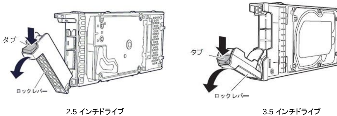
図 5.10 ロックの解除
