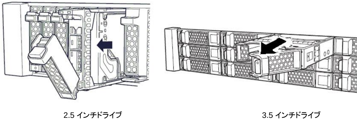
図 5.11 ドライブの引き出し
