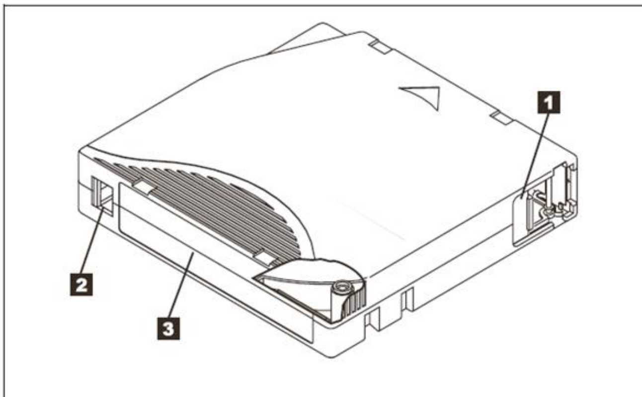
図 5: LTO Ultrium データ カートリッジ
