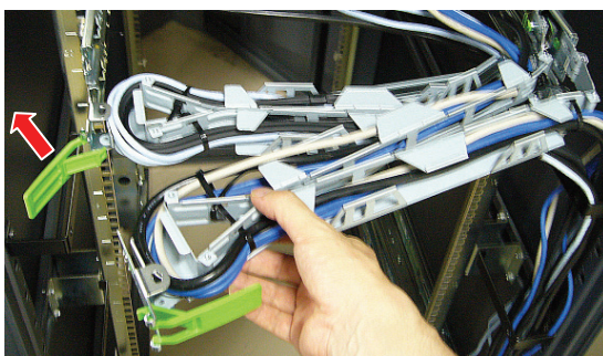
⑥ 下側：CMA ストップの解除
