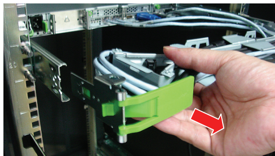
④ケーブルマネジメントアーム一式を後方に引き出す
