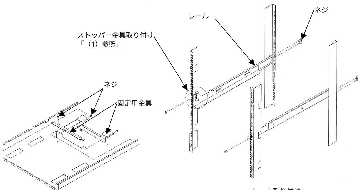
CRT 格納テーブル組み立て
