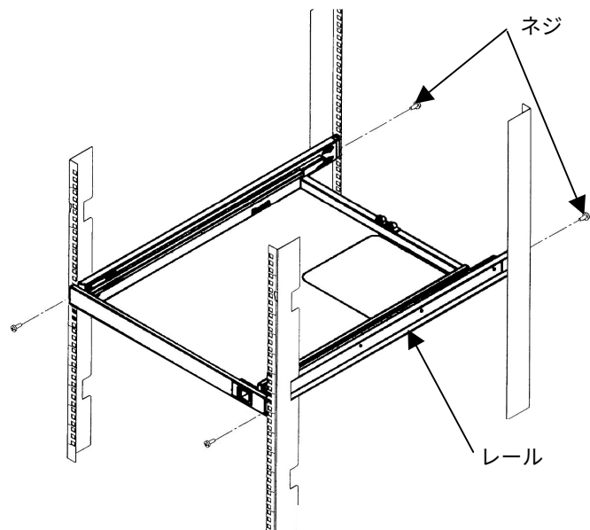
レール取り付け
