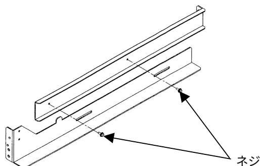
レール組み立て
