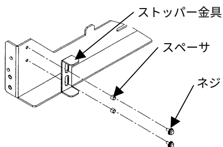
ストッパー金具取り付け詳細
