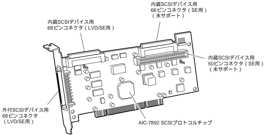
図1-1外観図
