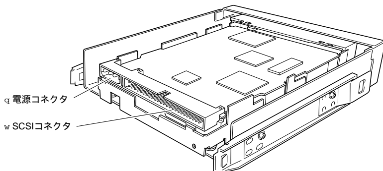
図1-2.ディスクユニットの後面
