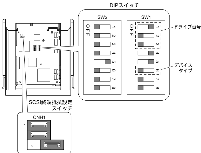
図2-1.各スイッチの初期状態
