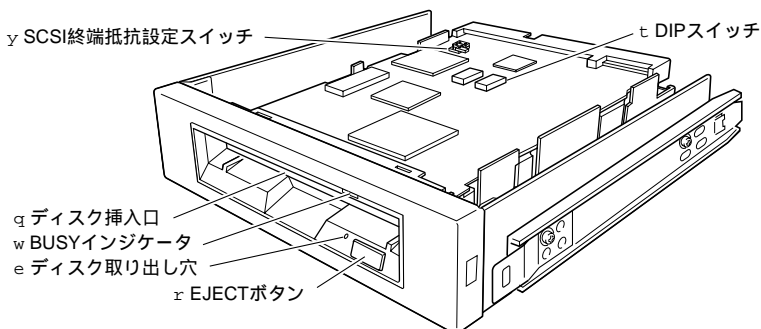
図1-1.ディスクユニットの前面および上面
