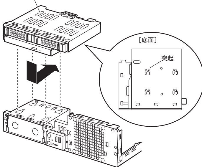
内蔵ハードディスクドライブベイ/内蔵CD-ROMドライブベイ
