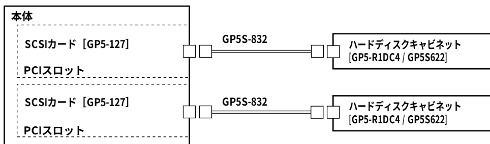
[SCSIカード(GP5-127)にハードディスクキャビネット(GP5-R1DC4 / GP5S622)を1台接続する場合]
