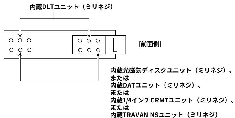
[ガイドレールのネジ穴位置]
