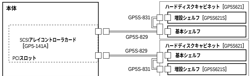
[SCSIアレイコントローラカード(GP5-141)にハードディスクキャビネット(GP5S621)を2台接続する場合]
