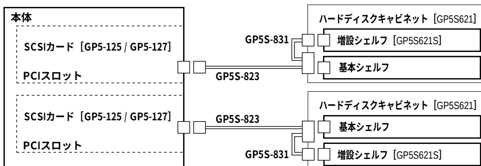
[SCSIカード(GP5-125)2枚にハードディスクキャビネット(GP5S621)を2台接続する場合]
