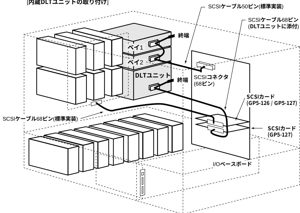
[内蔵DLTユニットの取り付け]
