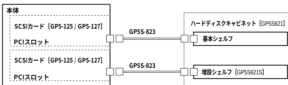
[SCSIカード(GP5-125)2枚にハードディスクキャビネット(GP5S621)を1台接続する場合]
