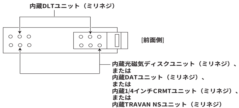
[ガイドレールのネジ穴位置]
