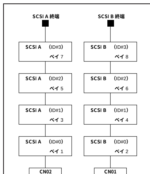
【装置正面より見た図】
