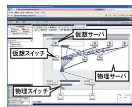
ネットワークマップの表示画面
