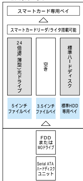
24倍速(薄型)光ドライブモデル
