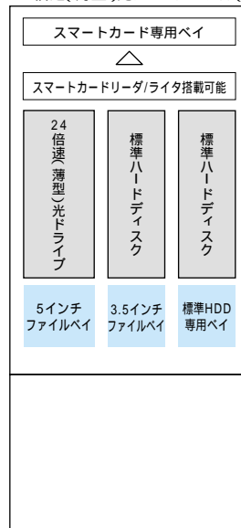
24倍速(薄型)光ドライブモデル(IDE-RAIDモデル)
