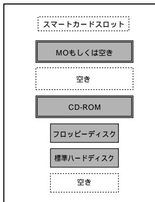
標準モデル
