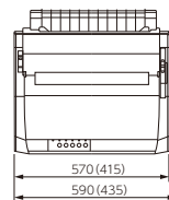
<上面図>
