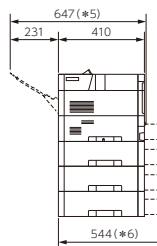
<側面図>
