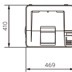
<上面図>
