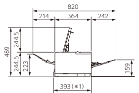
&lt;側面図&gt;
