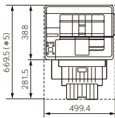
&lt;正面図&gt;
