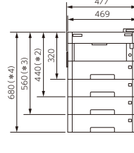
&lt;正面図&gt;
