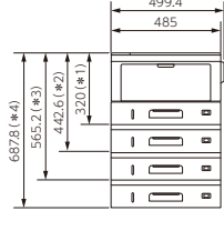
&lt;正面図&gt;
