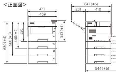
&lt;側面図&gt;
