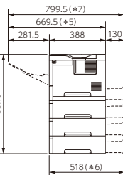
&lt;側面図&gt;
