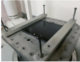
▼振動試験
