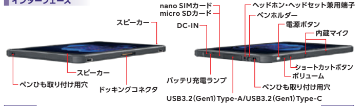
左側面
