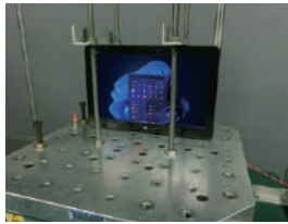
▼衝撃試験
