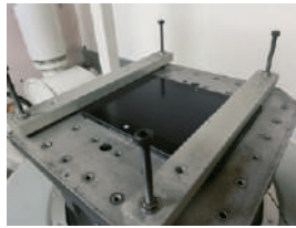
▼振動試験
