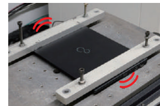
自動車や電車での移動・輸送時に加わる振動を想定し本体に振動をあたえ、動作のチェックを行います。
