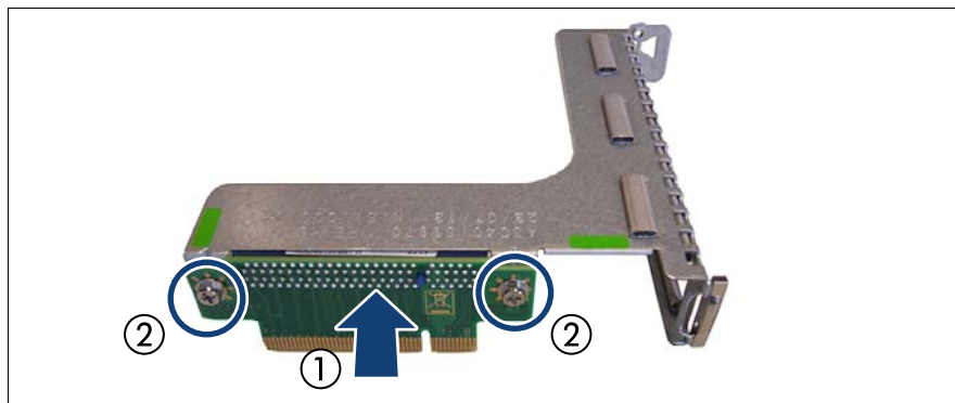
図 120: ライザーカードの取り付け - フルハイトライザーモジュールの例
