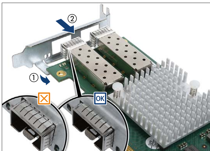
図 98: スロットブラケットの取り付け - D2755
