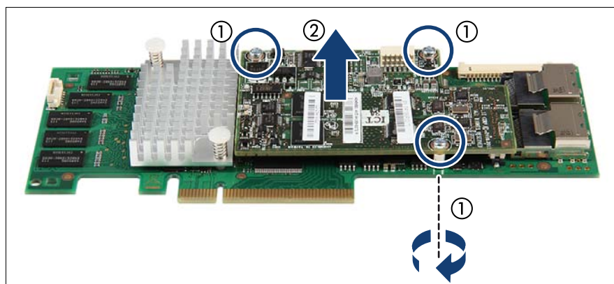
図 117: TFM の取り外し
