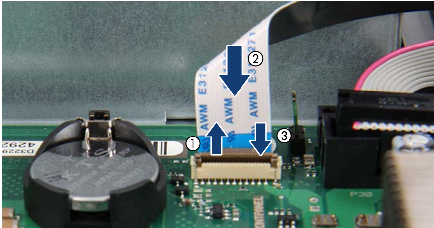
図 185: フロントパネルケーブルの接続 (B)
