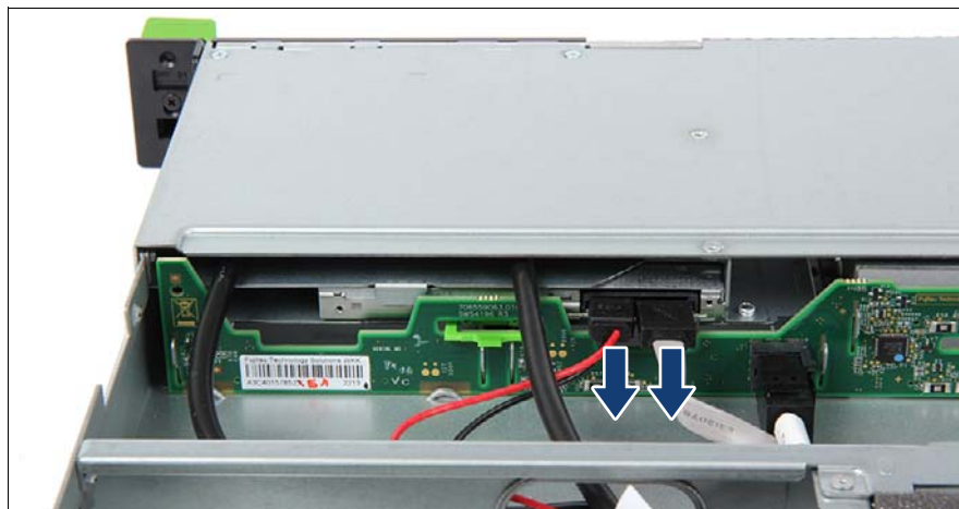
図 166: ODD からのケーブルの取り外し
