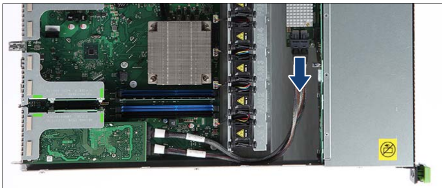
図 66: SAS ケーブルの取り外し
