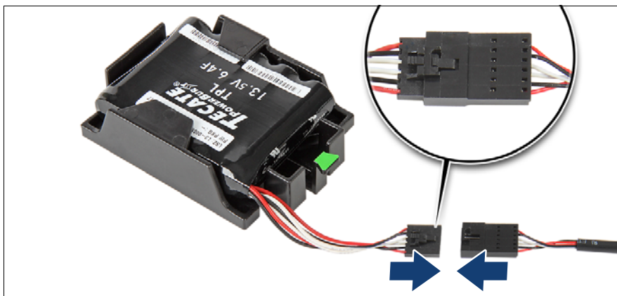
図 134: FBU への FBU アダプタケーブルの接続
