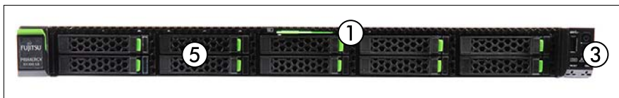
図 216: 前面 2.5 インチ HDD (最大 10 台の HDD)
