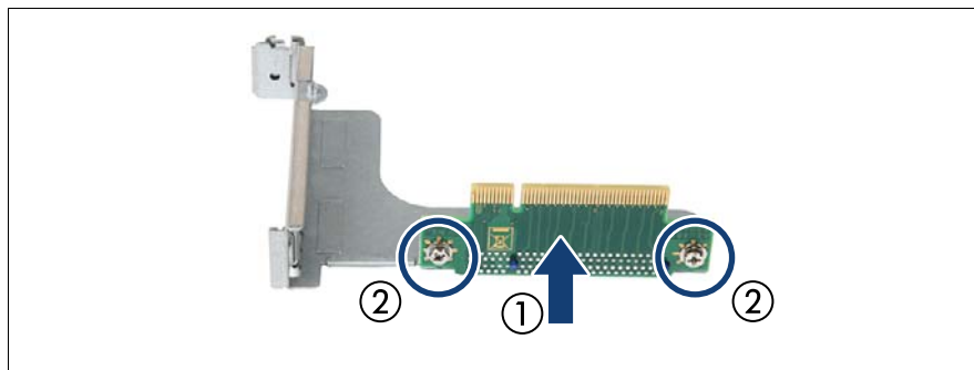
図 115: ライザーカードの取り付け - ライザーモジュールの例 1
