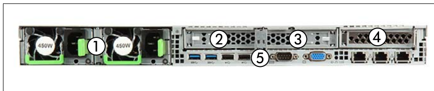
図 219: 背面（冗長電源ユニット）
