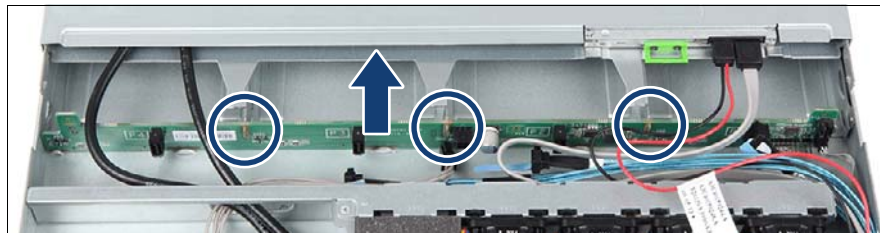
図 82: 3.5 インチ HDD バックプレーンの取り外し
