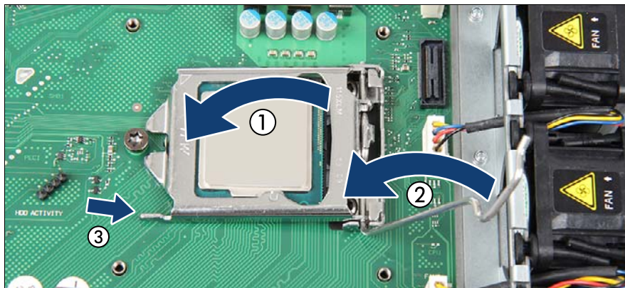
図 152: ホルダーを閉じる
