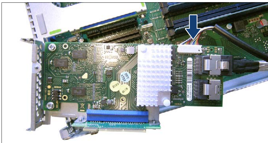
図 128: RAID コントローラへの BBU ケーブルの接続
