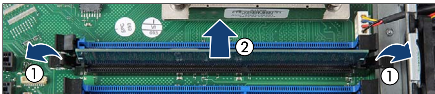
図 146: メモリモジュールの取り外し
