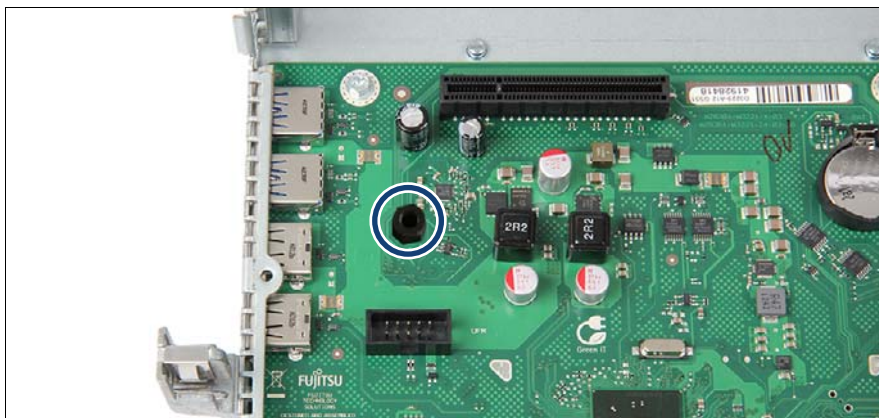
図 191: UFM スペーサーの取り外し
