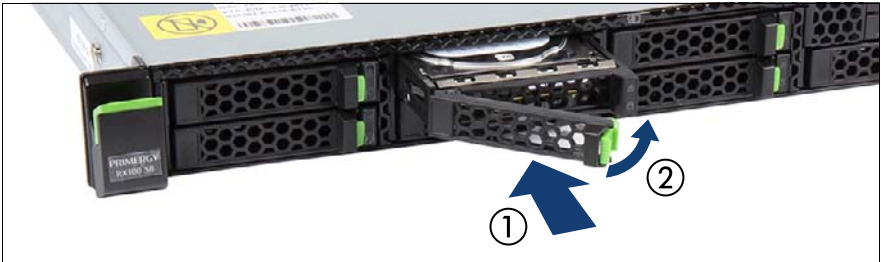
図 57: 2.5 インチ HDD/SSD モジュールの取り付け
