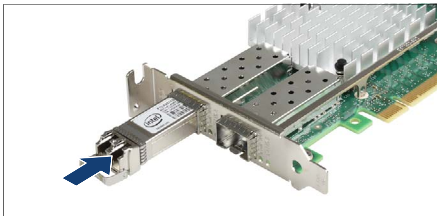
図 103: SFP+ トランシーバモジュールの挿入
