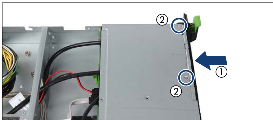
図 176: フロントパネルモジュールの取り付け
