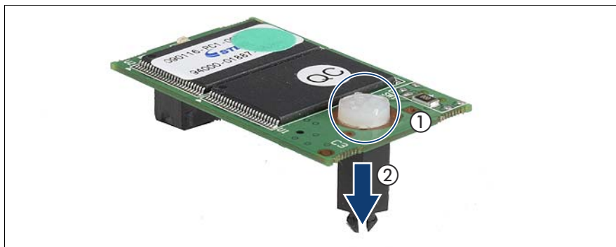
図 194: UFM スペーサーの取り外し
