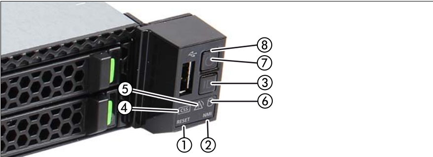
図 229: フロントパネル (HDDx10 モデル用 ) の表示ランプ
