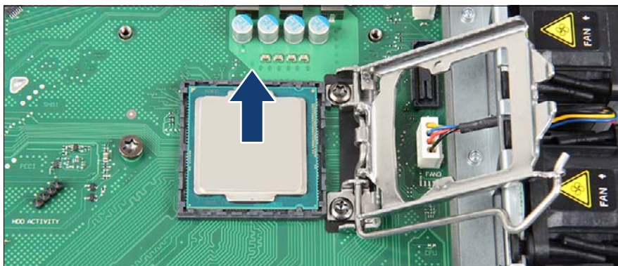
図 150: プロセッサの取り外し
