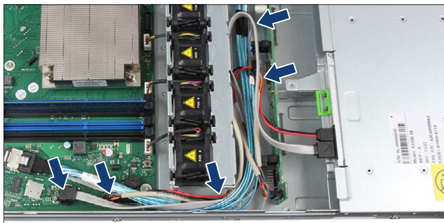
図 157: ODD ケーブルの配線 - 3.5 インチ HDD 構成の例
