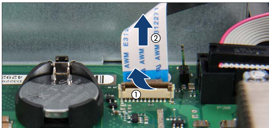
図 179: フロントパネルモジュールのケーブルの取り外し
