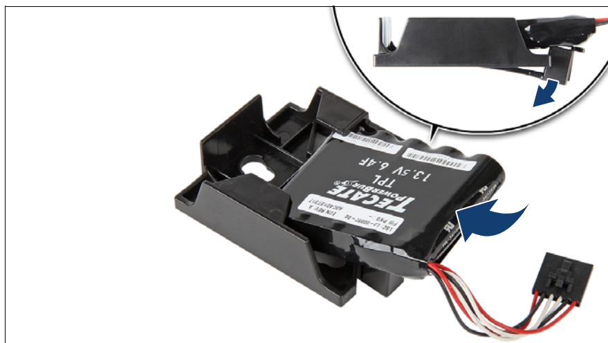
図 132: ホルダーへの FBU の取り付け (A)
