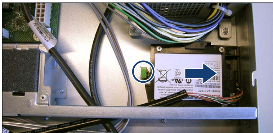
図 127: BBU とホルダーの取り付け
