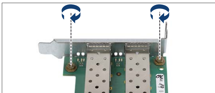
図 99: スロットブラケットの固定 - D2755
