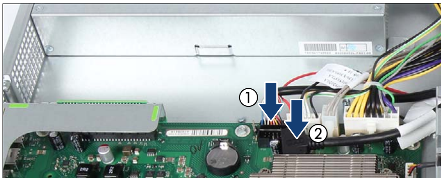
図 177: ケーブルの接続 (A)
