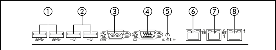
図 225: コネクタパネル
