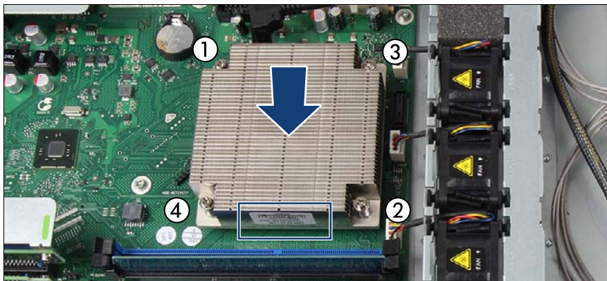
図 155: ヒートシンクの取り付け
