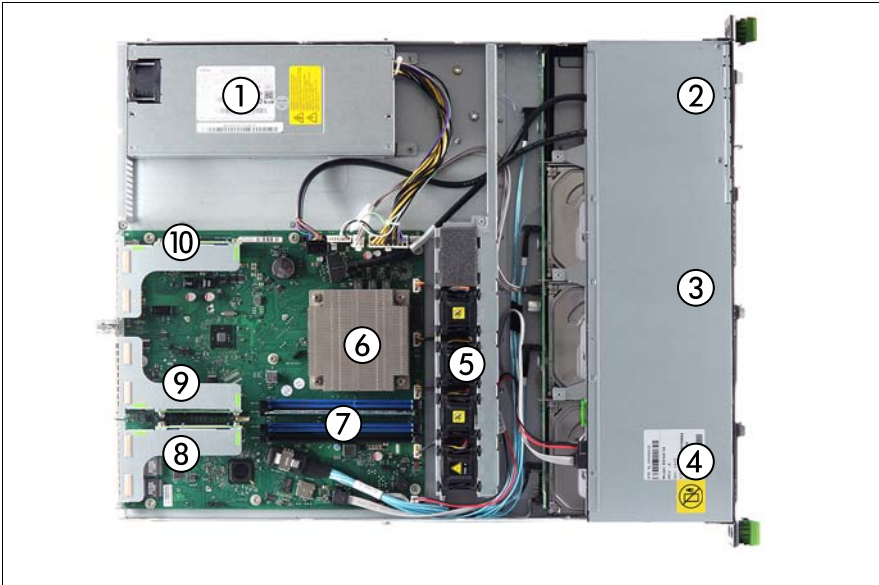
図 221: 内部（3.5 インチ HDD および標準電源の例）
