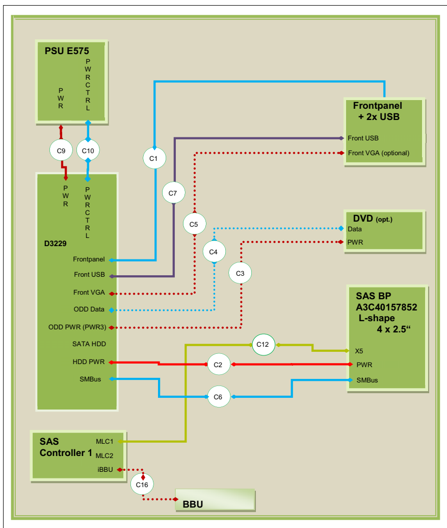
図 211: 配線 4x 2.5 インチ HDD、BBU、冗長電源
