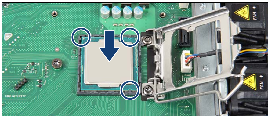
図 151: プロセッサを取り付ける
