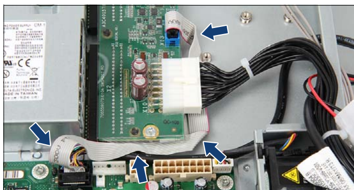
図 38: フラットケーブルの配線
