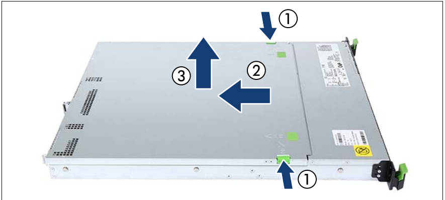
図 6: トップカバーの取り外し
