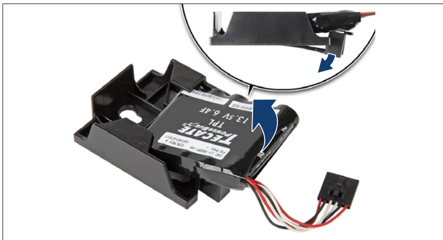
図 141: FBU をホルダーから取り外す
