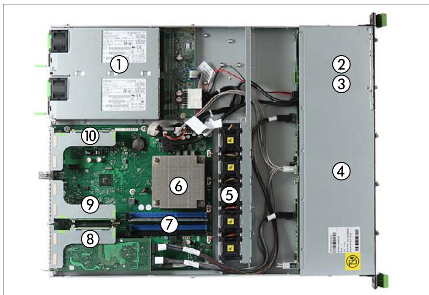
図 222: 内部（2.5 インチ HDD および冗長電源の例）
