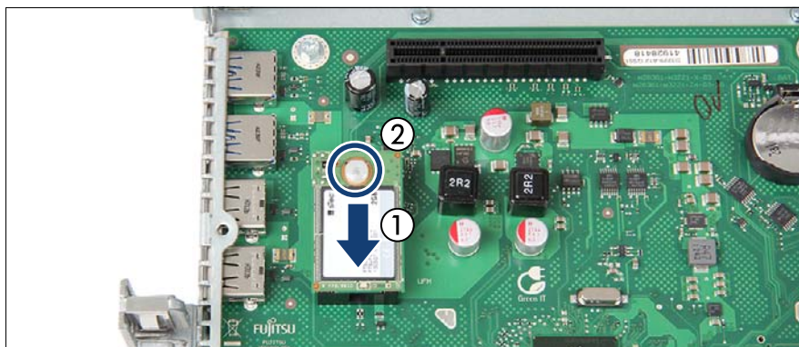
図 195: UFM の取り付け
