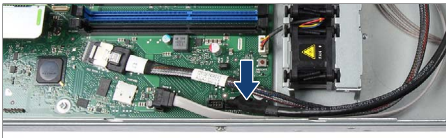
図 178: ケーブルの接続 (B)
