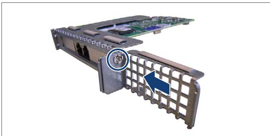
図 122: 拡張ブラケットの取り付け
