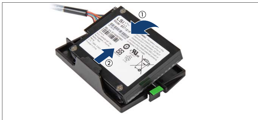
図 138: ホルダーからの BBU の取り外し
