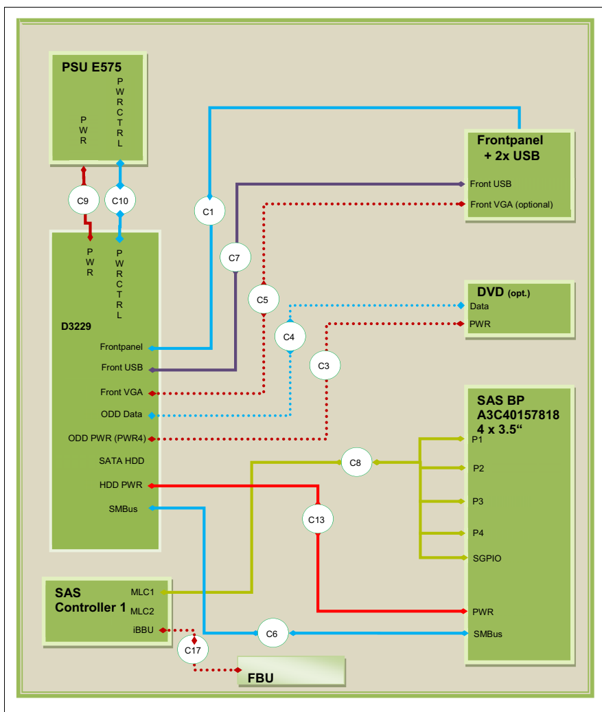
図 209: 配線 4x 3.5 インチ HDD、冗長電源
