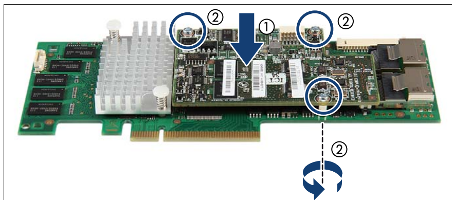
図 131: TFM の取り付け
