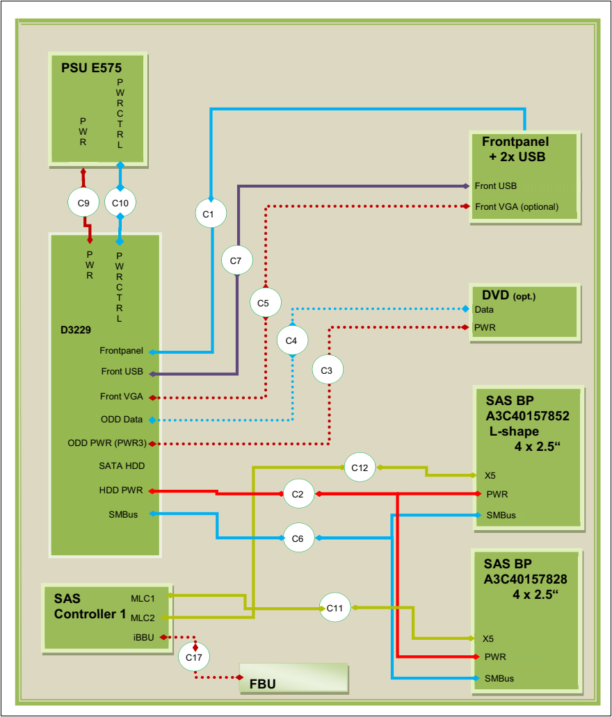
図 212: 配線 8x 2.5 インチ HDD、FBU、冗長電源
