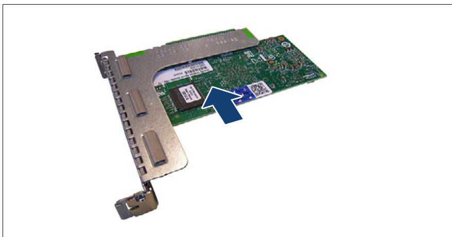
図 121: 拡張カードの取り付け - フルハイトライザーモジュールの例
