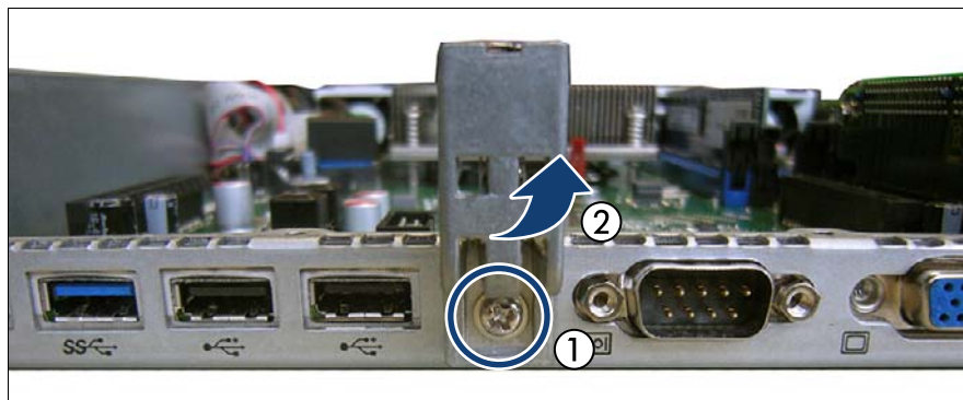
図 119: ライザーモジュールのサポートの取り外し
