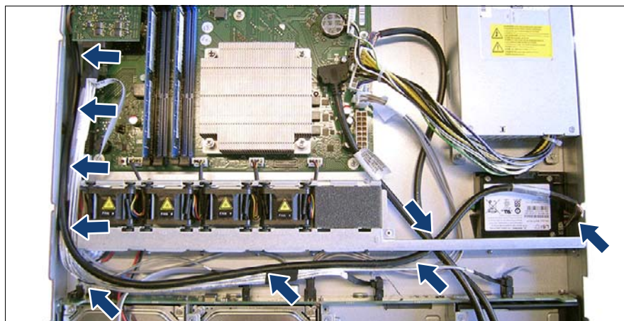
図 129: BBU ケーブルの配線
