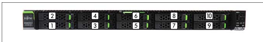
図 53: 最大 10 台の 2.5 インチ HDD/SSD の命名体系
