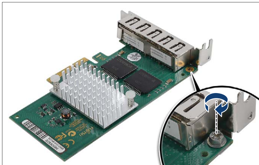
図 96: スロットブラケットの固定 - D2745
