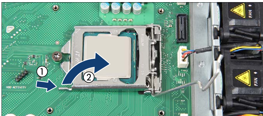
図 149: ホルダーを開く
