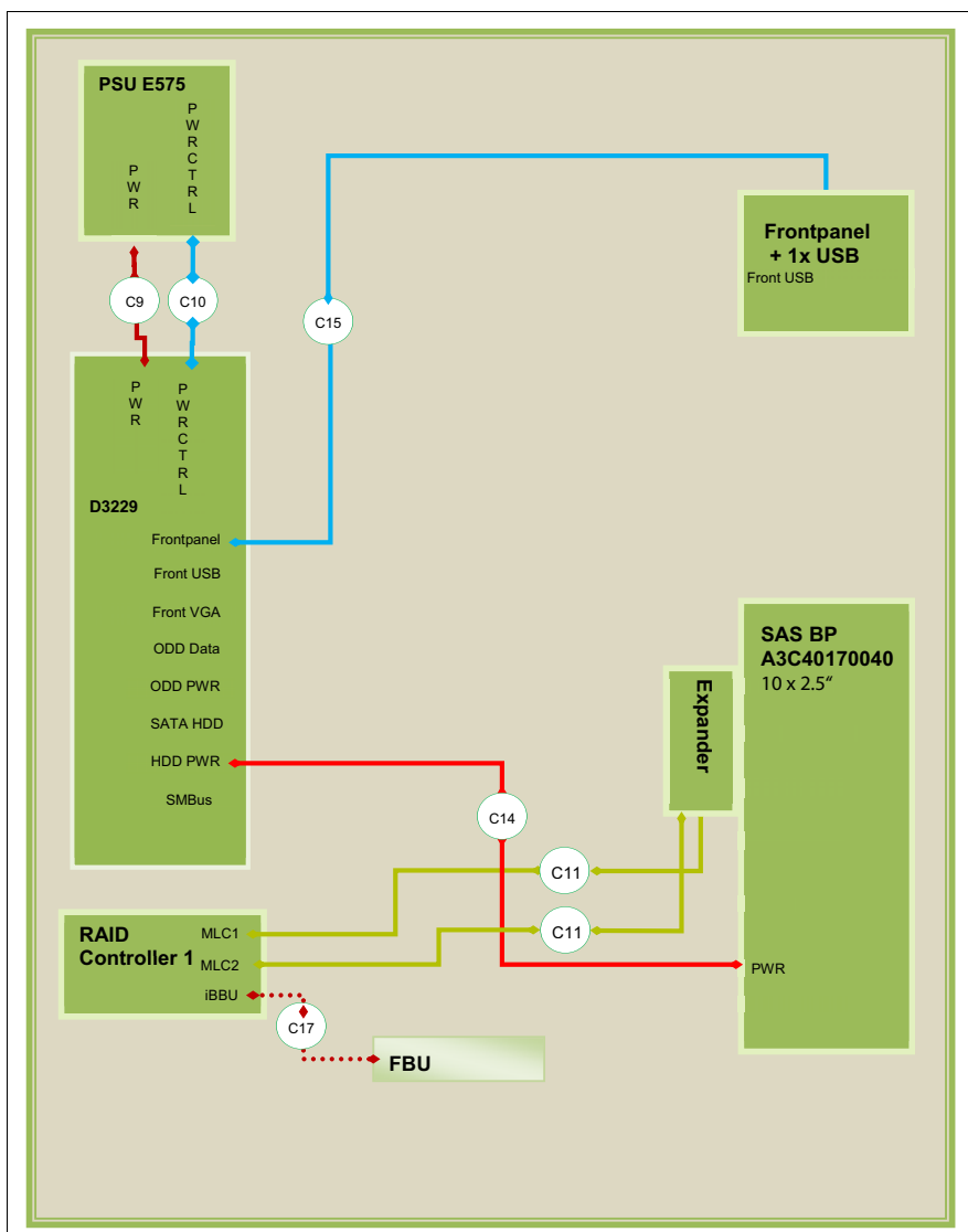
図 213: 配線 10x 2.5 インチ HDD、FBU、冗長電源
