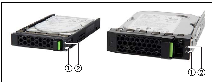
図 231: ホットプラグ HDD モジュールの表示ランプ
