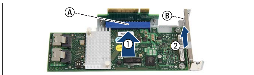
図 111: 拡張カードの取り付け - ライザーモジュールの例 1
