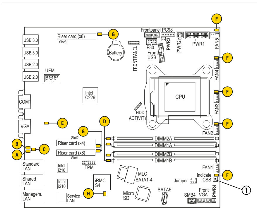
図 224: オンボード表示ランプと CSS ボタン
