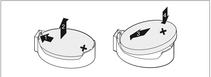
図 186: CMOS バッテリーの交換
