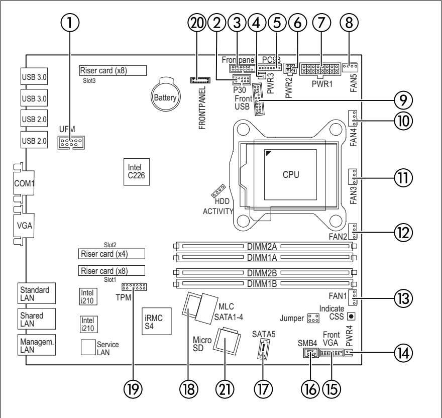
図 223: システムボード D3229 の内部コネクタ
