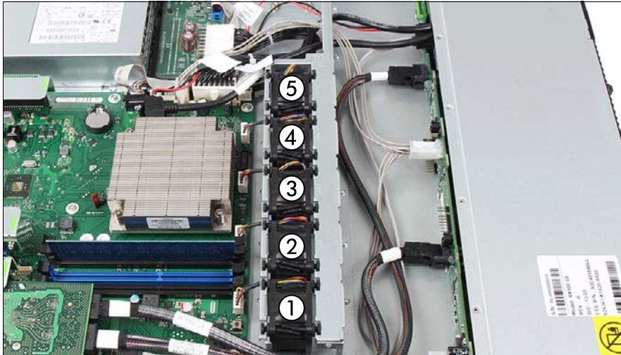
図 85: ファンモジュールの番号付け
