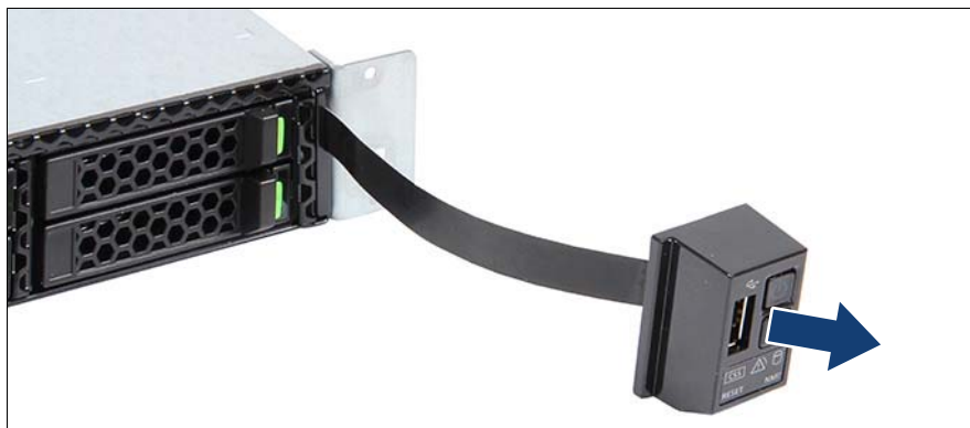
図 182: フロントパネル（HDDx10 モデル用）の取り外し（B）
