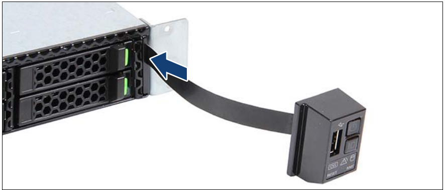
図 183: フロントパネルの取り付け (A)
