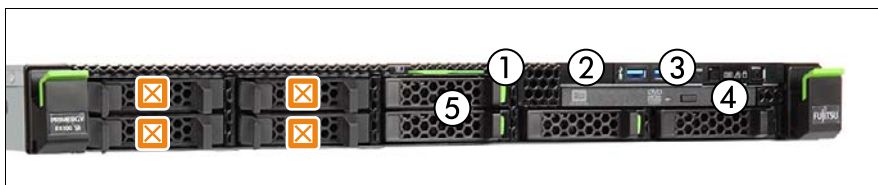
図 214: 前面 2.5 インチ HDD (最大 4 台の HDD)
