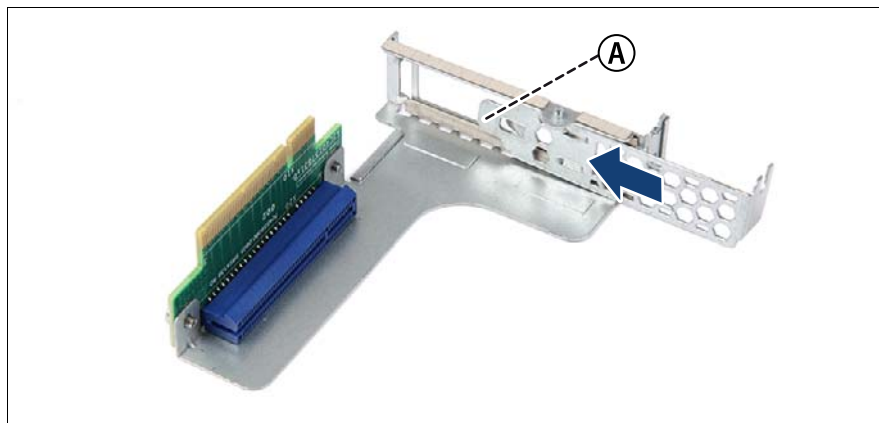
図 113: スロットカバーの取り付け - ライザーモジュールの例 1
