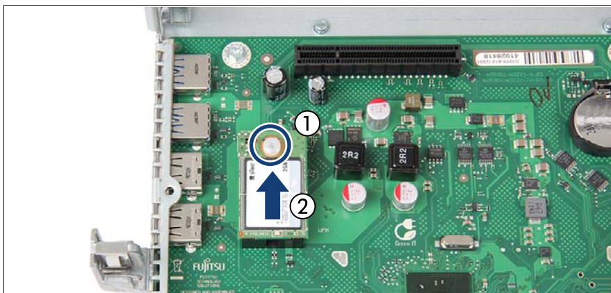
図 190: UFM の取り外し
