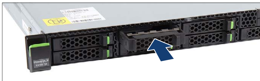
図 58: 2.5 インチ ダミーモジュールの取り付け
