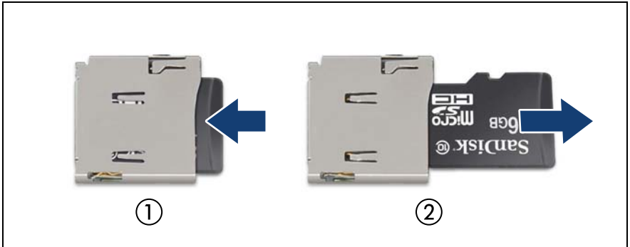
図 205: iRMC microSD カードの取り外し
