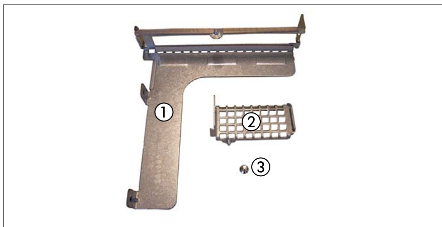
図 118: アップグレードキット
