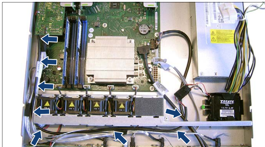
図 136: FBU ケーブルの配線
