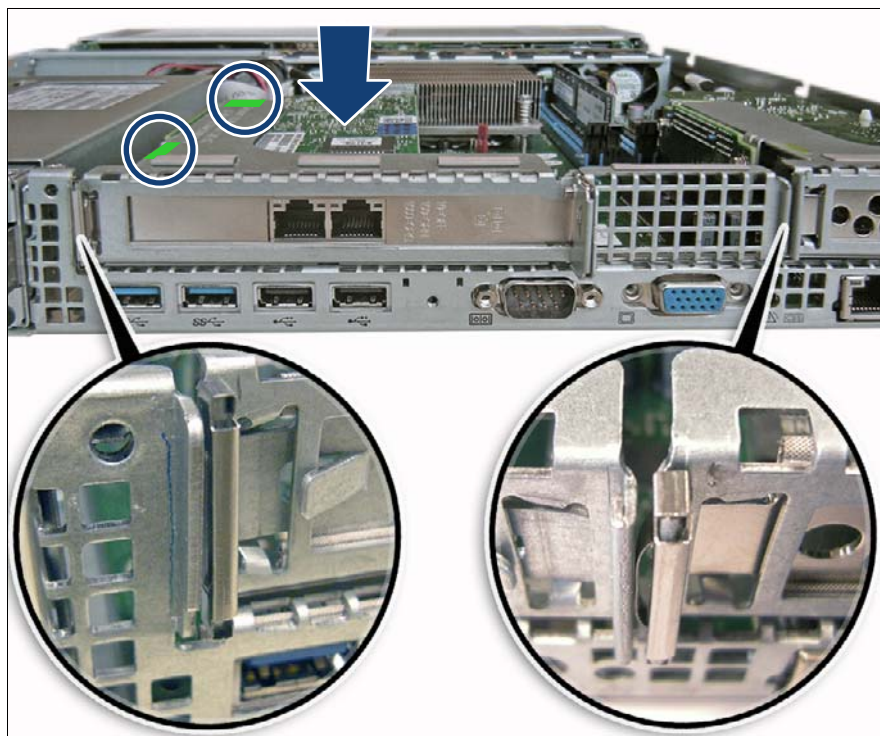
図 123: フルハイトライザーモジュールの取り付け
