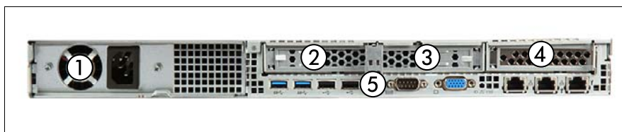
図 218: 背面（標準電源）
