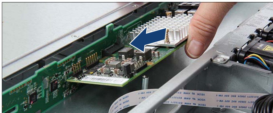
図 71: SAS エキスパンダボードの取り付け（A）
