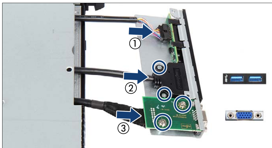
図 175: フロントパネルモジュールへのケーブルの接続
