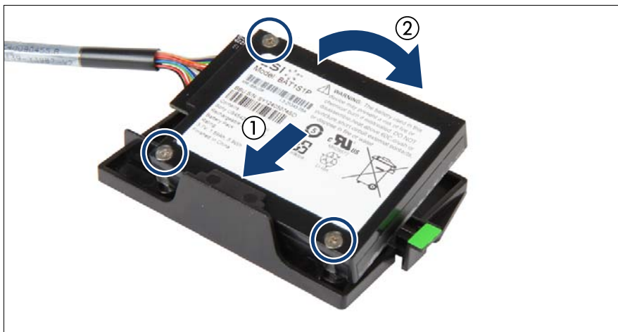
図 125: BBUホルダーへの取り付け
