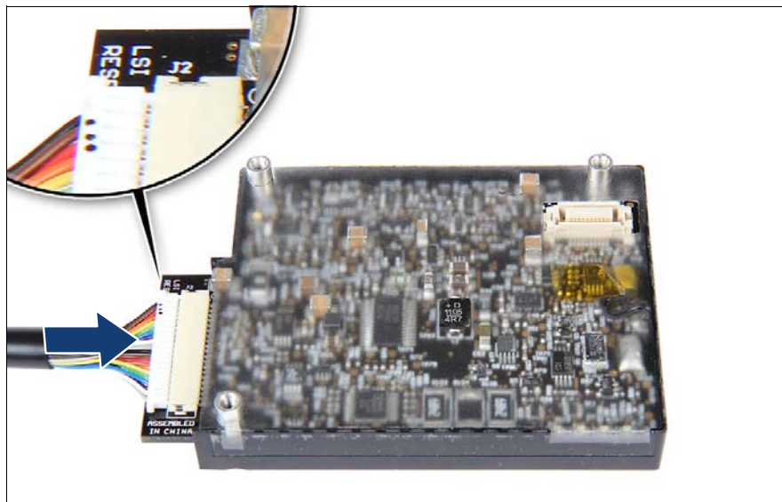
図 124: BBU ケーブルの接続
