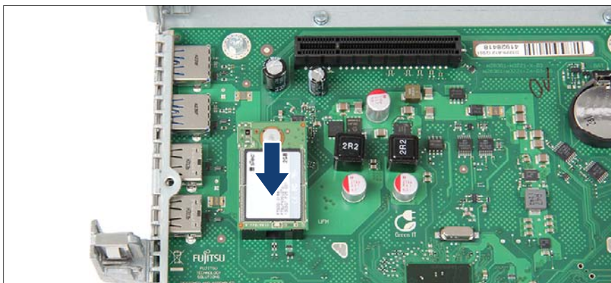
図 189: UFM の取り付け
