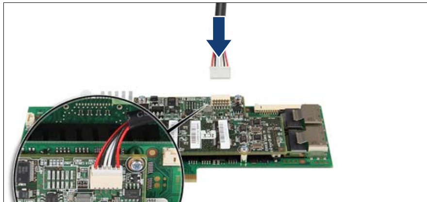
図 135: TFM への FBU アダプタケーブルの接続
