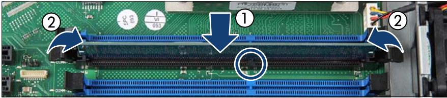
図 145: メモリモジュールを取り付ける
