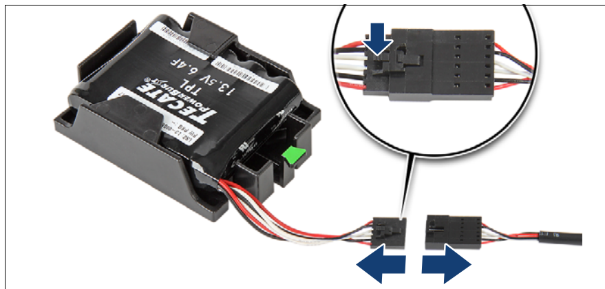
図 140: FBU からの FBU ケーブルの取り外し
