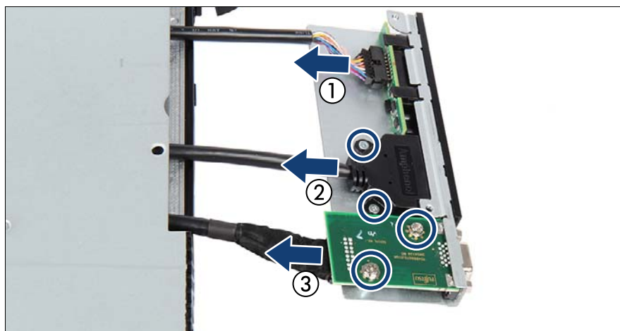
図 173: フロントパネルモジュールからのケーブルの取り外し
