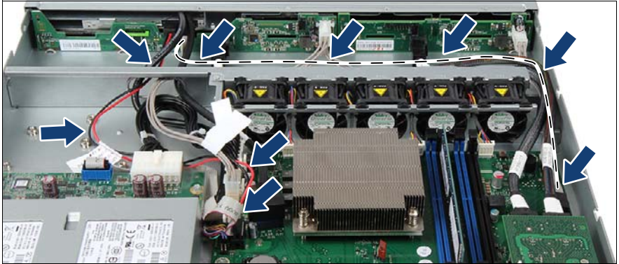
図 159: ODD ケーブルの配線 - 2.5 インチ HDD 構成の例
