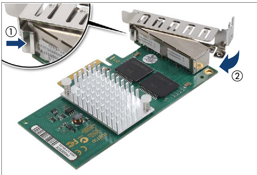
図 95: スロットブラケットの取り付け - D2745
