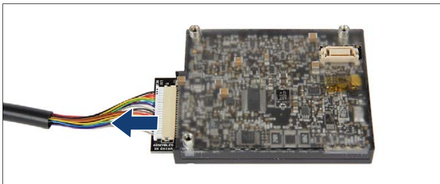
図 139: BBU からの BBU ケーブルの取り外し
