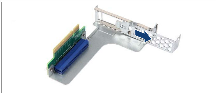
図 110: スロットカバーの取り外し - ライザーモジュールの例 1
