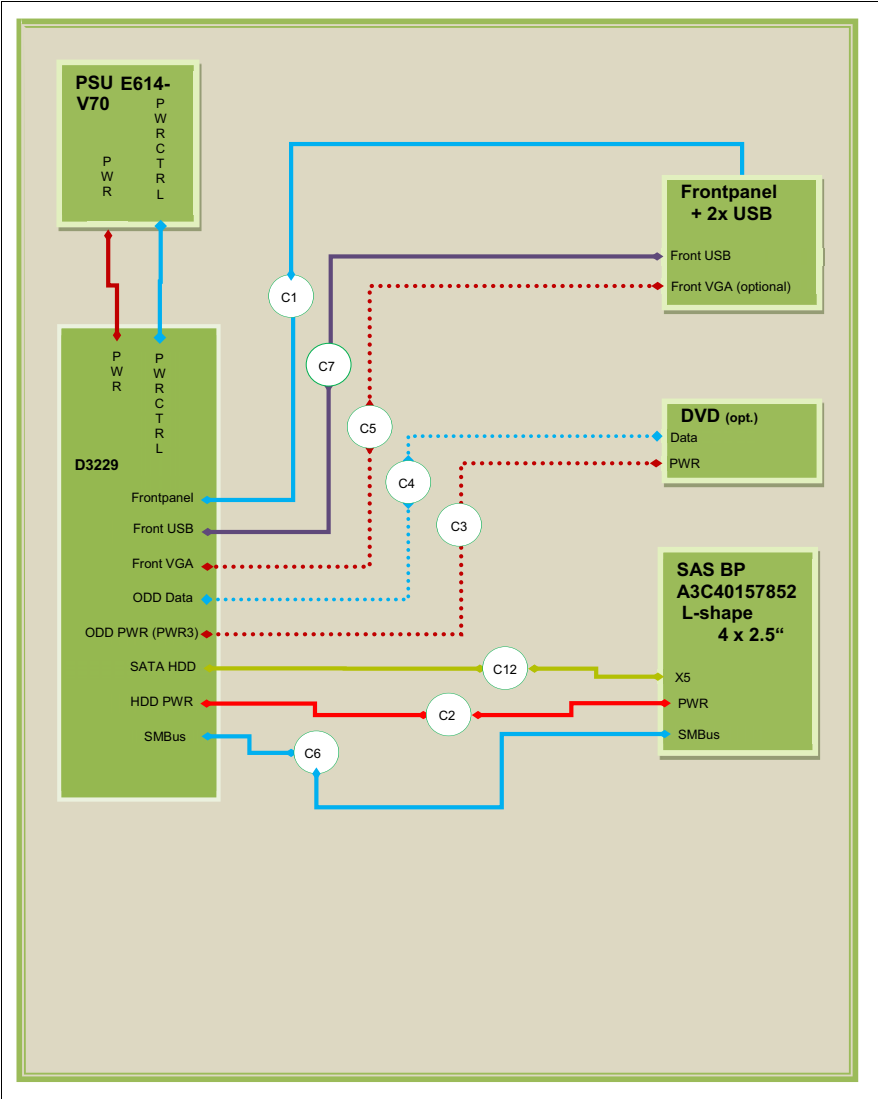
図 210: 配線 4x 2.5 インチ HDD、標準電源
