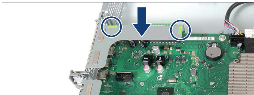
図 18: ライザーモジュール 3 の取り付け
