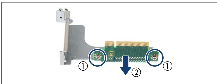
図 114: ライザーカードの取り外し - ライザーモジュールの例 1
