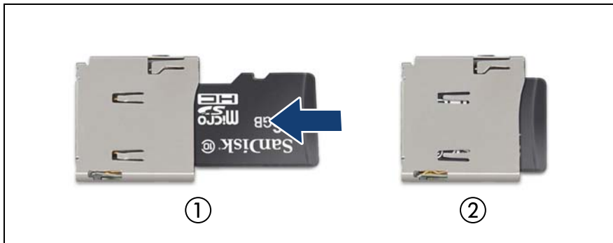
図 204: iRMC microSD カードの取り付け
