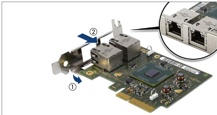
図 92: スロットブラケットの取り付け - D2735
