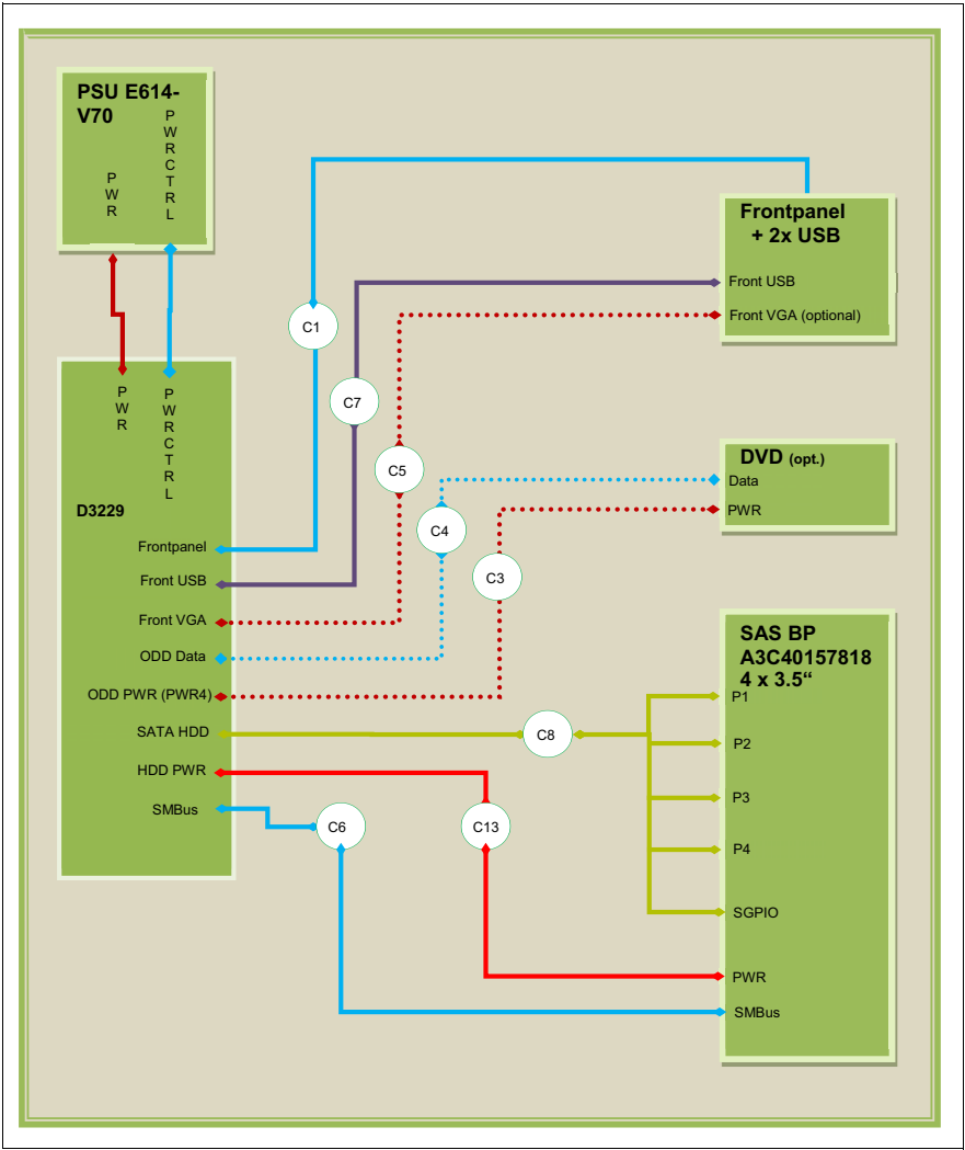
図 208: 配線 4x 3.5 インチ HDD、標準電源
