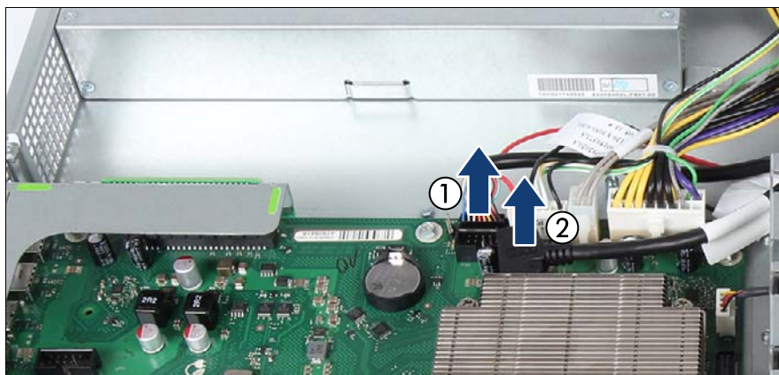
図 170: ケーブルの取り外し (A)
