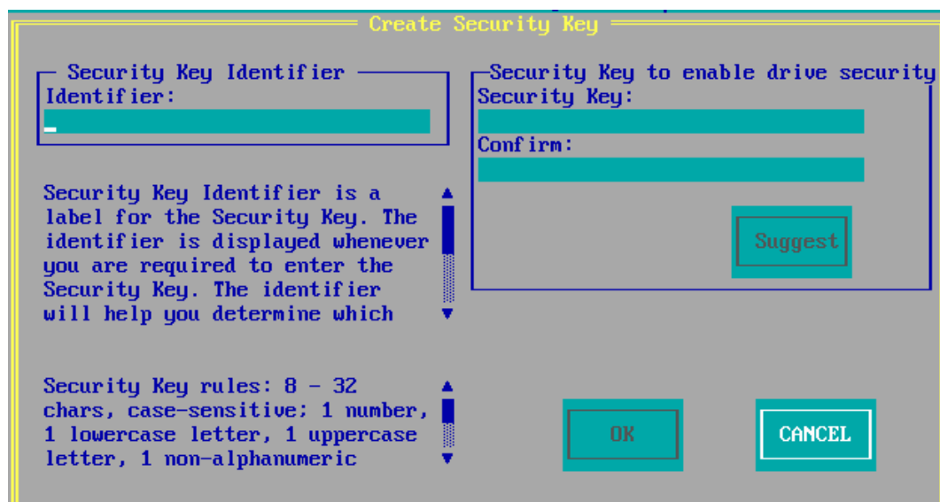
図 13 Enable Security (24.7.0-0061)
