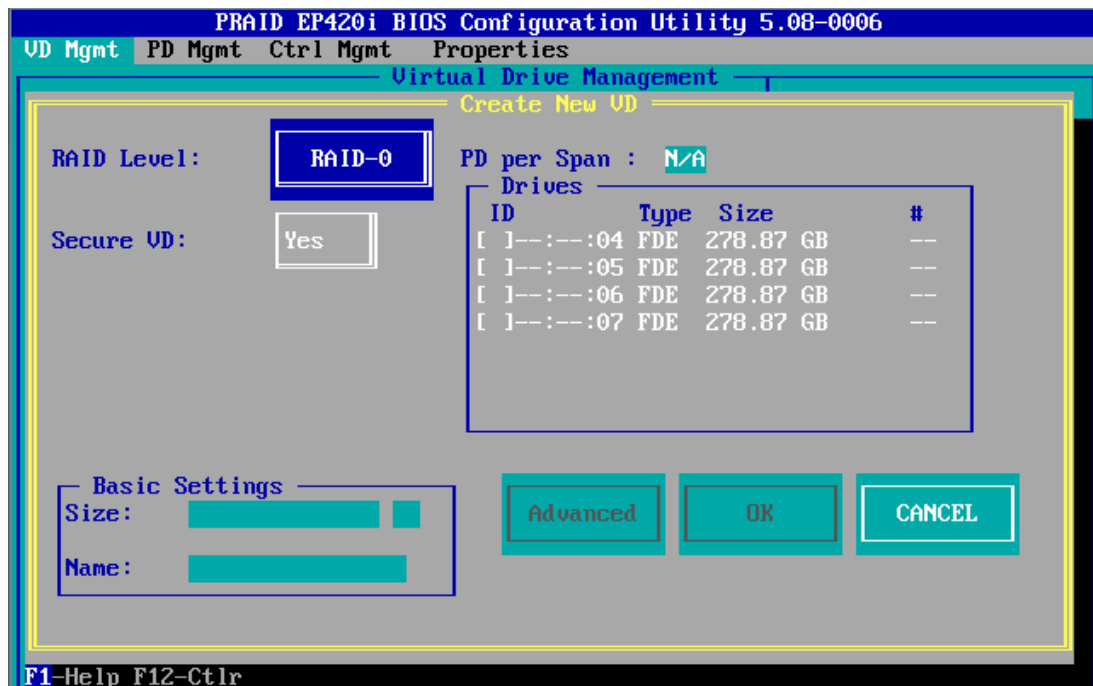
図 12 Create VD (24.7.0-0061)
