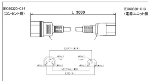
【IEC60320-C13 - IEC60320-C14】
