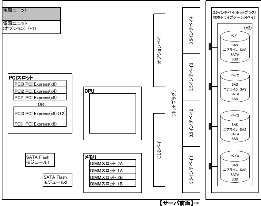
【サーバ前面】→
