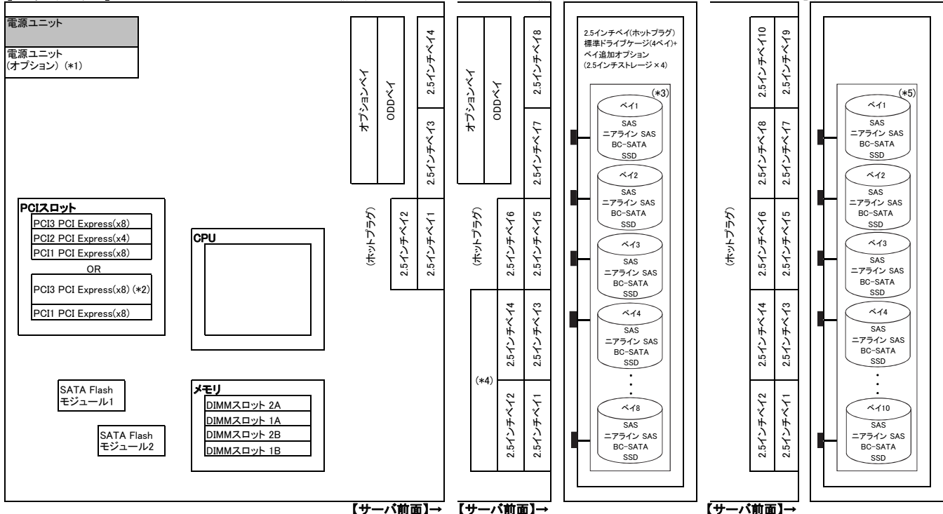
【サーバ前面】→
