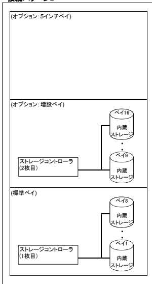
・接続パターン2
