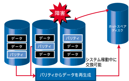
アレイ構成の一例 RAID5)
